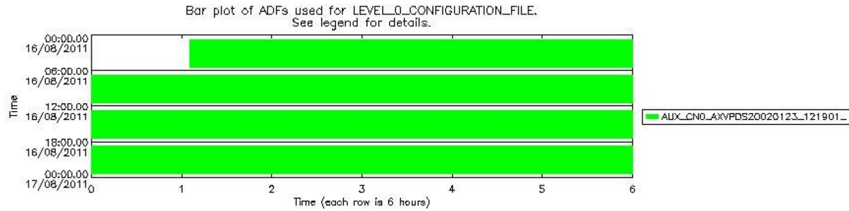
mipas_daily_report_level0_KSPT_L0_4504_N_20110816_12.PNG
