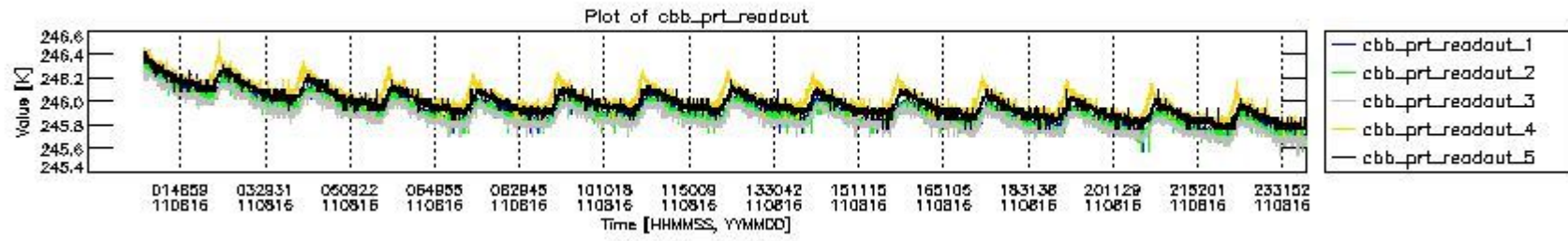
mipas_daily_report_level0_KSPT_L0_4504_N_20110816_9.PNG
