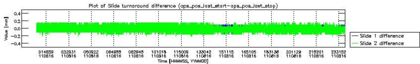
mipas_daily_report_level0_KSPT_L0_4504_N_20110816_5.PNG
