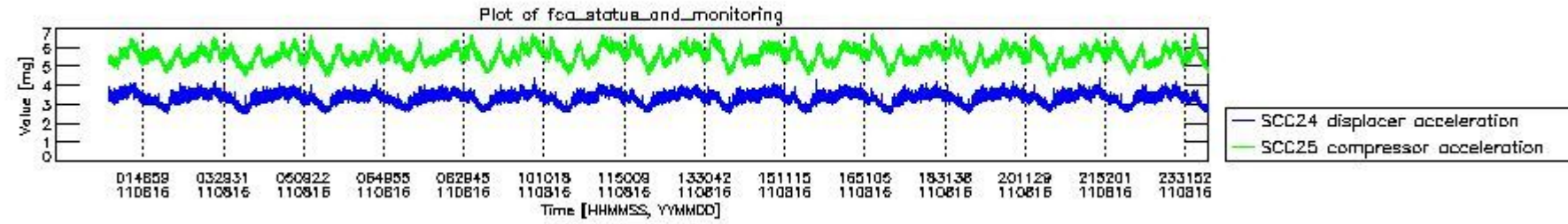
mipas_daily_report_level0_KSPT_L0_4504_N_20110816_10.PNG
