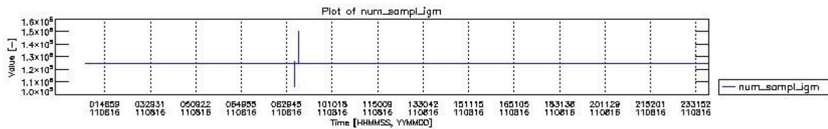
mipas_daily_report_level0_KSPT_L0_4504_N_20110816_0.PNG
