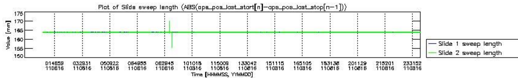
mipas_daily_report_level0_KSPT_L0_4504_N_20110816_7.PNG
