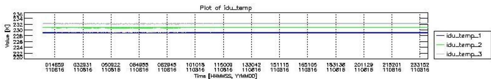
mipas_daily_report_level0_KSPT_L0_4504_N_20110816_2.PNG
