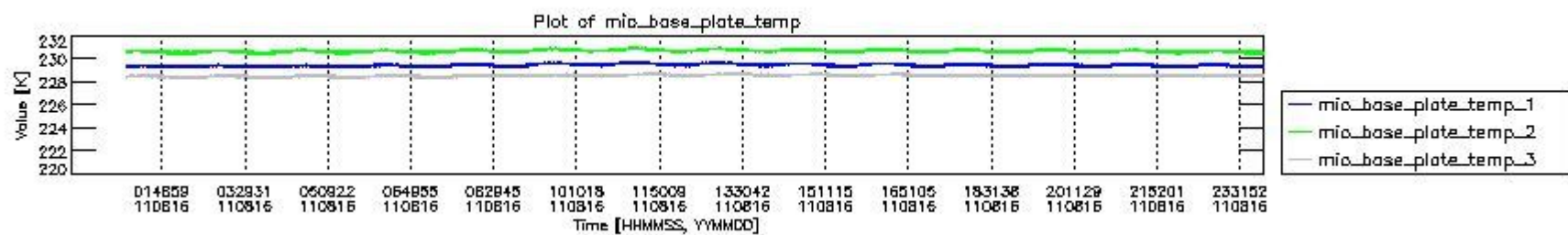
mipas_daily_report_level0_KSPT_L0_4504_N_20110816_1.PNG
