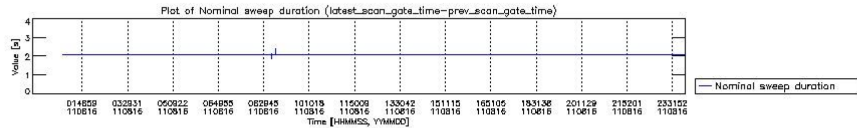
mipas_daily_report_level0_KSPT_L0_4504_N_20110816_4.PNG
