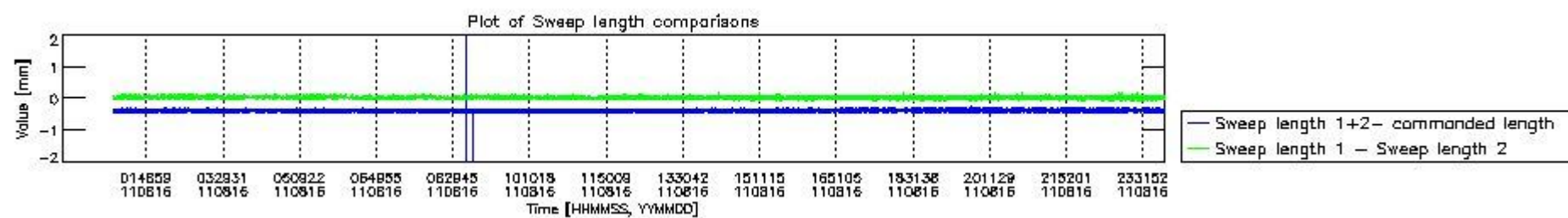
mipas_daily_report_level0_KSPT_L0_4504_N_20110816_8.PNG
