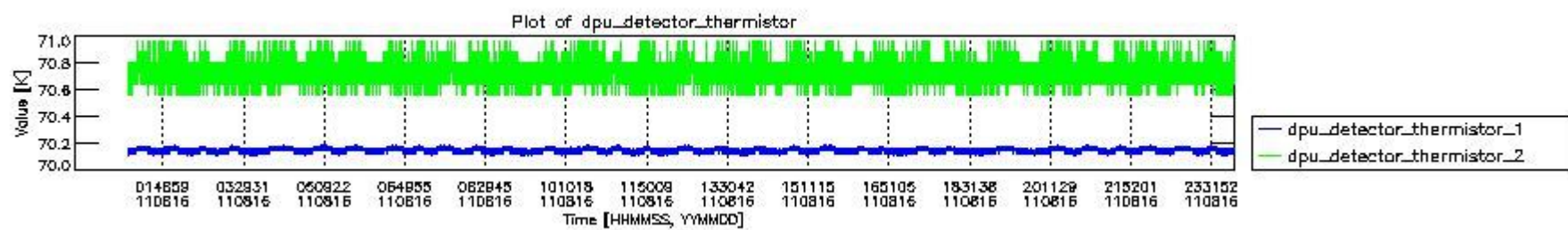
mipas_daily_report_level0_KSPT_L0_4504_N_20110816_3.PNG
