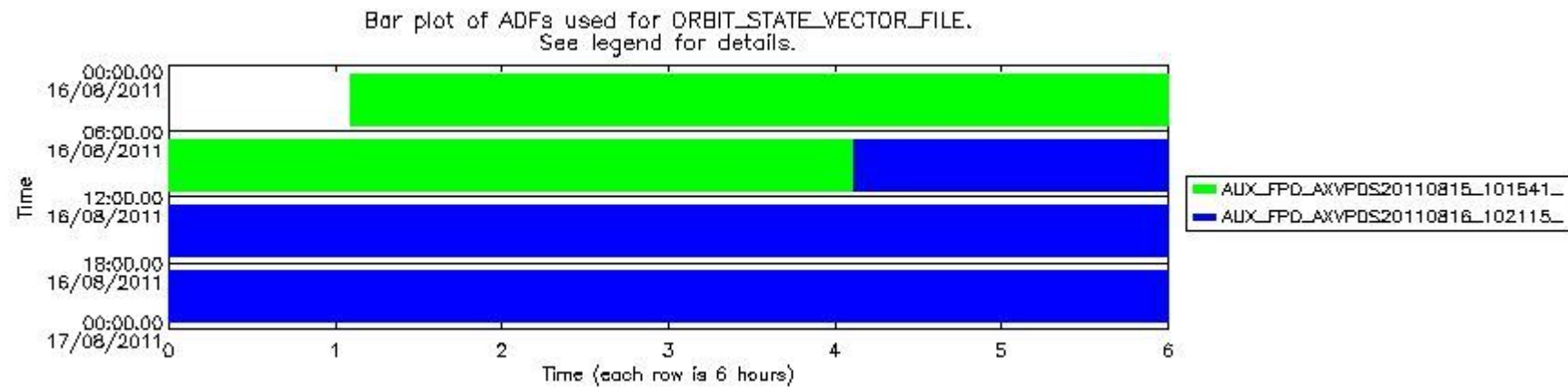
mipas_daily_report_level0_KSPT_L0_4504_N_20110816_13.PNG
