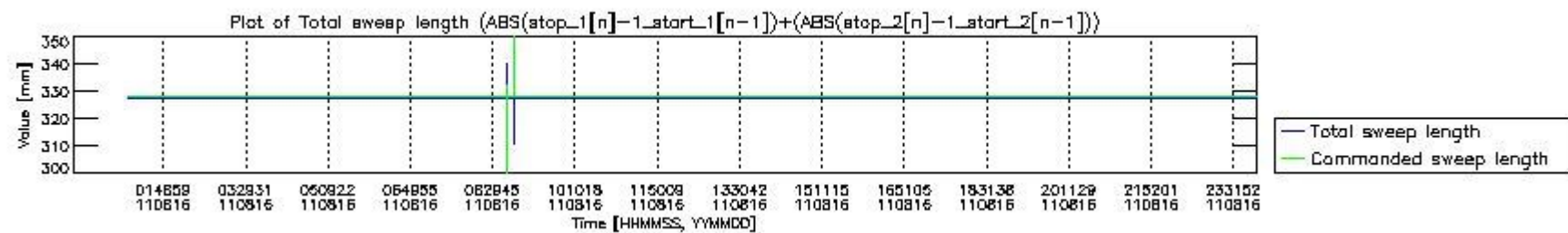
mipas_daily_report_level0_KSPT_L0_4504_N_20110816_6.PNG
