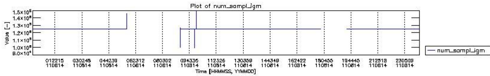
mipas_daily_report_level0_KSPT_L0_4504_N_20110814_0.PNG
