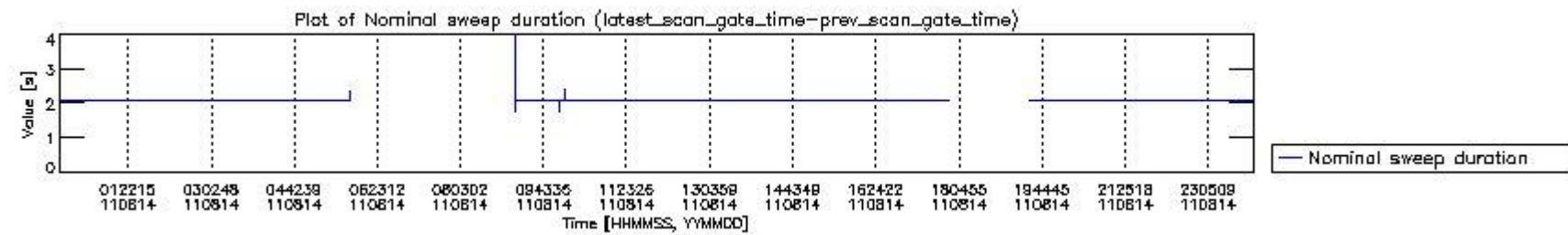
mipas_daily_report_level0_KSPT_L0_4504_N_20110814_4.PNG
