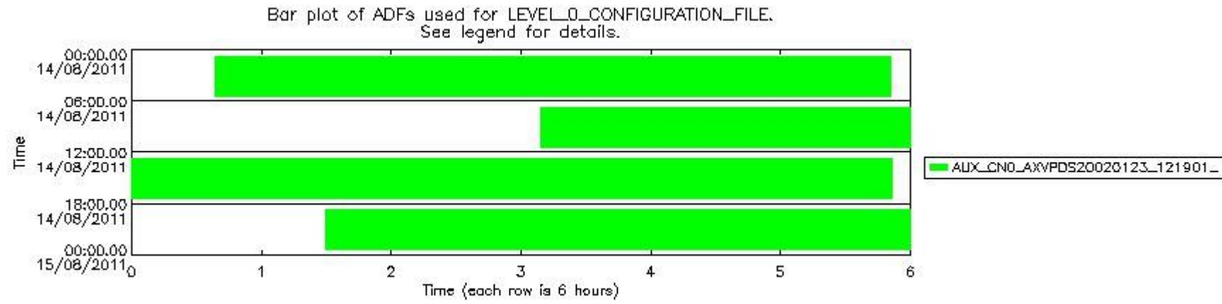
mipas_daily_report_level0_KSPT_L0_4504_N_20110814_12.PNG
