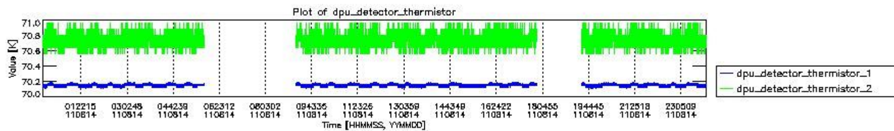
mipas_daily_report_level0_KSPT_L0_4504_N_20110814_3.PNG
