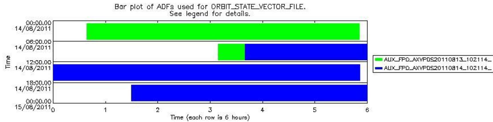
mipas_daily_report_level0_KSPT_L0_4504_N_20110814_13.PNG
