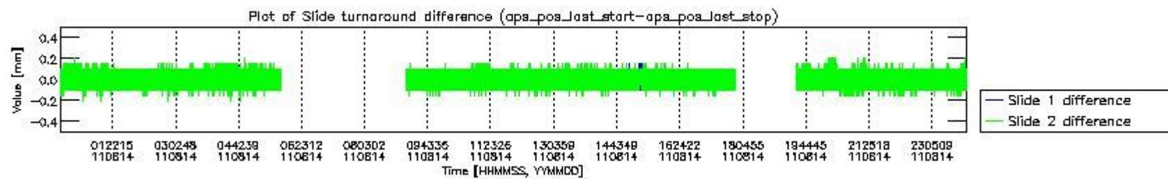
mipas_daily_report_level0_KSPT_L0_4504_N_20110814_5.PNG
