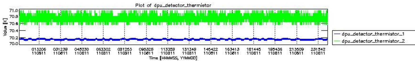
mipas_daily_report_level0_KSPT_L0_4504_N_20110811_3.PNG
