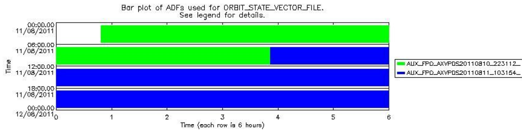
mipas_daily_report_level0_KSPT_L0_4504_N_20110811_13.PNG
