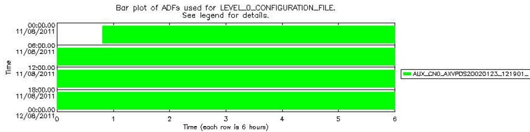
mipas_daily_report_level0_KSPT_L0_4504_N_20110811_12.PNG
