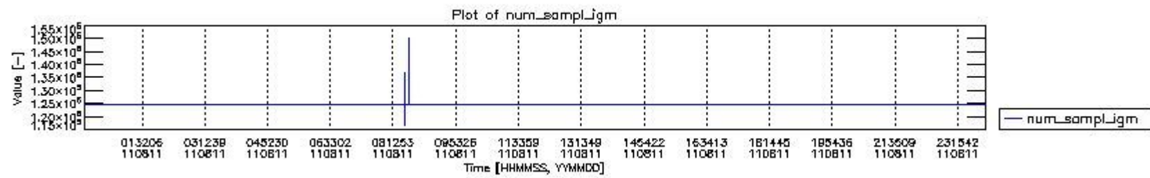
mipas_daily_report_level0_KSPT_L0_4504_N_20110811_0.PNG
