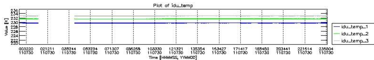
mipas_daily_report_level0_KSPT_L0_4504_N_20110730_2.PNG
