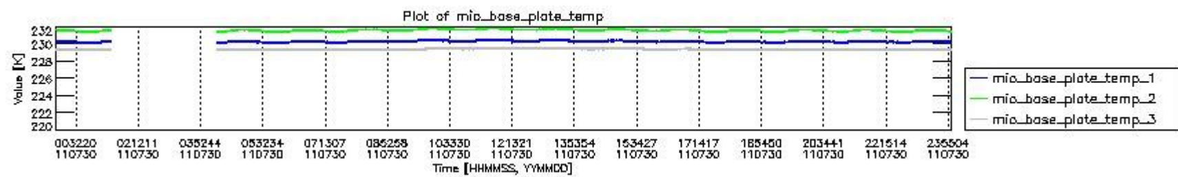
mipas_daily_report_level0_KSPT_L0_4504_N_20110730_1.PNG
