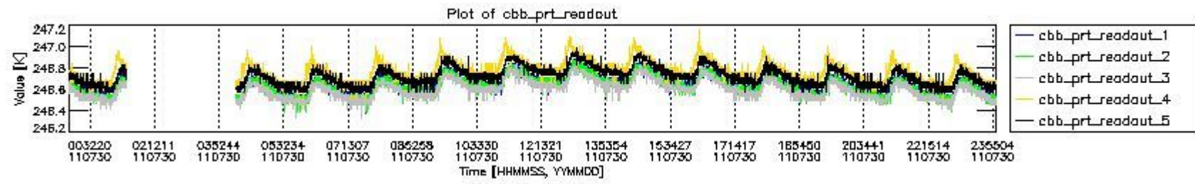
mipas_daily_report_level0_KSPT_L0_4504_N_20110730_9.PNG
