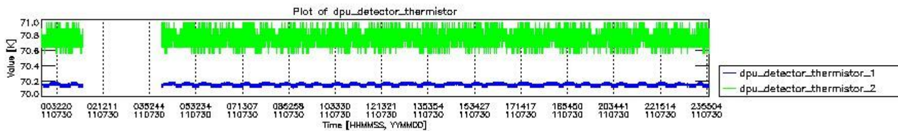
mipas_daily_report_level0_KSPT_L0_4504_N_20110730_3.PNG
