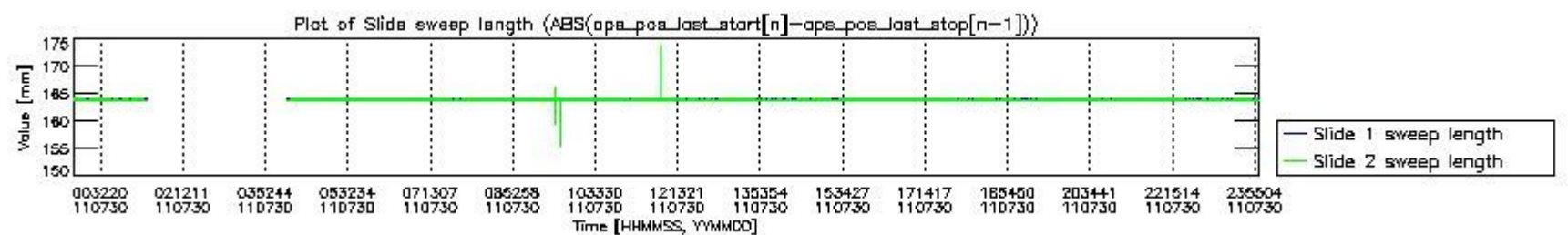
mipas_daily_report_level0_KSPT_L0_4504_N_20110730_7.PNG
