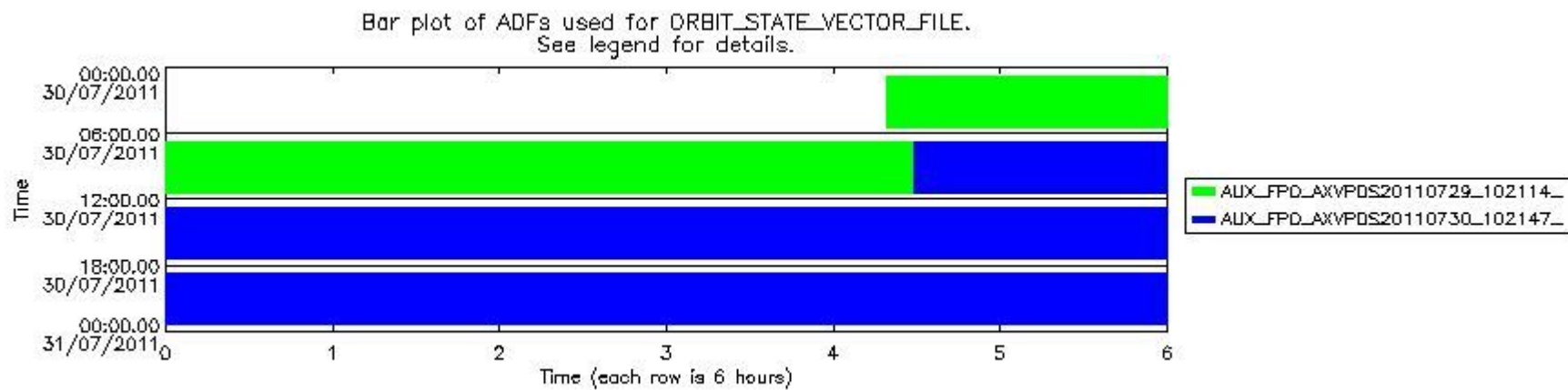
mipas_daily_report_level0_KSPT_L0_4504_N_20110730_13.PNG
