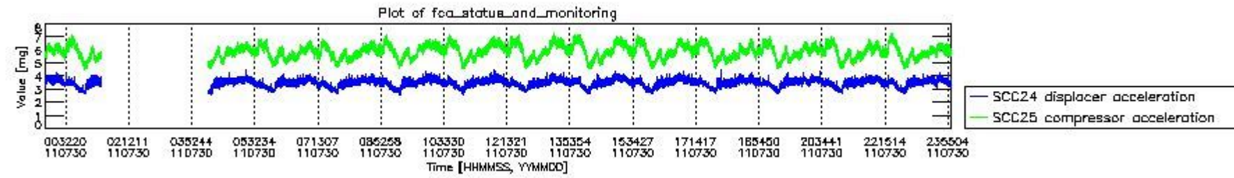
mipas_daily_report_level0_KSPT_L0_4504_N_20110730_10.PNG
