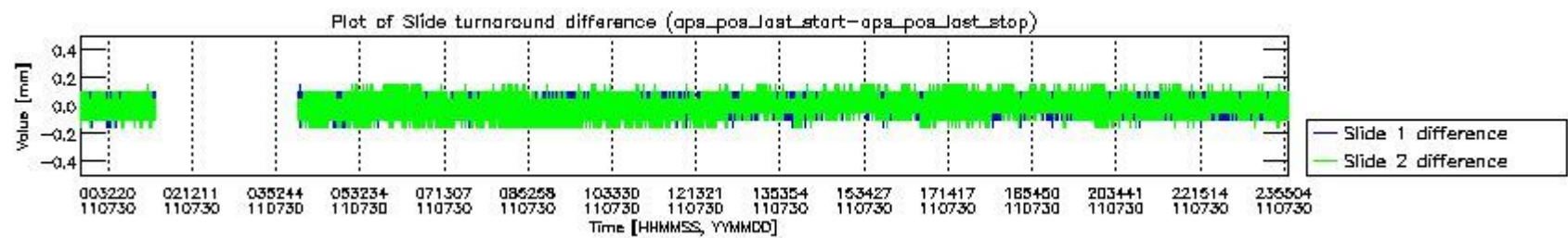
mipas_daily_report_level0_KSPT_L0_4504_N_20110730_5.PNG
