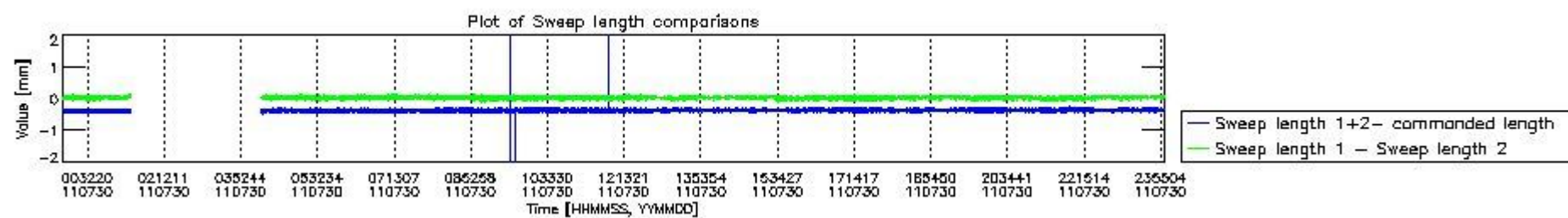
mipas_daily_report_level0_KSPT_L0_4504_N_20110730_8.PNG
