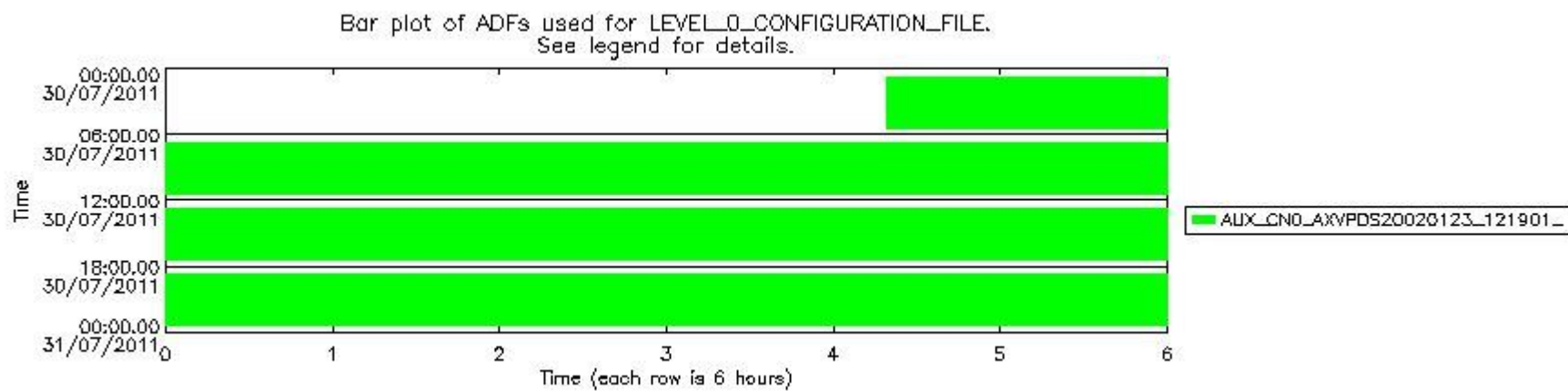
mipas_daily_report_level0_KSPT_L0_4504_N_20110730_12.PNG
