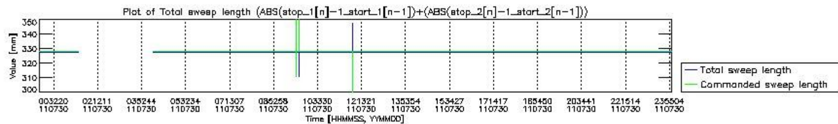
mipas_daily_report_level0_KSPT_L0_4504_N_20110730_6.PNG
