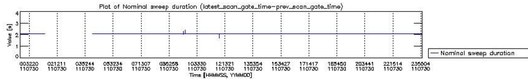
mipas_daily_report_level0_KSPT_L0_4504_N_20110730_4.PNG
