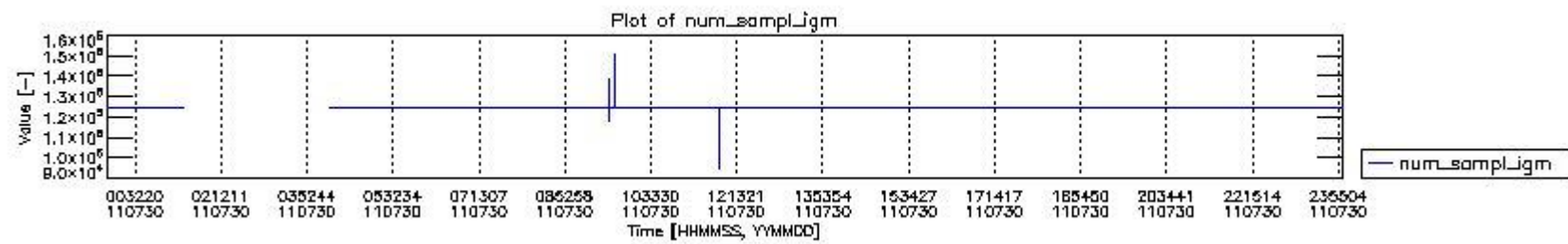
mipas_daily_report_level0_KSPT_L0_4504_N_20110730_0.PNG
