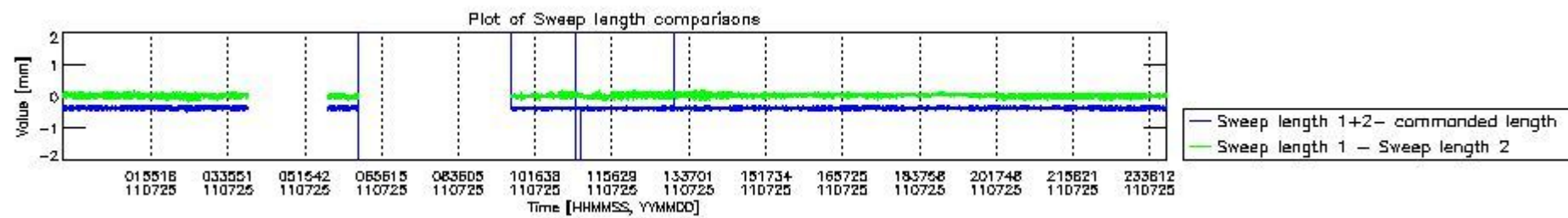
mipas_daily_report_level0_KSPT_L0_4504_N_20110725_8.PNG
