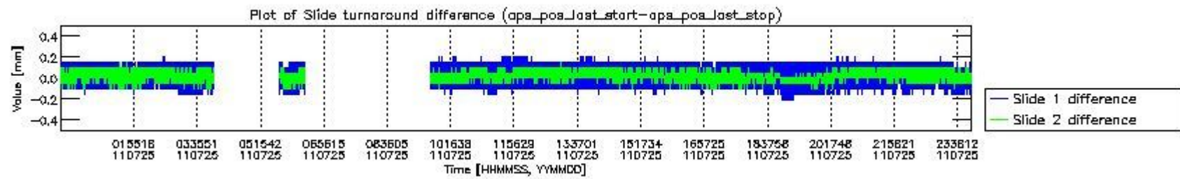
mipas_daily_report_level0_KSPT_L0_4504_N_20110725_5.PNG
