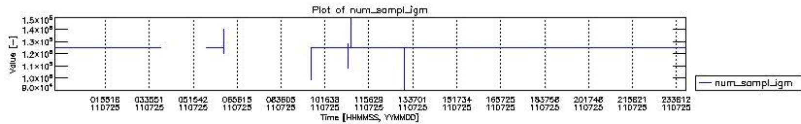
mipas_daily_report_level0_KSPT_L0_4504_N_20110725_0.PNG
