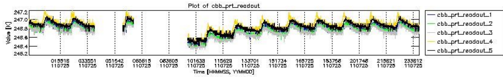
mipas_daily_report_level0_KSPT_L0_4504_N_20110725_9.PNG
