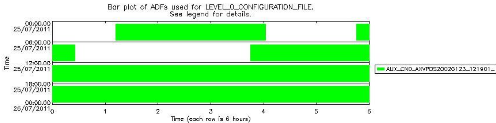
mipas_daily_report_level0_KSPT_L0_4504_N_20110725_12.PNG
