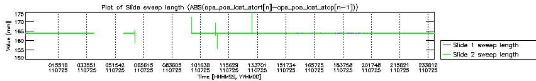
mipas_daily_report_level0_KSPT_L0_4504_N_20110725_7.PNG
