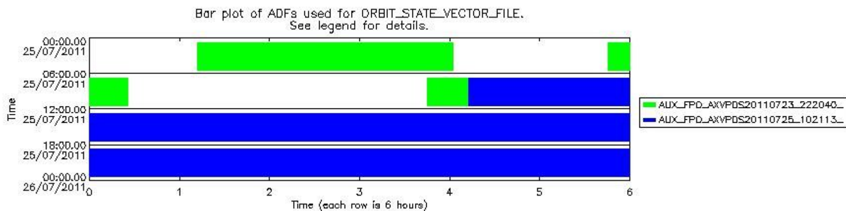
mipas_daily_report_level0_KSPT_L0_4504_N_20110725_13.PNG
