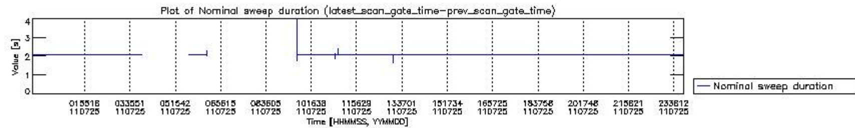
mipas_daily_report_level0_KSPT_L0_4504_N_20110725_4.PNG
