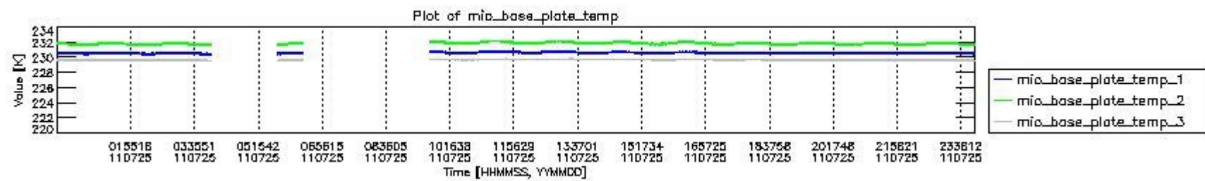
mipas_daily_report_level0_KSPT_L0_4504_N_20110725_1.PNG
