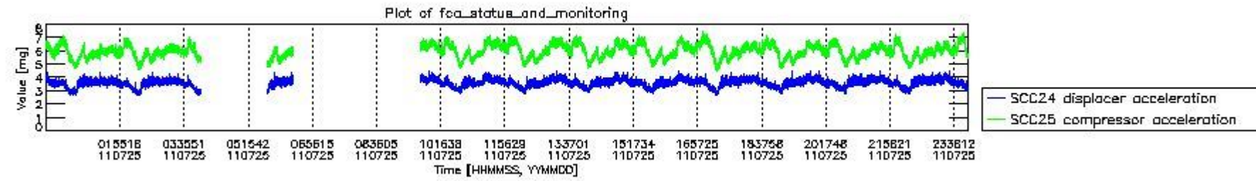
mipas_daily_report_level0_KSPT_L0_4504_N_20110725_10.PNG
