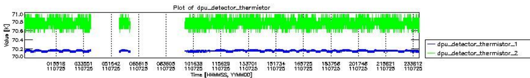
mipas_daily_report_level0_KSPT_L0_4504_N_20110725_3.PNG
