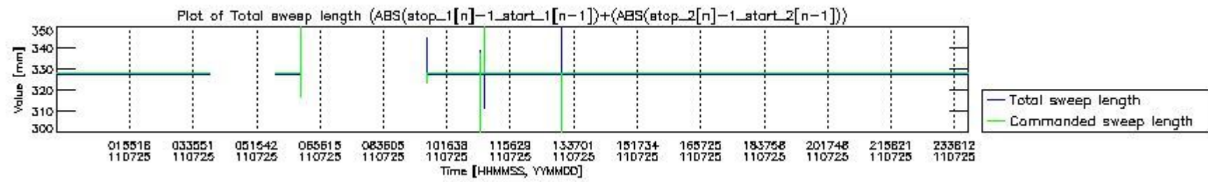
mipas_daily_report_level0_KSPT_L0_4504_N_20110725_6.PNG
