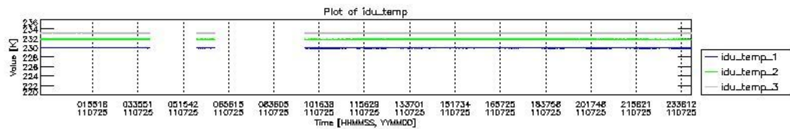
mipas_daily_report_level0_KSPT_L0_4504_N_20110725_2.PNG
