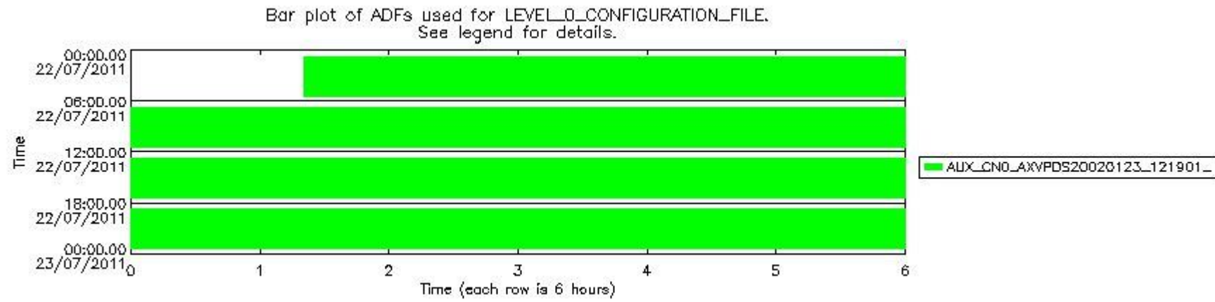
mipas_daily_report_level0_KSPT_L0_4504_N_20110722_12.PNG
