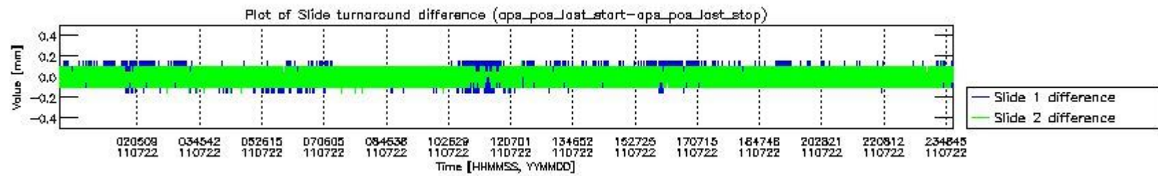
mipas_daily_report_level0_KSPT_L0_4504_N_20110722_5.PNG
