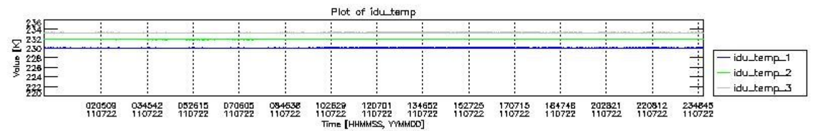
mipas_daily_report_level0_KSPT_L0_4504_N_20110722_2.PNG
