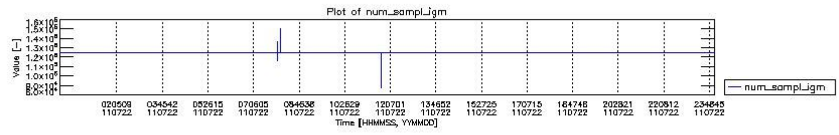
mipas_daily_report_level0_KSPT_L0_4504_N_20110722_0.PNG
