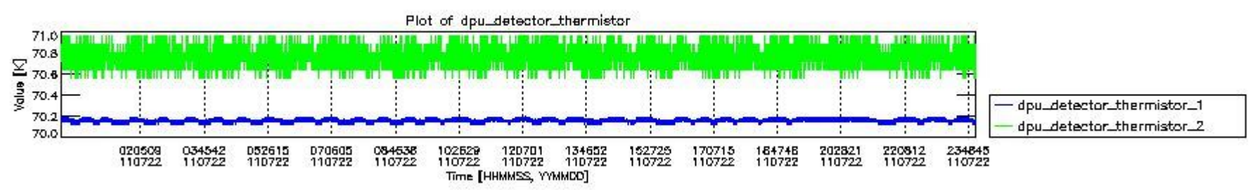
mipas_daily_report_level0_KSPT_L0_4504_N_20110722_3.PNG
