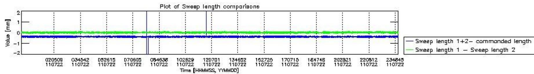
mipas_daily_report_level0_KSPT_L0_4504_N_20110722_8.PNG
