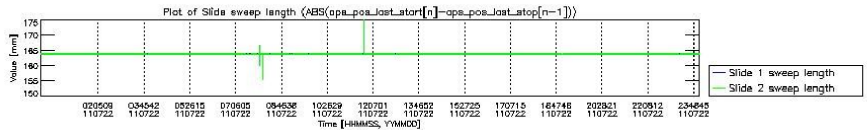
mipas_daily_report_level0_KSPT_L0_4504_N_20110722_7.PNG
