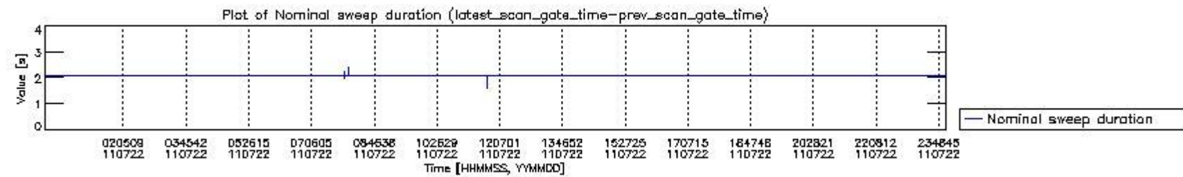
mipas_daily_report_level0_KSPT_L0_4504_N_20110722_4.PNG
