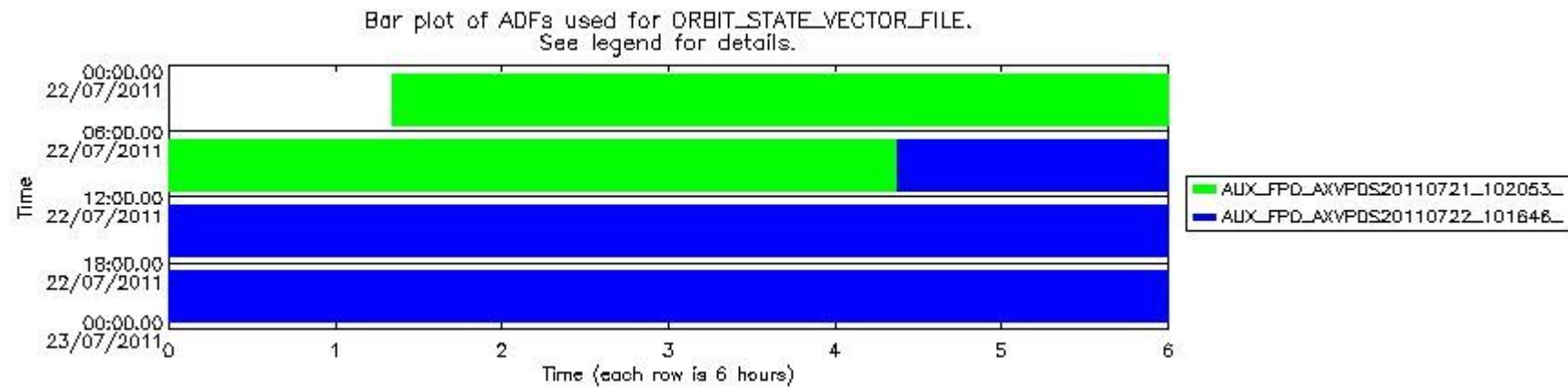
mipas_daily_report_level0_KSPT_L0_4504_N_20110722_13.PNG
