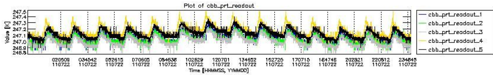
mipas_daily_report_level0_KSPT_L0_4504_N_20110722_9.PNG
