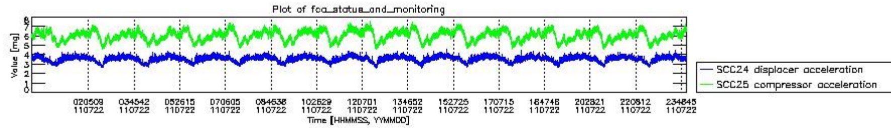
mipas_daily_report_level0_KSPT_L0_4504_N_20110722_10.PNG
