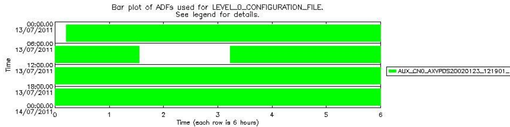
mipas_daily_report_level0_KSPT_L0_4504_N_20110713_12.PNG
