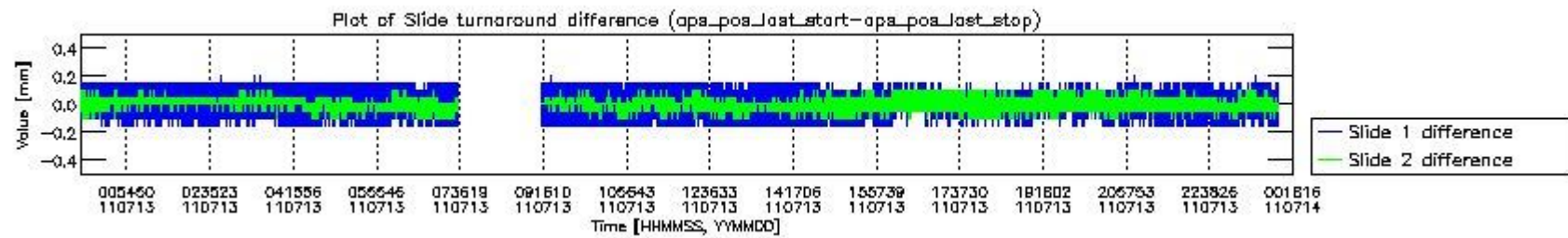
mipas_daily_report_level0_KSPT_L0_4504_N_20110713_5.PNG
