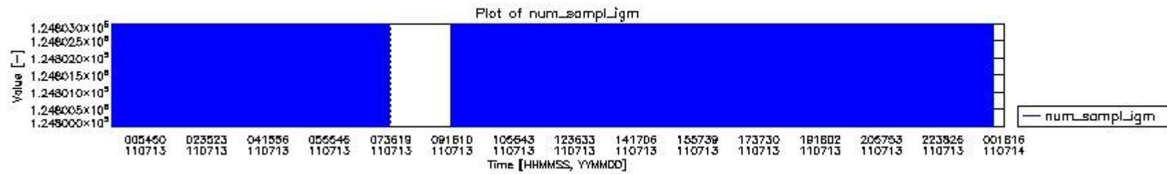
mipas_daily_report_level0_KSPT_L0_4504_N_20110713_0.PNG
