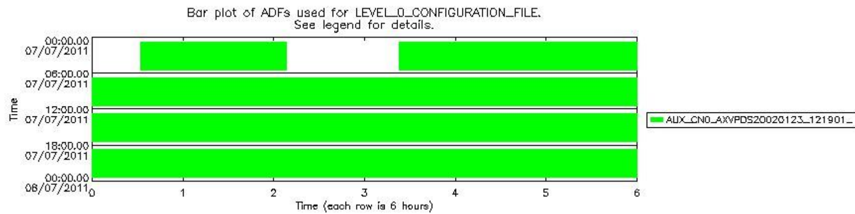
mipas_daily_report_level0_KSPT_L0_4504_N_20110707_12.PNG
