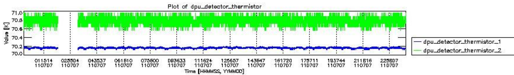
mipas_daily_report_level0_KSPT_L0_4504_N_20110707_3.PNG
