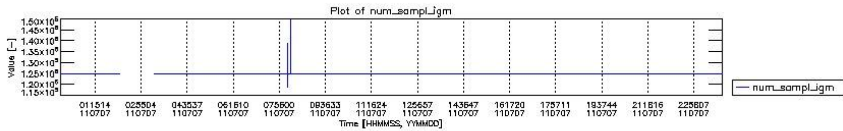
mipas_daily_report_level0_KSPT_L0_4504_N_20110707_0.PNG
