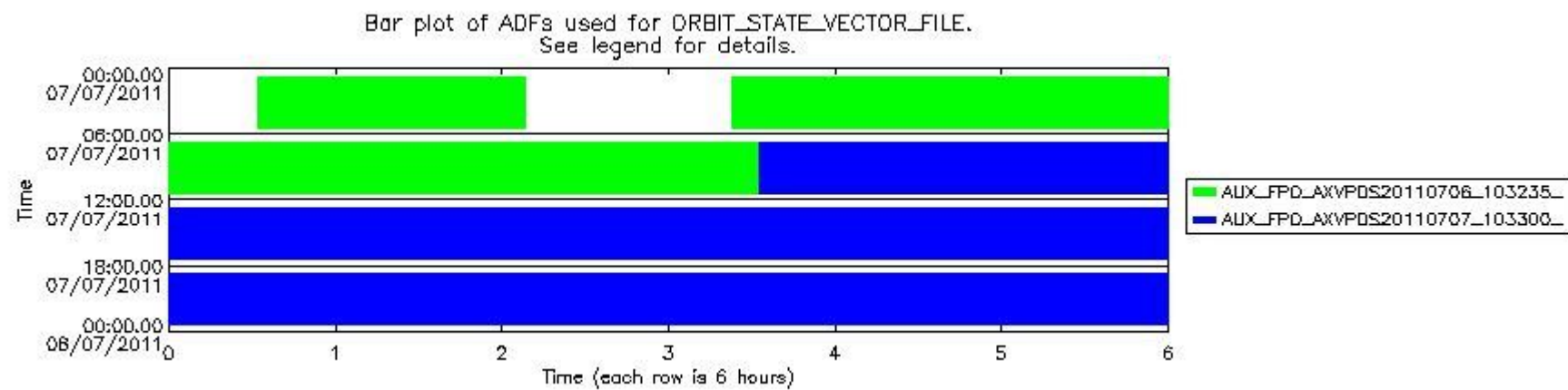
mipas_daily_report_level0_KSPT_L0_4504_N_20110707_13.PNG
