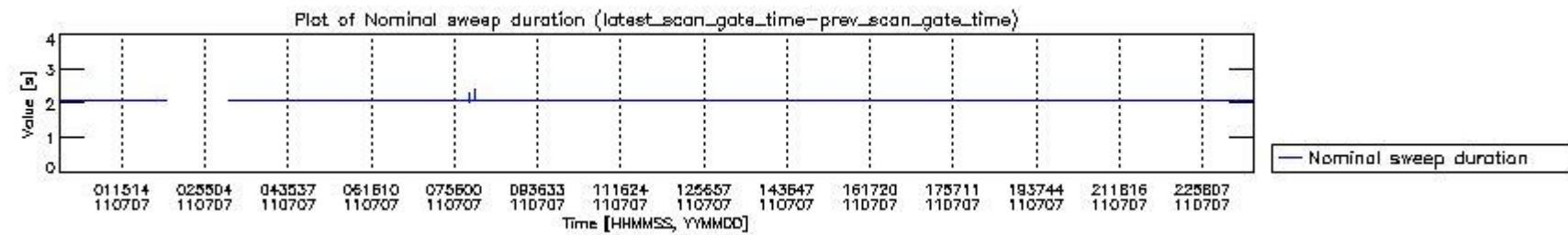
mipas_daily_report_level0_KSPT_L0_4504_N_20110707_4.PNG
