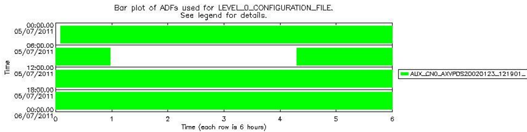
mipas_daily_report_level0_KSPT_L0_4504_N_20110705_12.PNG
