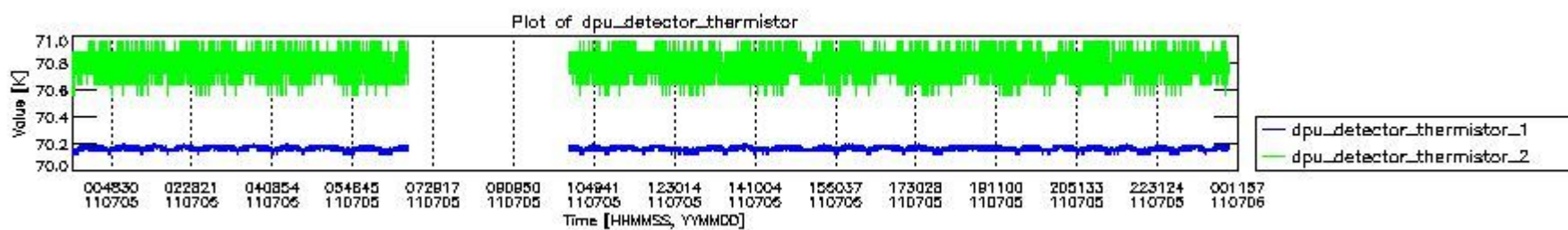
mipas_daily_report_level0_KSPT_L0_4504_N_20110705_3.PNG
