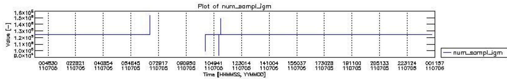
mipas_daily_report_level0_KSPT_L0_4504_N_20110705_0.PNG
