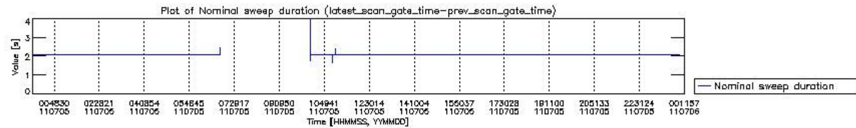
mipas_daily_report_level0_KSPT_L0_4504_N_20110705_4.PNG
