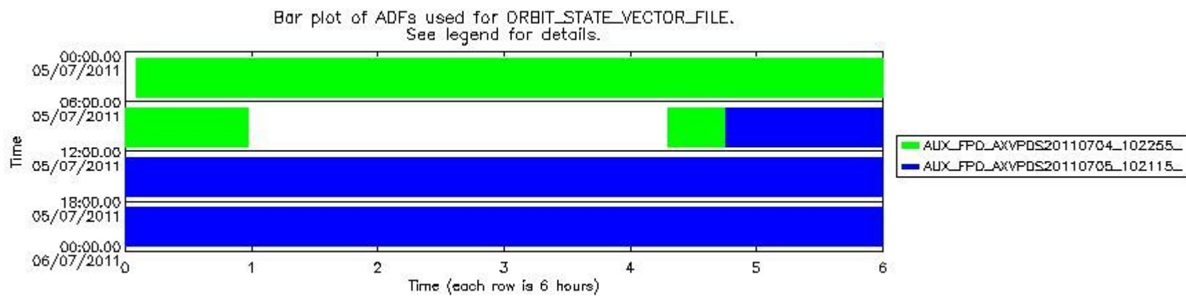
mipas_daily_report_level0_KSPT_L0_4504_N_20110705_13.PNG
