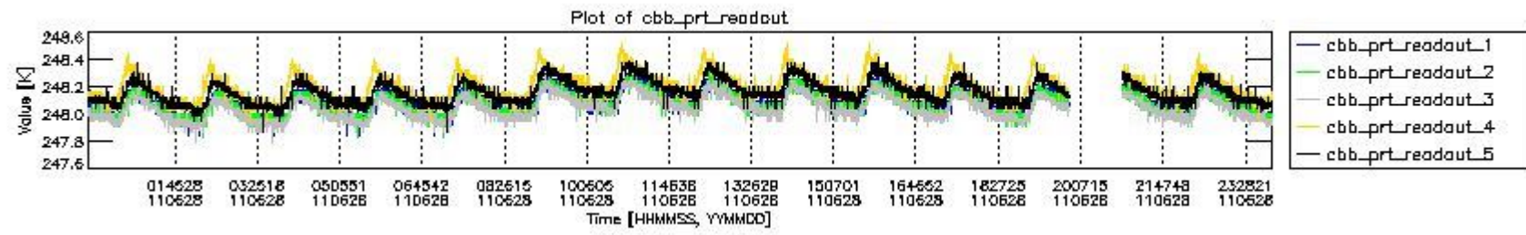
mipas_daily_report_level0_KSPT_L0_4504_N_20110628_9.PNG
