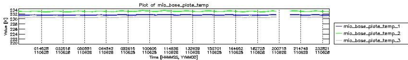
mipas_daily_report_level0_KSPT_L0_4504_N_20110628_1.PNG
