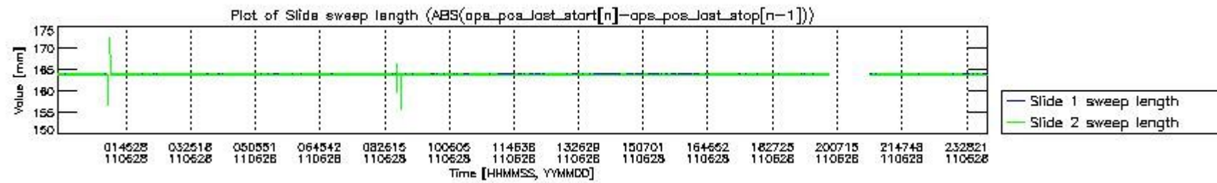
mipas_daily_report_level0_KSPT_L0_4504_N_20110628_7.PNG
