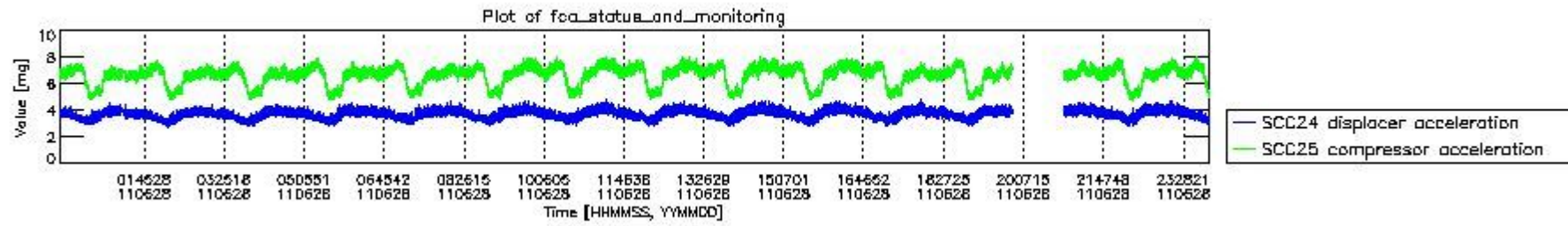
mipas_daily_report_level0_KSPT_L0_4504_N_20110628_10.PNG
