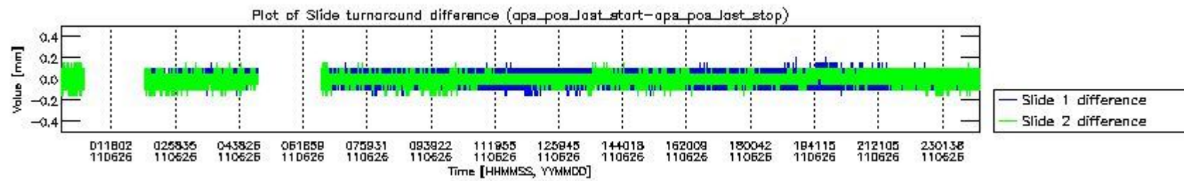
mipas_daily_report_level0_KSPT_L0_4504_N_20110626_5.PNG
