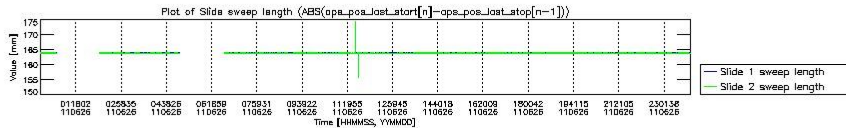
mipas_daily_report_level0_KSPT_L0_4504_N_20110626_7.PNG
