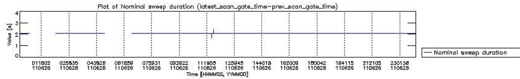
mipas_daily_report_level0_KSPT_L0_4504_N_20110626_4.PNG
