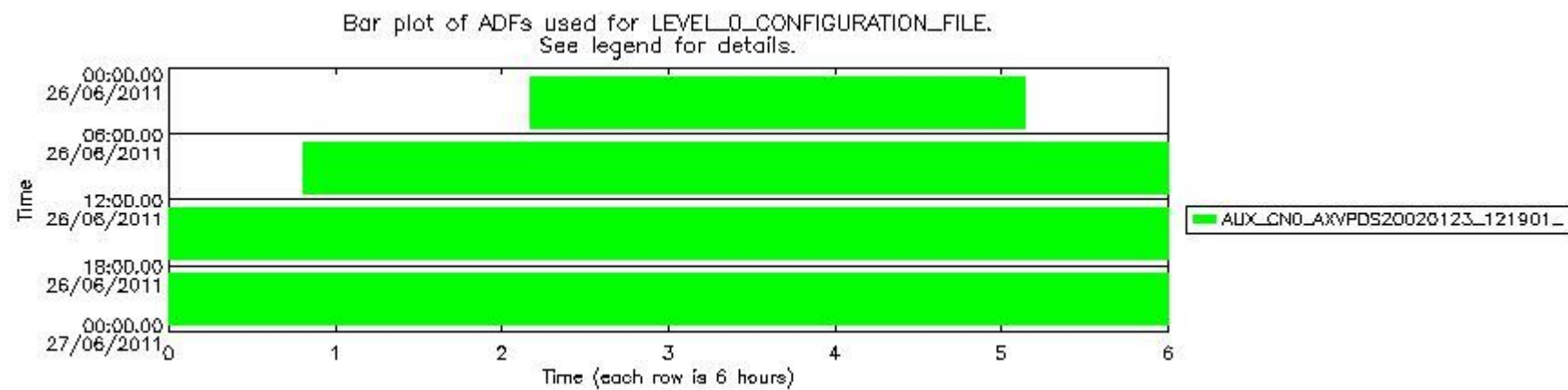
mipas_daily_report_level0_KSPT_L0_4504_N_20110626_12.PNG
