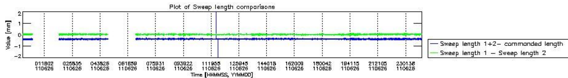
mipas_daily_report_level0_KSPT_L0_4504_N_20110626_8.PNG
