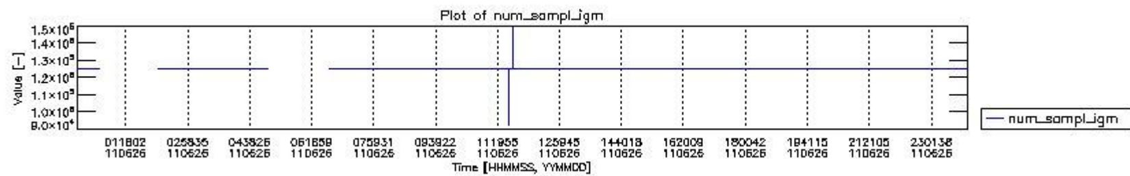
mipas_daily_report_level0_KSPT_L0_4504_N_20110626_0.PNG
