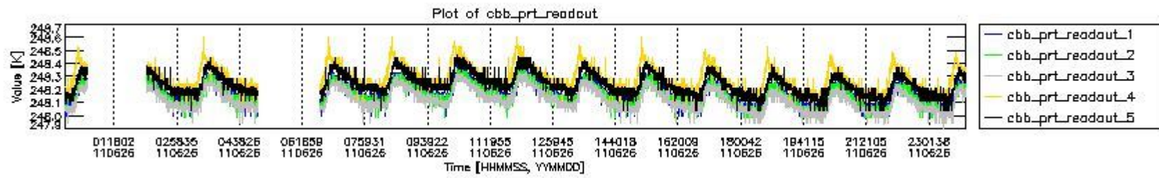
mipas_daily_report_level0_KSPT_L0_4504_N_20110626_9.PNG
