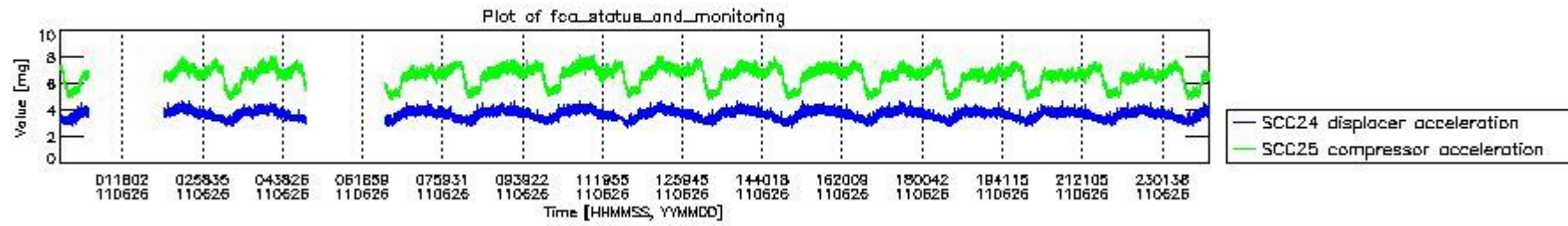
mipas_daily_report_level0_KSPT_L0_4504_N_20110626_10.PNG
