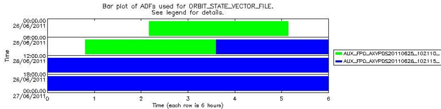
mipas_daily_report_level0_KSPT_L0_4504_N_20110626_13.PNG
