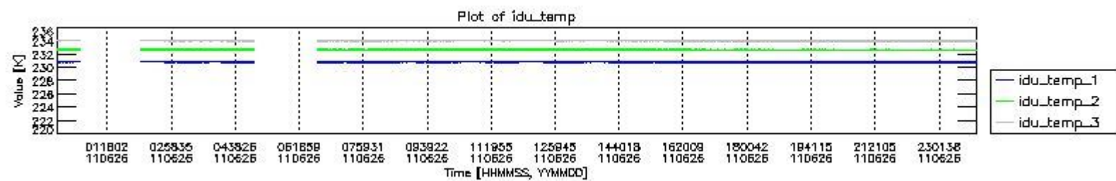
mipas_daily_report_level0_KSPT_L0_4504_N_20110626_2.PNG
