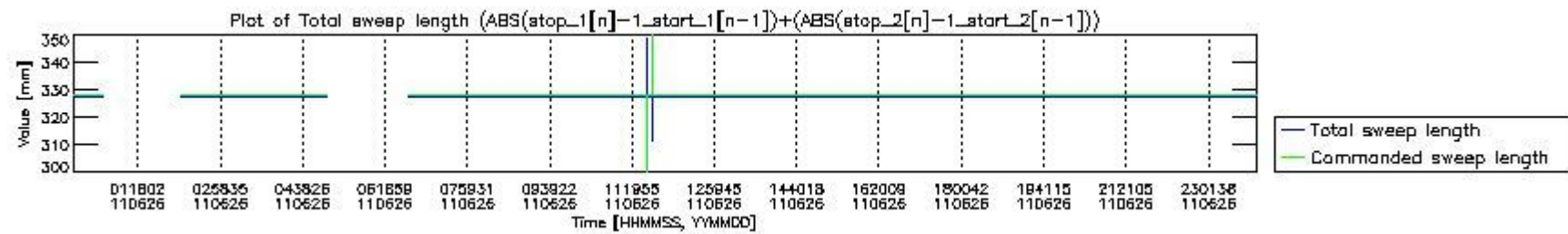
mipas_daily_report_level0_KSPT_L0_4504_N_20110626_6.PNG
