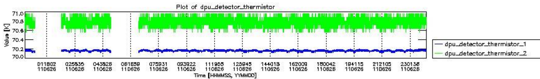
mipas_daily_report_level0_KSPT_L0_4504_N_20110626_3.PNG
