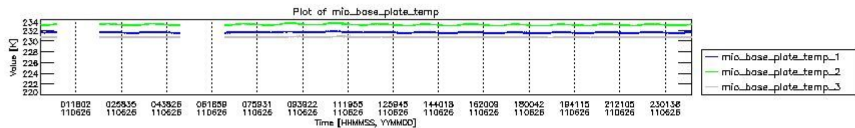
mipas_daily_report_level0_KSPT_L0_4504_N_20110626_1.PNG
