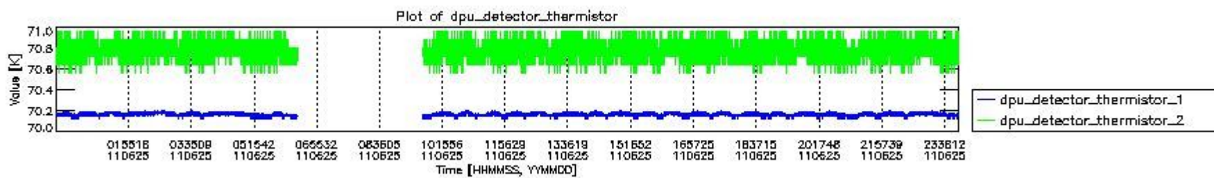
mipas_daily_report_level0_KSPT_L0_4504_N_20110625_3.PNG
