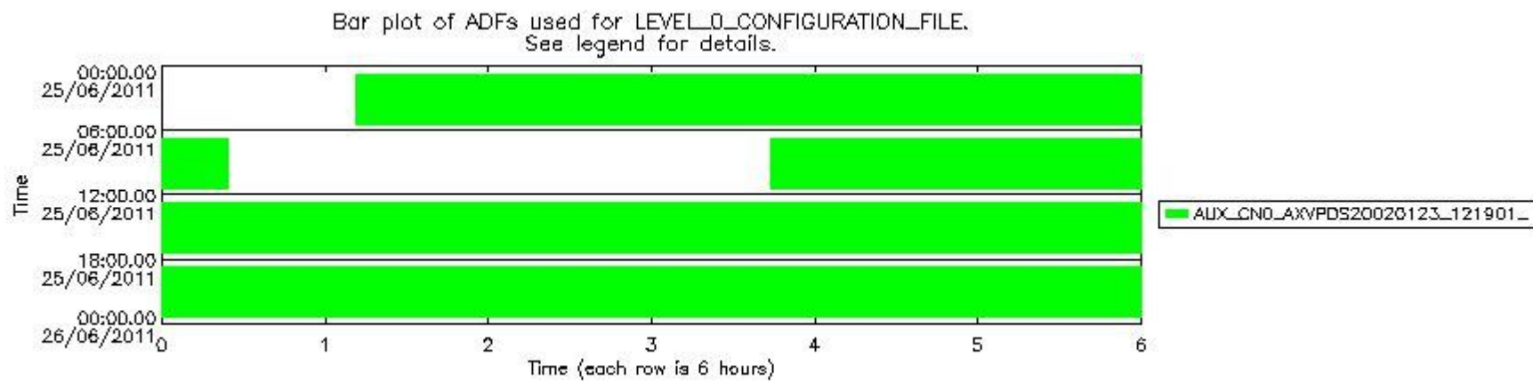
mipas_daily_report_level0_KSPT_L0_4504_N_20110625_12.PNG
