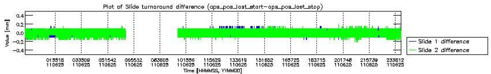
mipas_daily_report_level0_KSPT_L0_4504_N_20110625_5.PNG
