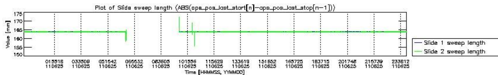
mipas_daily_report_level0_KSPT_L0_4504_N_20110625_7.PNG
