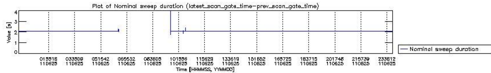
mipas_daily_report_level0_KSPT_L0_4504_N_20110625_4.PNG
