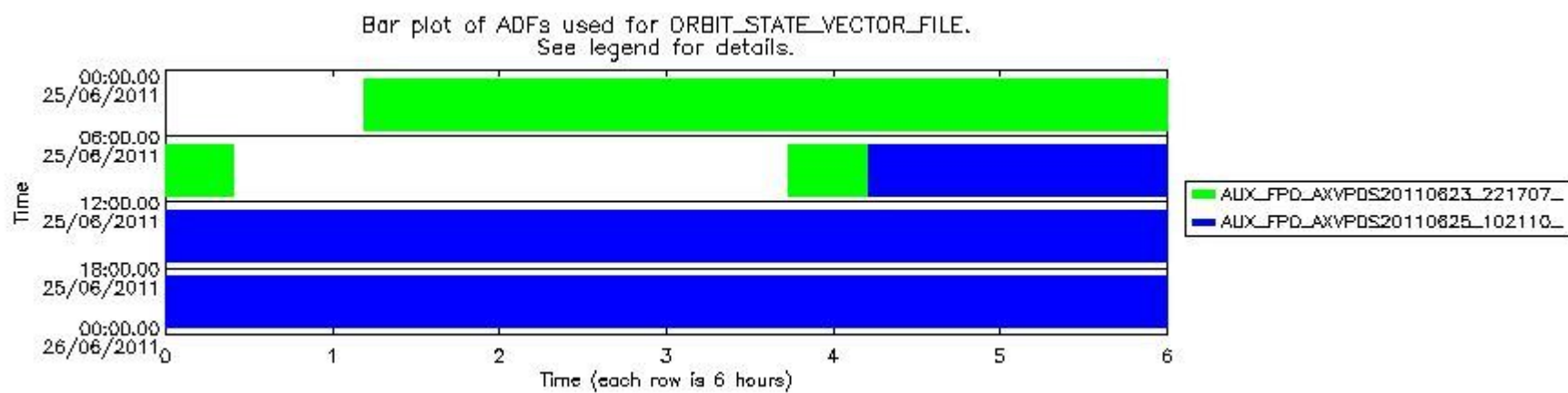
mipas_daily_report_level0_KSPT_L0_4504_N_20110625_13.PNG
