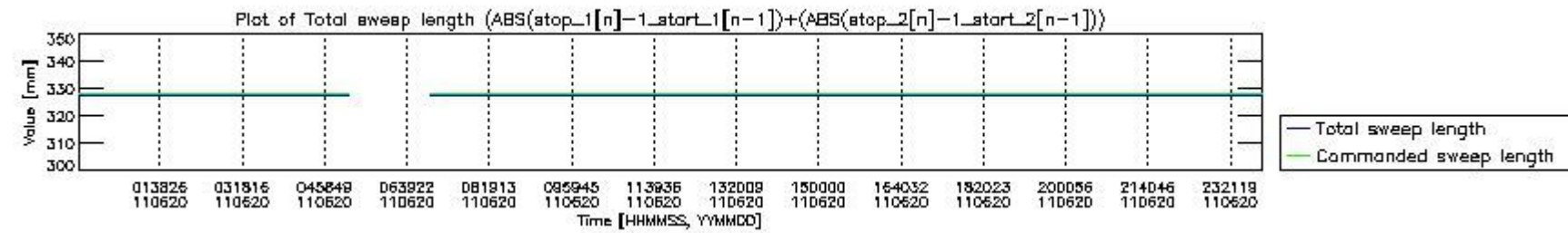
mipas_daily_report_level0_KSPT_L0_4504_N_20110620_6.PNG
