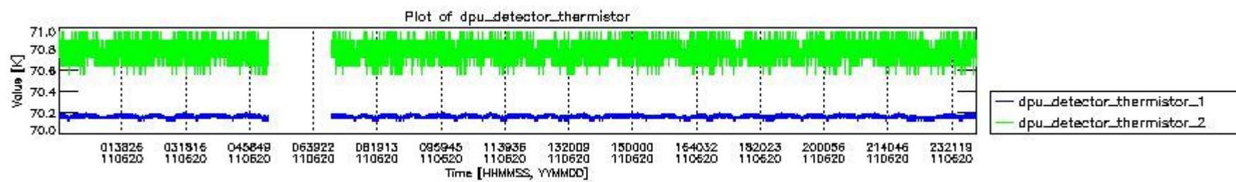
mipas_daily_report_level0_KSPT_L0_4504_N_20110620_3.PNG
