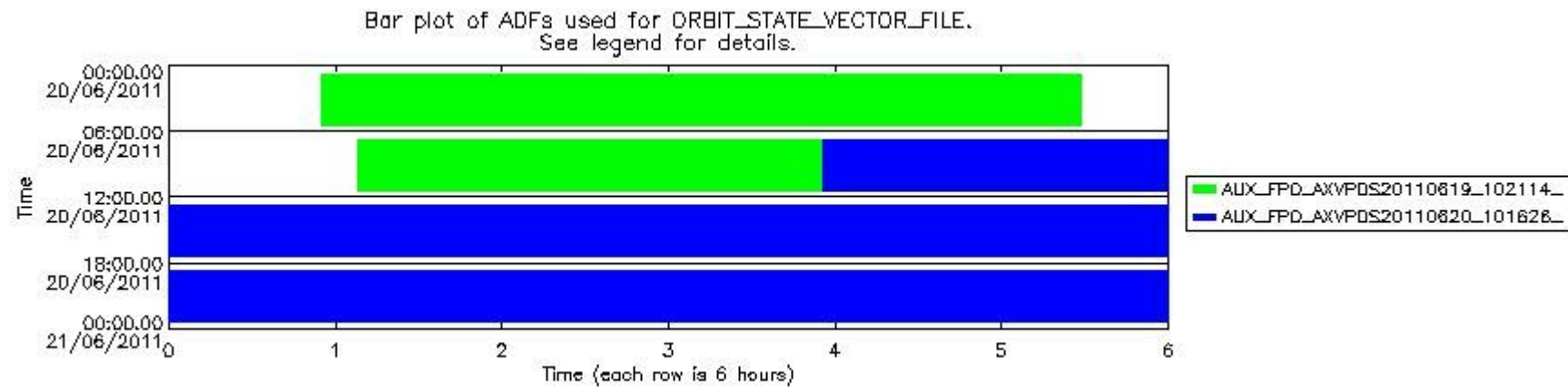
mipas_daily_report_level0_KSPT_L0_4504_N_20110620_13.PNG
