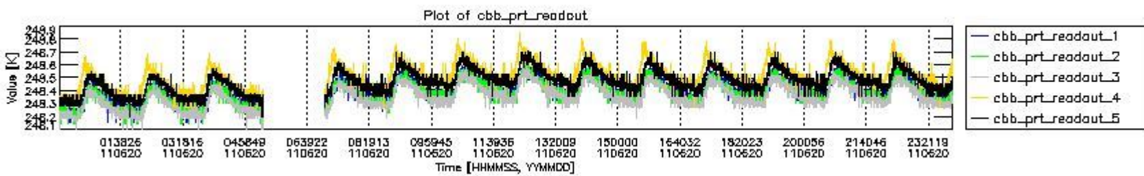
mipas_daily_report_level0_KSPT_L0_4504_N_20110620_9.PNG
