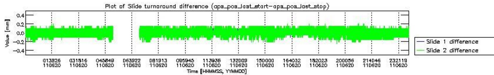
mipas_daily_report_level0_KSPT_L0_4504_N_20110620_5.PNG
