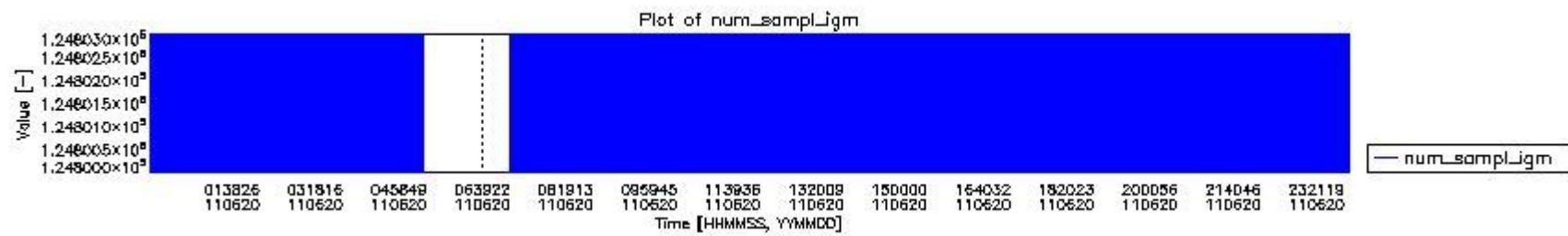
mipas_daily_report_level0_KSPT_L0_4504_N_20110620_0.PNG
