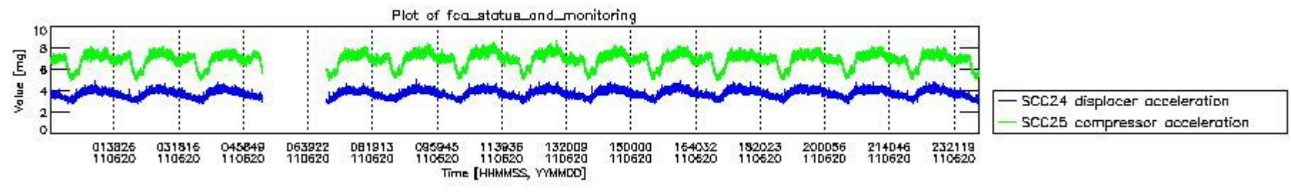
mipas_daily_report_level0_KSPT_L0_4504_N_20110620_10.PNG
