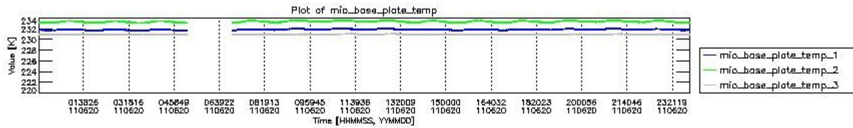
mipas_daily_report_level0_KSPT_L0_4504_N_20110620_1.PNG
