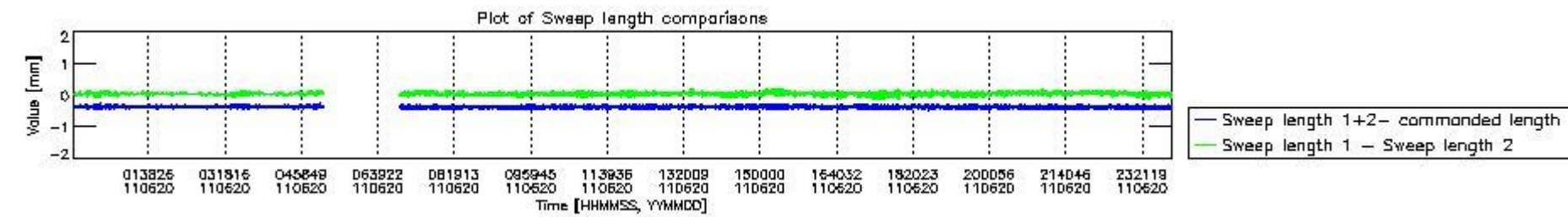
mipas_daily_report_level0_KSPT_L0_4504_N_20110620_8.PNG
