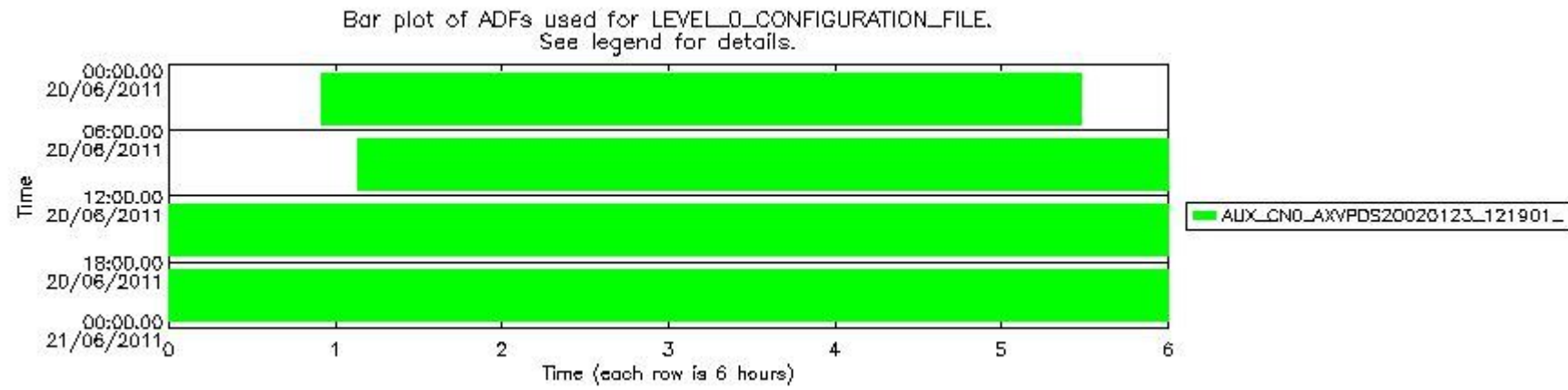
mipas_daily_report_level0_KSPT_L0_4504_N_20110620_12.PNG
