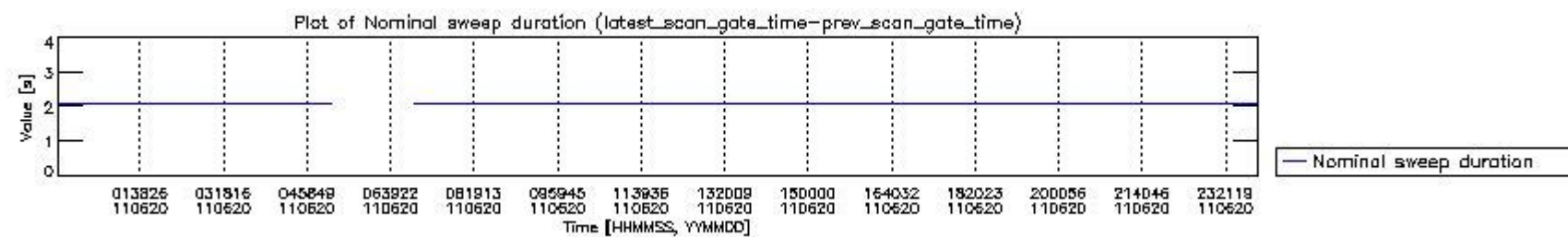
mipas_daily_report_level0_KSPT_L0_4504_N_20110620_4.PNG
