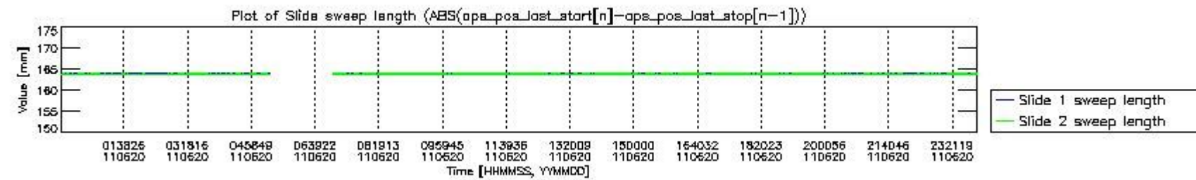
mipas_daily_report_level0_KSPT_L0_4504_N_20110620_7.PNG
