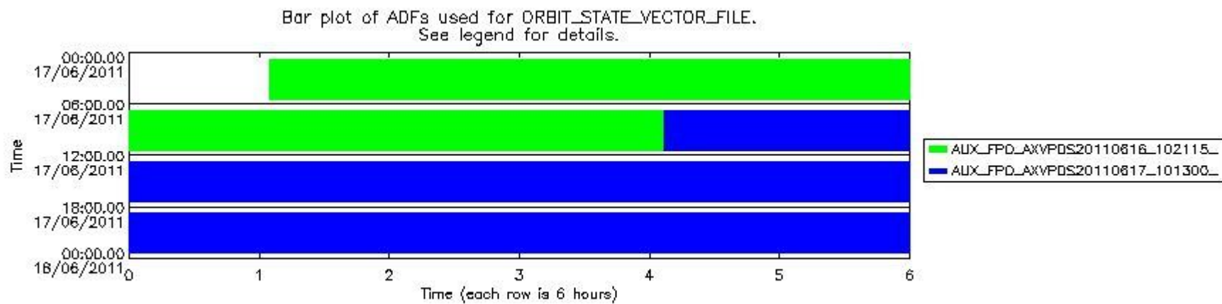
mipas_daily_report_level0_KSPT_L0_4504_N_20110617_13.PNG
