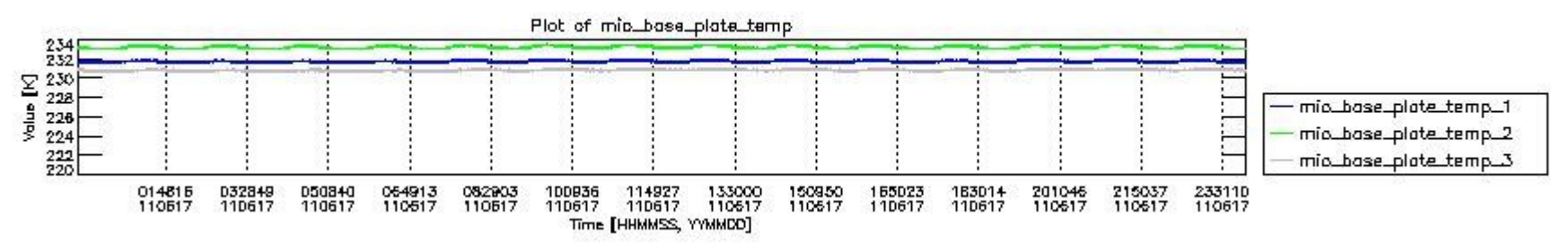
mipas_daily_report_level0_KSPT_L0_4504_N_20110617_1.PNG
