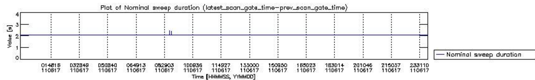
mipas_daily_report_level0_KSPT_L0_4504_N_20110617_4.PNG
