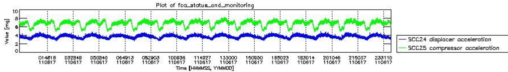
mipas_daily_report_level0_KSPT_L0_4504_N_20110617_10.PNG
