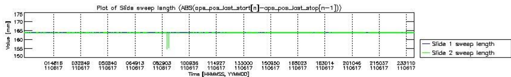
mipas_daily_report_level0_KSPT_L0_4504_N_20110617_7.PNG
