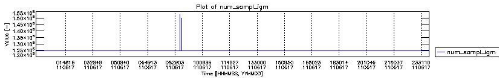
mipas_daily_report_level0_KSPT_L0_4504_N_20110617_0.PNG
