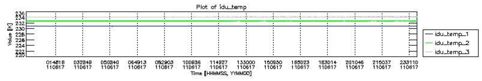
mipas_daily_report_level0_KSPT_L0_4504_N_20110617_2.PNG
