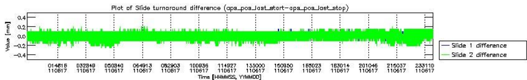
mipas_daily_report_level0_KSPT_L0_4504_N_20110617_5.PNG
