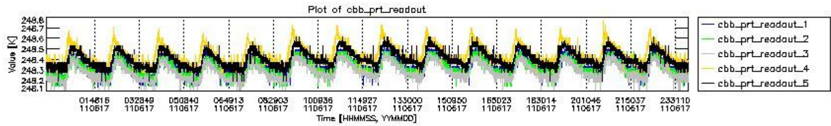
mipas_daily_report_level0_KSPT_L0_4504_N_20110617_9.PNG
