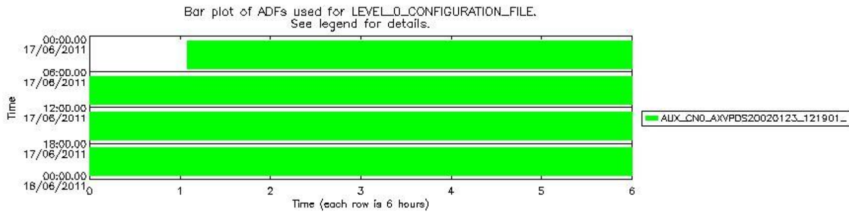
mipas_daily_report_level0_KSPT_L0_4504_N_20110617_12.PNG
