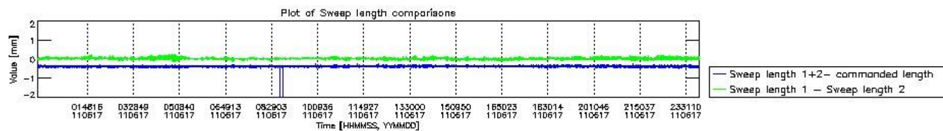
mipas_daily_report_level0_KSPT_L0_4504_N_20110617_8.PNG
