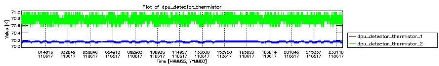
mipas_daily_report_level0_KSPT_L0_4504_N_20110617_3.PNG
