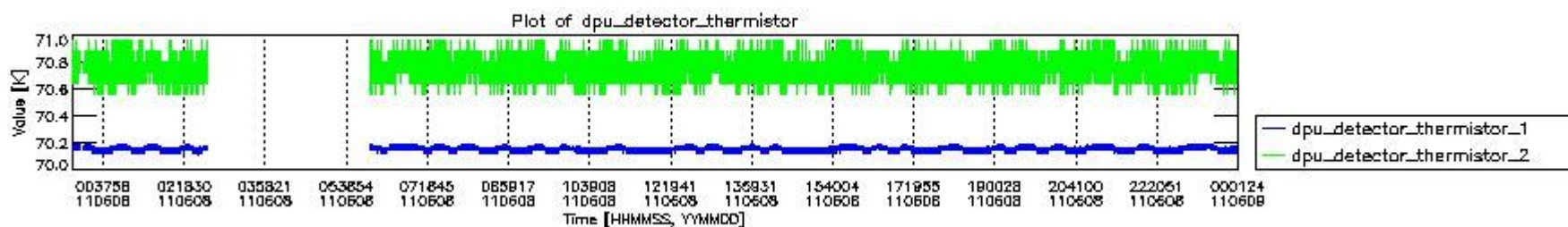
mipas_daily_report_level0_KSPT_L0_4504_N_20110608_3.PNG
