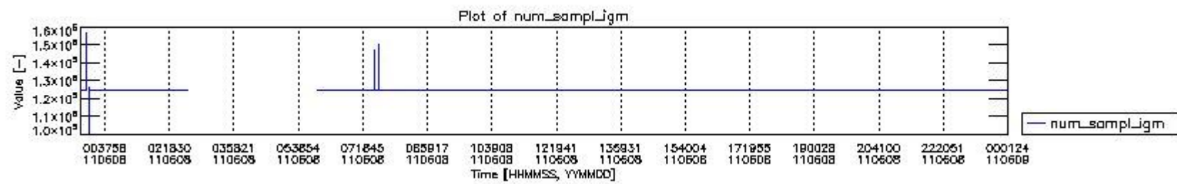
mipas_daily_report_level0_KSPT_L0_4504_N_20110608_0.PNG
