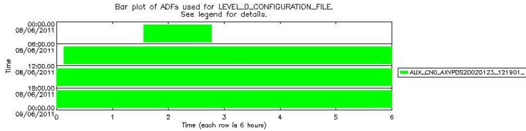
mipas_daily_report_level0_KSPT_L0_4504_N_20110608_12.PNG
