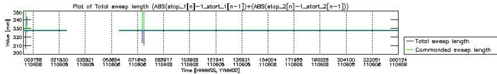
mipas_daily_report_level0_KSPT_L0_4504_N_20110608_6.PNG
