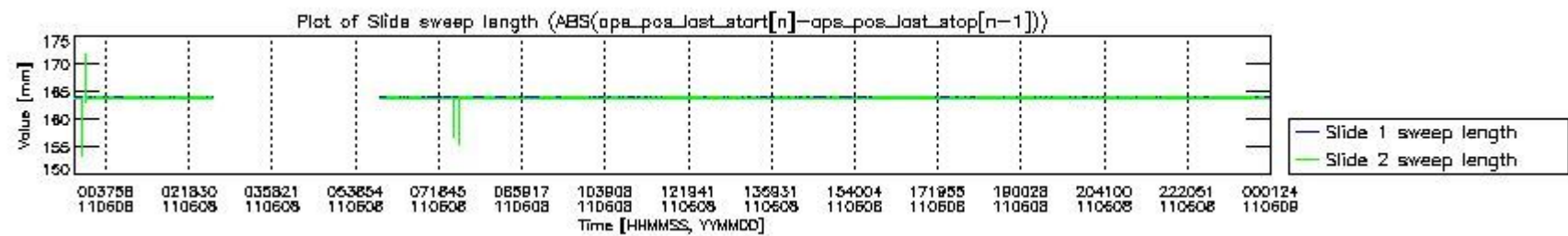
mipas_daily_report_level0_KSPT_L0_4504_N_20110608_7.PNG
