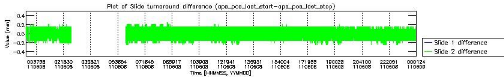
mipas_daily_report_level0_KSPT_L0_4504_N_20110608_5.PNG
