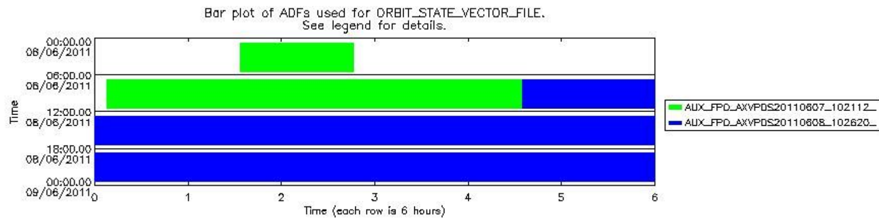
mipas_daily_report_level0_KSPT_L0_4504_N_20110608_13.PNG
