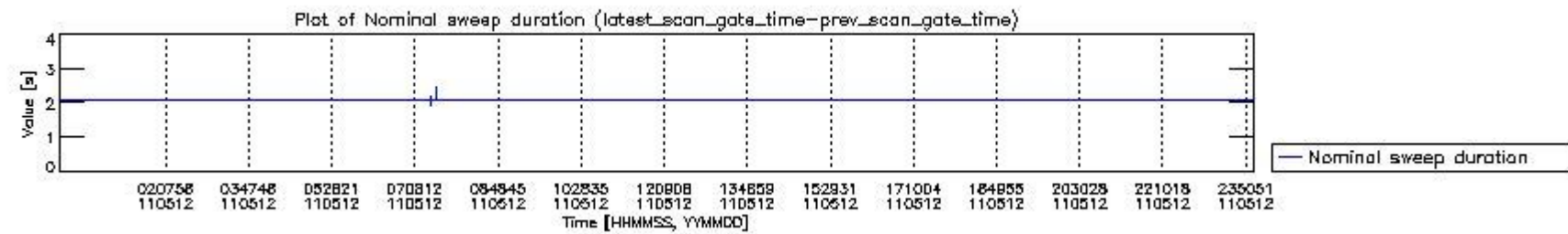
mipas_daily_report_level0_KSPT_L0_4504_N_20110512_4.PNG
