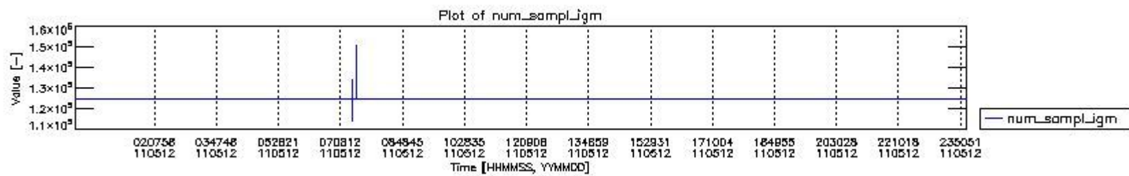
mipas_daily_report_level0_KSPT_L0_4504_N_20110512_0.PNG
