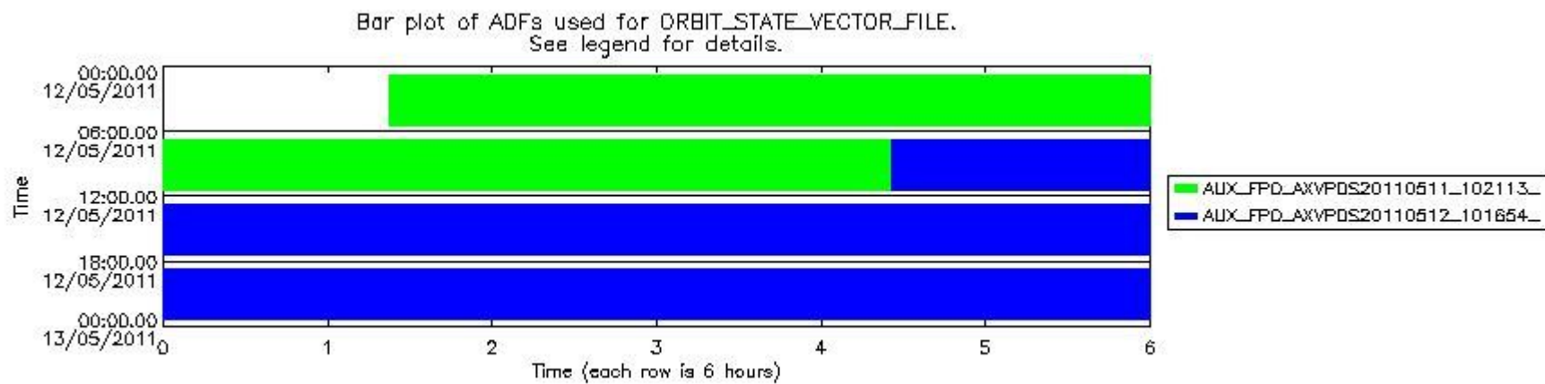
mipas_daily_report_level0_KSPT_L0_4504_N_20110512_13.PNG
