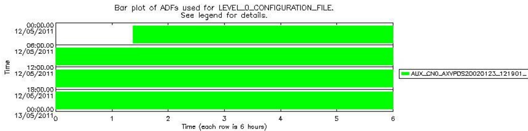
mipas_daily_report_level0_KSPT_L0_4504_N_20110512_12.PNG
