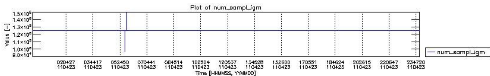
mipas_daily_report_level0_KSPT_L0_4504_N_20110423_0.PNG
