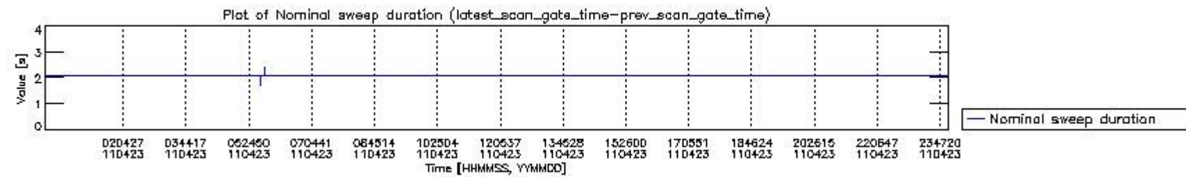
mipas_daily_report_level0_KSPT_L0_4504_N_20110423_4.PNG
