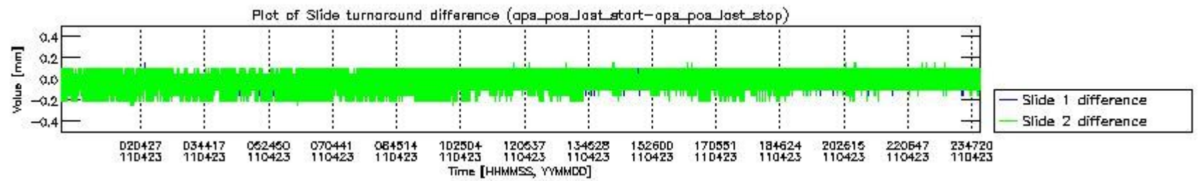
mipas_daily_report_level0_KSPT_L0_4504_N_20110423_5.PNG
