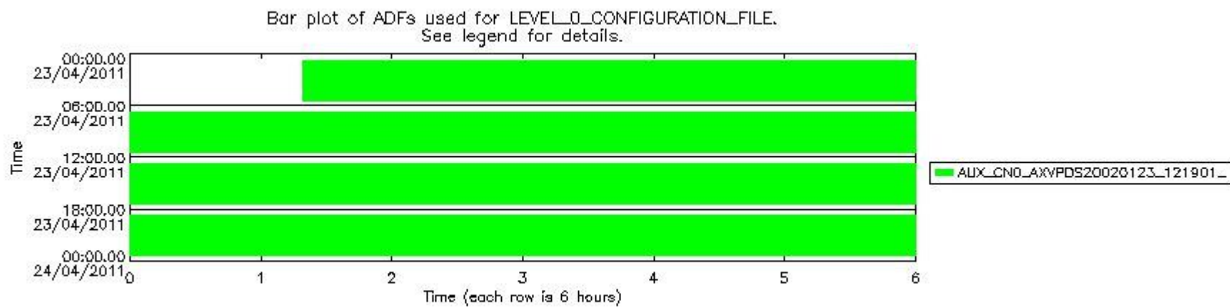
mipas_daily_report_level0_KSPT_L0_4504_N_20110423_12.PNG
