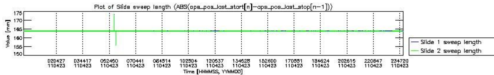
mipas_daily_report_level0_KSPT_L0_4504_N_20110423_7.PNG
