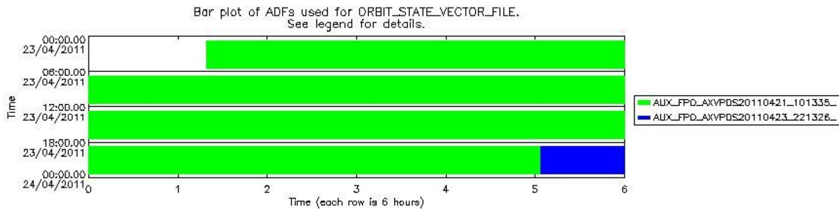
mipas_daily_report_level0_KSPT_L0_4504_N_20110423_13.PNG
