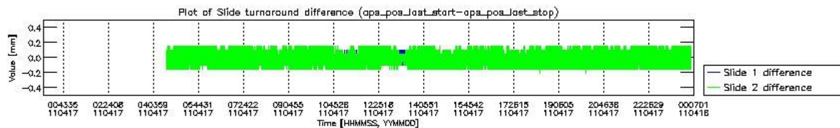
mipas_daily_report_level0_KSPT_L0_4504_N_20110417_5.PNG
