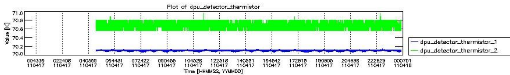
mipas_daily_report_level0_KSPT_L0_4504_N_20110417_3.PNG
