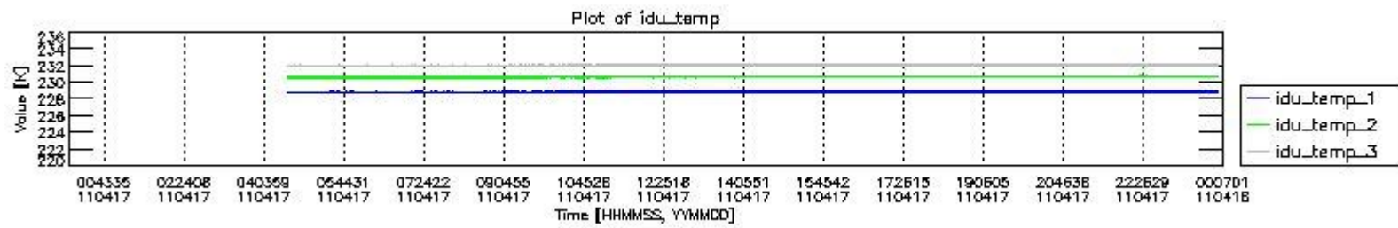
mipas_daily_report_level0_KSPT_L0_4504_N_20110417_2.PNG
