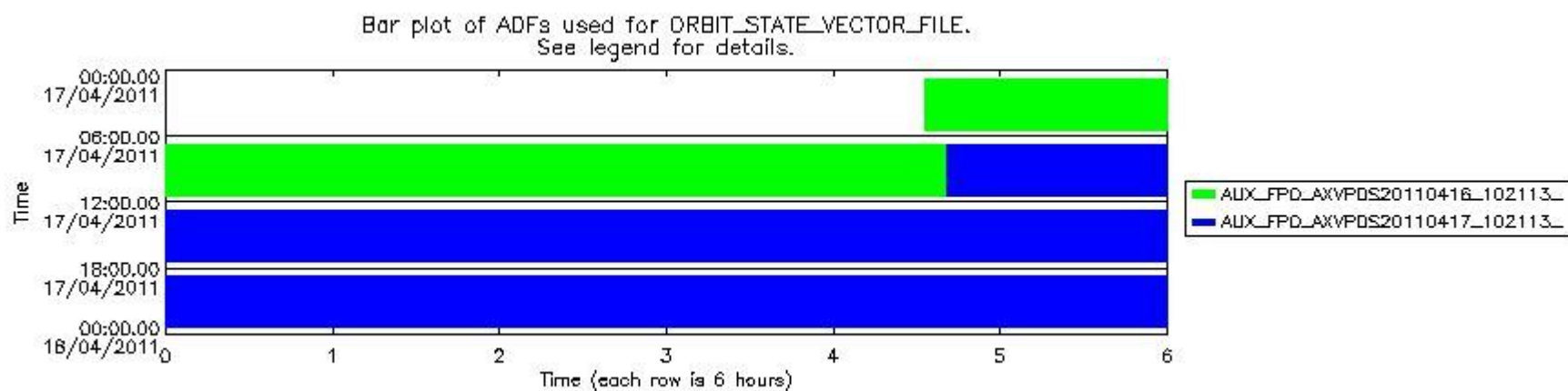
mipas_daily_report_level0_KSPT_L0_4504_N_20110417_13.PNG
