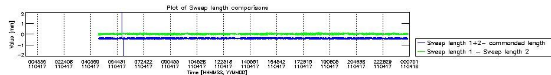
mipas_daily_report_level0_KSPT_L0_4504_N_20110417_8.PNG
