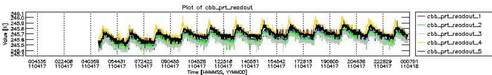
mipas_daily_report_level0_KSPT_L0_4504_N_20110417_9.PNG
