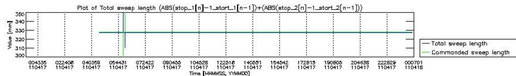
mipas_daily_report_level0_KSPT_L0_4504_N_20110417_6.PNG
