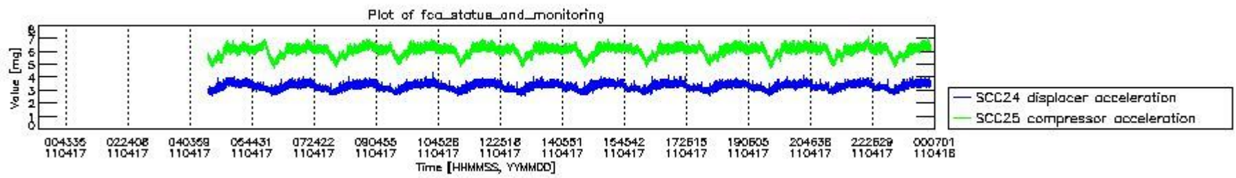
mipas_daily_report_level0_KSPT_L0_4504_N_20110417_10.PNG
