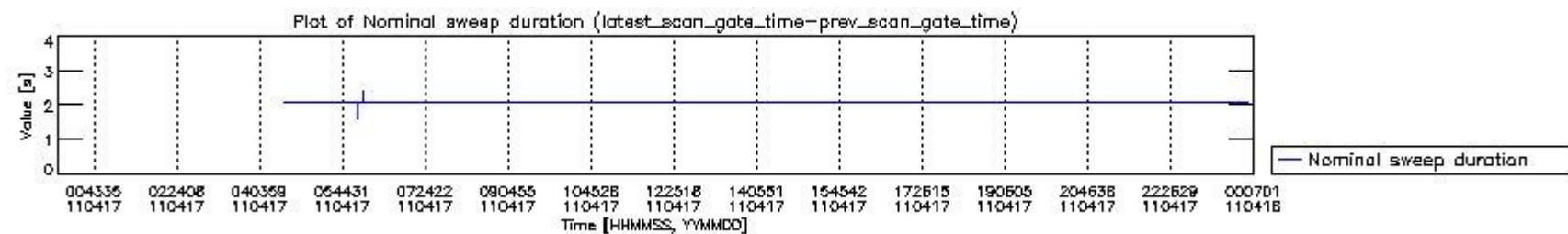
mipas_daily_report_level0_KSPT_L0_4504_N_20110417_3.PNG
