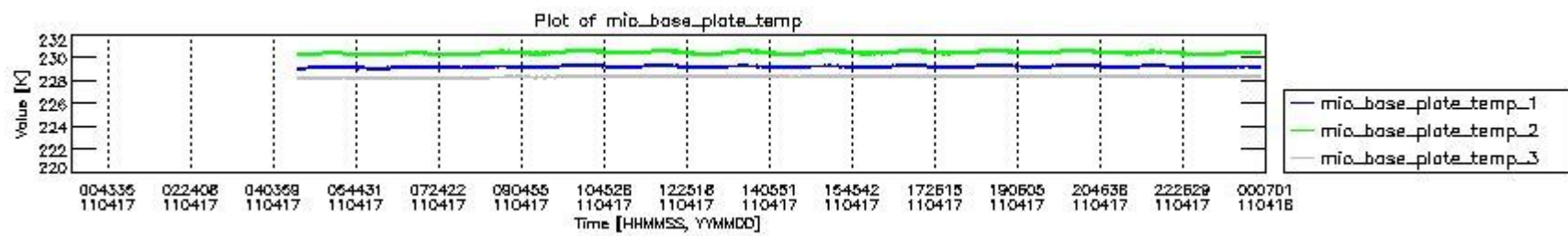
mipas_daily_report_level0_KSPT_L0_4504_N_20110417_1.PNG
