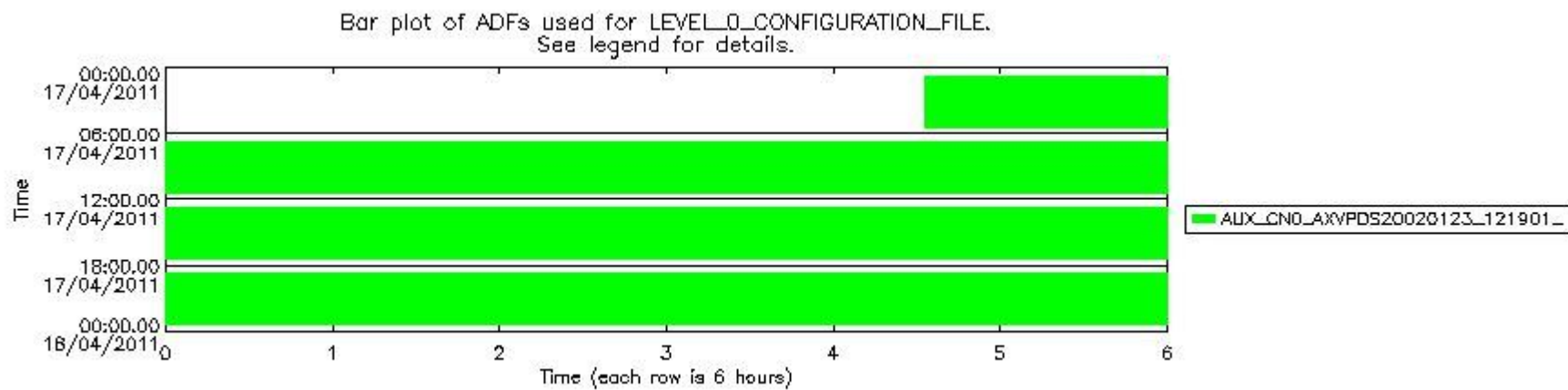
mipas_daily_report_level0_KSPT_L0_4504_N_20110417_12.PNG
