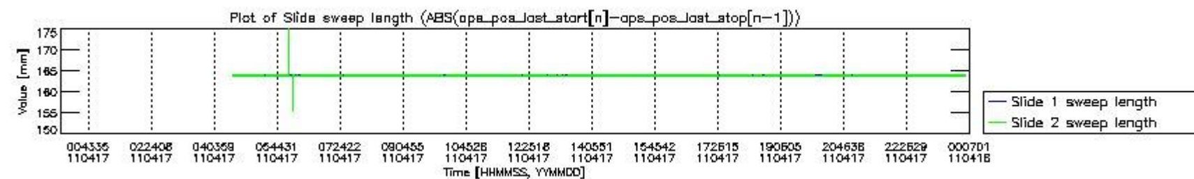
mipas_daily_report_level0_KSPT_L0_4504_N_20110417_7.PNG
