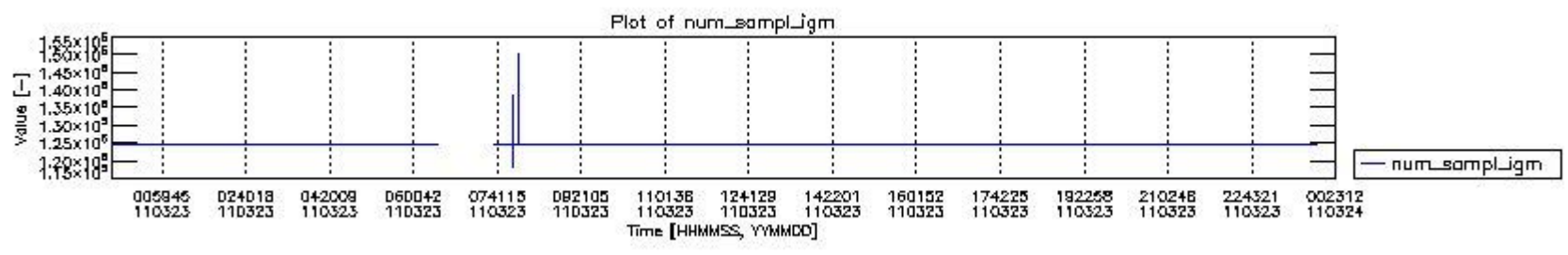
mipas_daily_report_level0_KSPT_L0_4504_N_20110323_0.PNG
