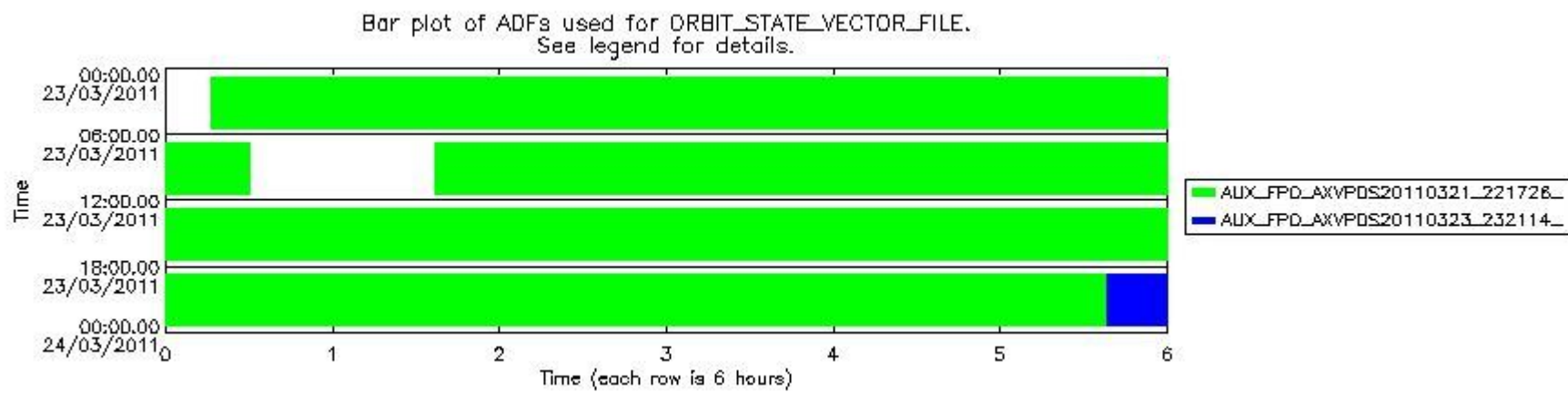
mipas_daily_report_level0_KSPT_L0_4504_N_20110323_13.PNG
