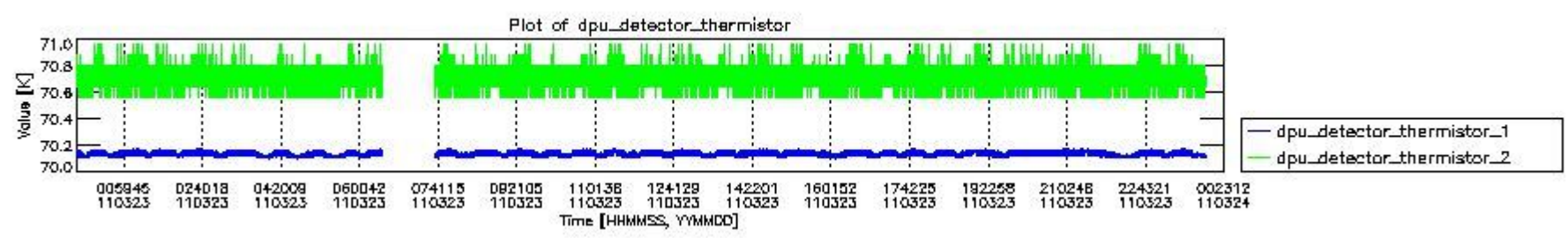
mipas_daily_report_level0_KSPT_L0_4504_N_20110323_3.PNG
