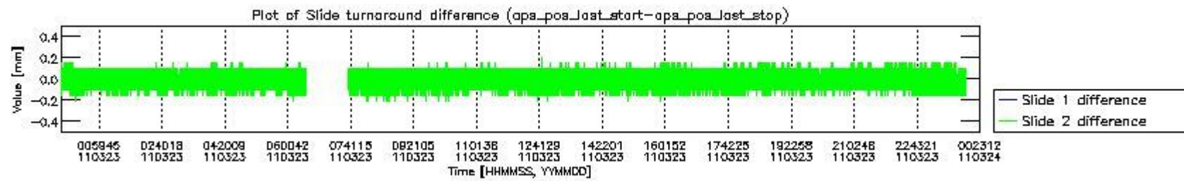
mipas_daily_report_level0_KSPT_L0_4504_N_20110323_5.PNG
