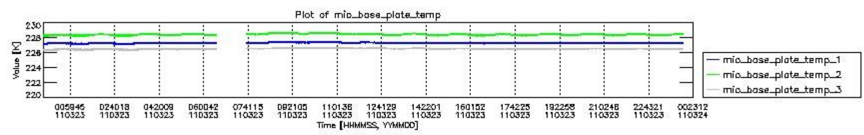
mipas_daily_report_level0_KSPT_L0_4504_N_20110323_1.PNG
