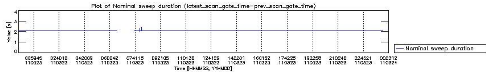
mipas_daily_report_level0_KSPT_L0_4504_N_20110323_4.PNG
