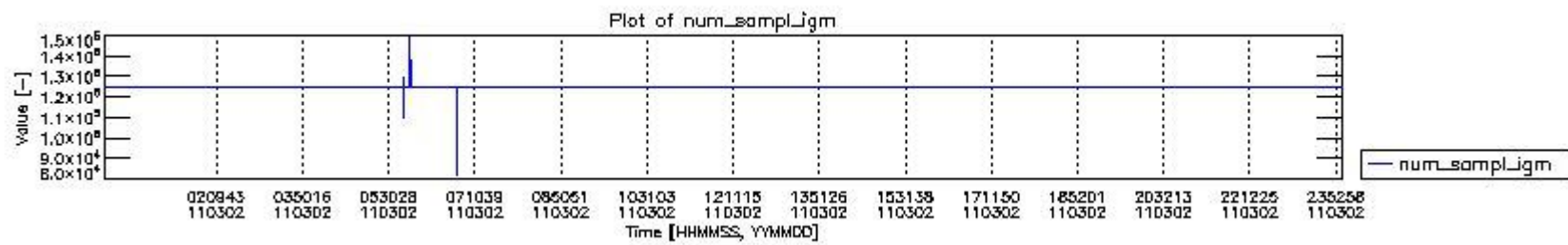
mipas_daily_report_level0_KSPT_L0_4504_N_20110302_0.PNG
