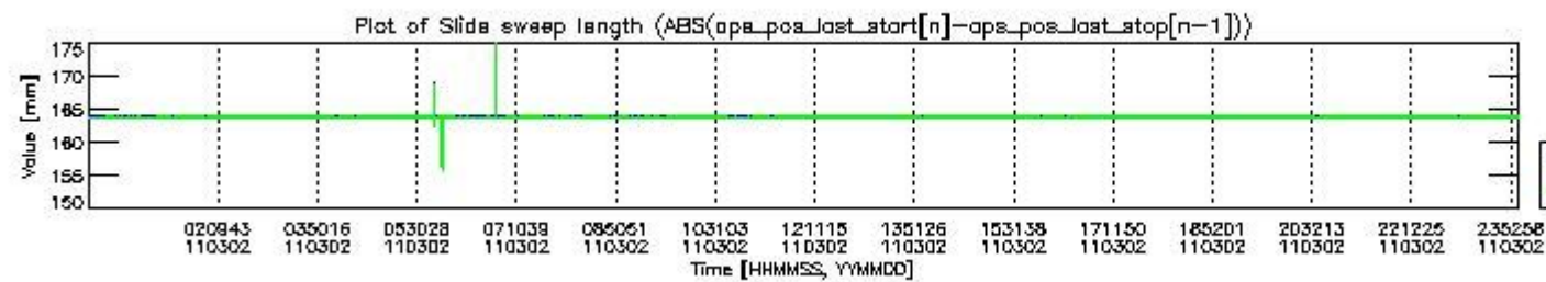
mipas_daily_report_level0_KSPT_L0_4504_N_20110302_7.PNG
