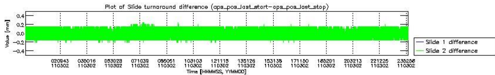
mipas_daily_report_level0_KSPT_L0_4504_N_20110302_5.PNG
