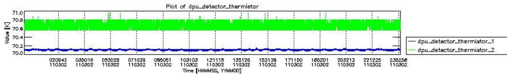
mipas_daily_report_level0_KSPT_L0_4504_N_20110302_3.PNG
