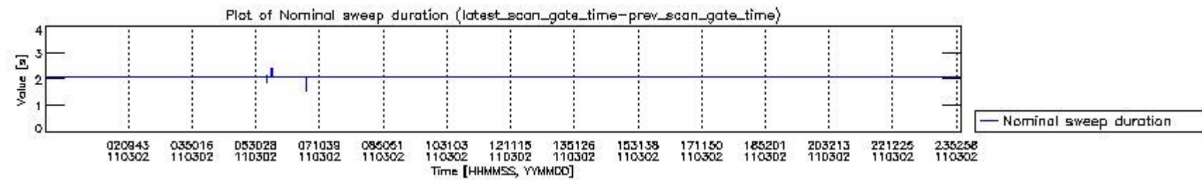
mipas_daily_report_level0_KSPT_L0_4504_N_20110302_4.PNG
