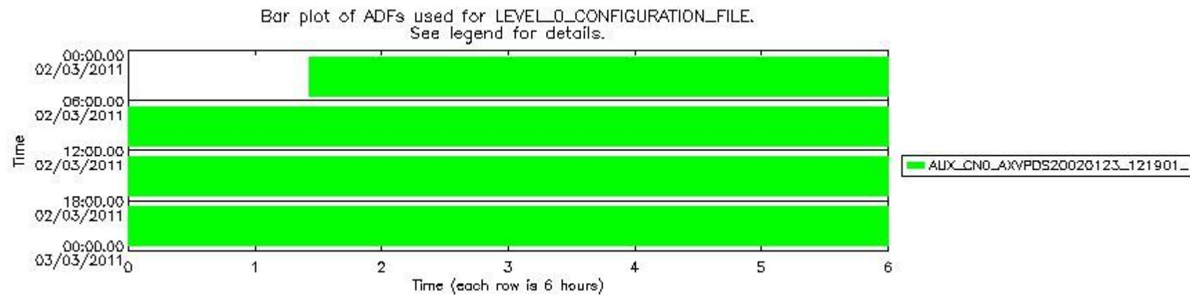
mipas_daily_report_level0_KSPT_L0_4504_N_20110302_12.PNG
