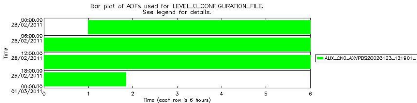
mipas_daily_report_level0_KSPT_L0_4504_N_20110228_12.PNG
