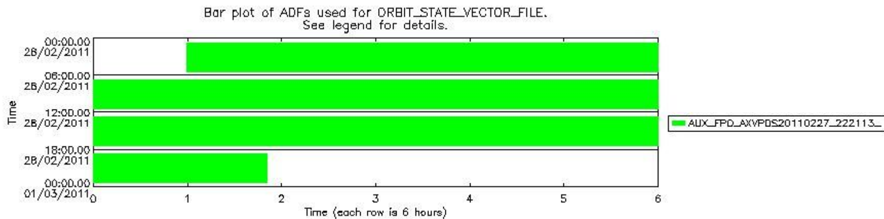
mipas_daily_report_level0_KSPT_L0_4504_N_20110228_13.PNG
