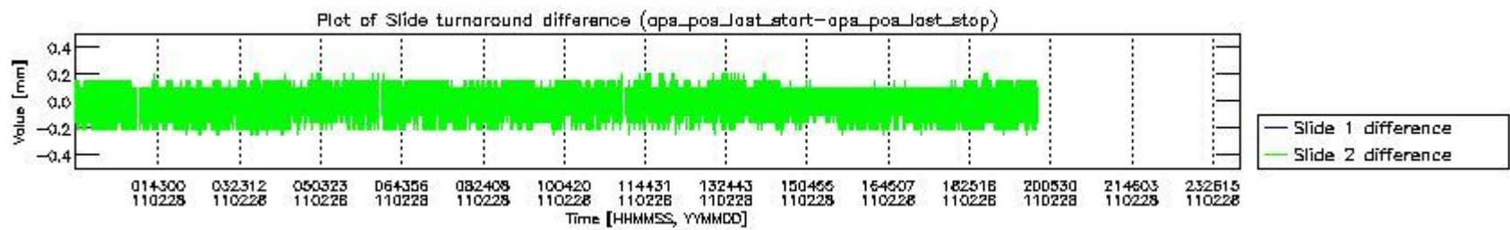
mipas_daily_report_level0_KSPT_L0_4504_N_20110228_5.PNG
