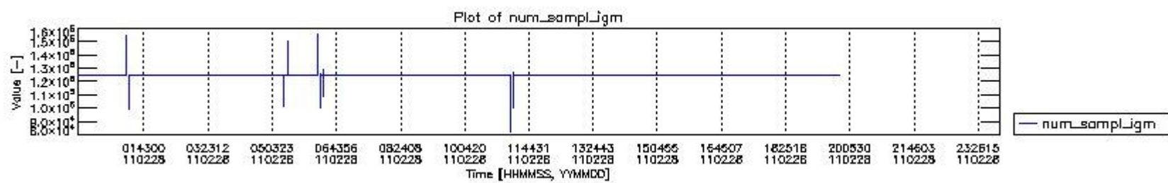
mipas_daily_report_level0_KSPT_L0_4504_N_20110228_0.PNG
