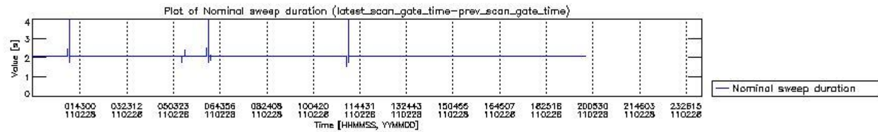
mipas_daily_report_level0_KSPT_L0_4504_N_20110228_4.PNG
