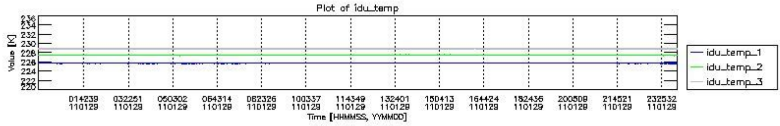
mipas_daily_report_level0_KSPT_L0_4504_N_20110129_2.PNG
