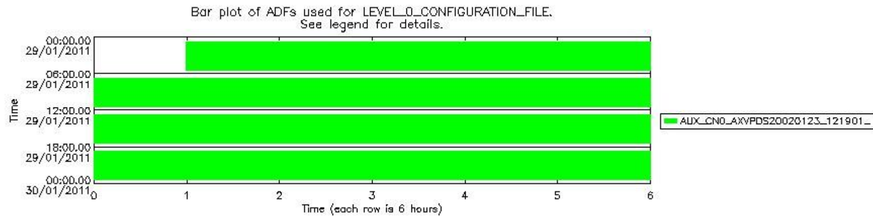
mipas_daily_report_level0_KSPT_L0_4504_N_20110129_12.PNG
