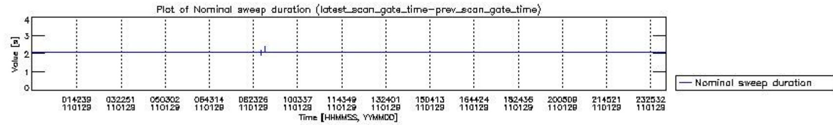
mipas_daily_report_level0_KSPT_L0_4504_N_20110129_4.PNG
