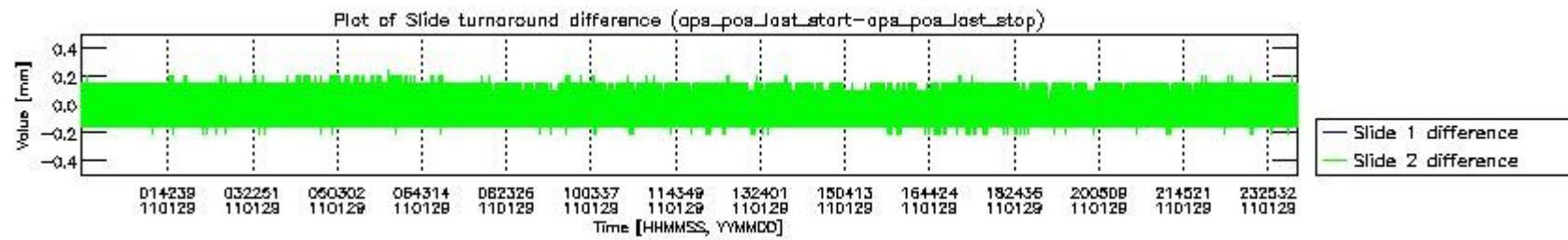
mipas_daily_report_level0_KSPT_L0_4504_N_20110129_5.PNG
