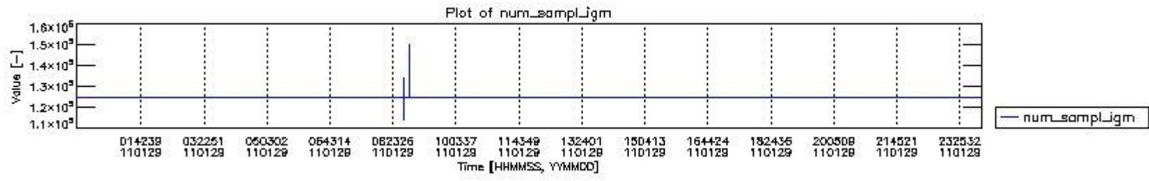
mipas_daily_report_level0_KSPT_L0_4504_N_20110129_0.PNG
