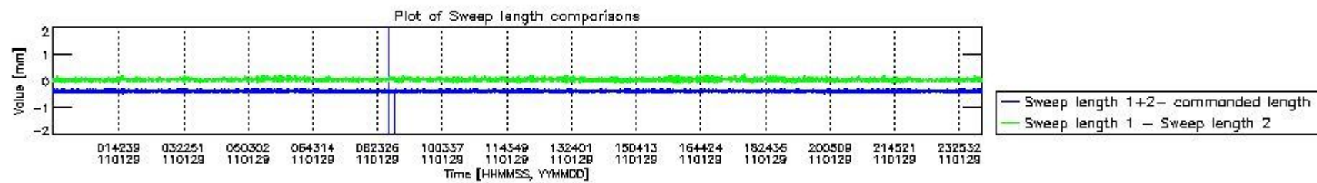
mipas_daily_report_level0_KSPT_L0_4504_N_20110129_8.PNG
