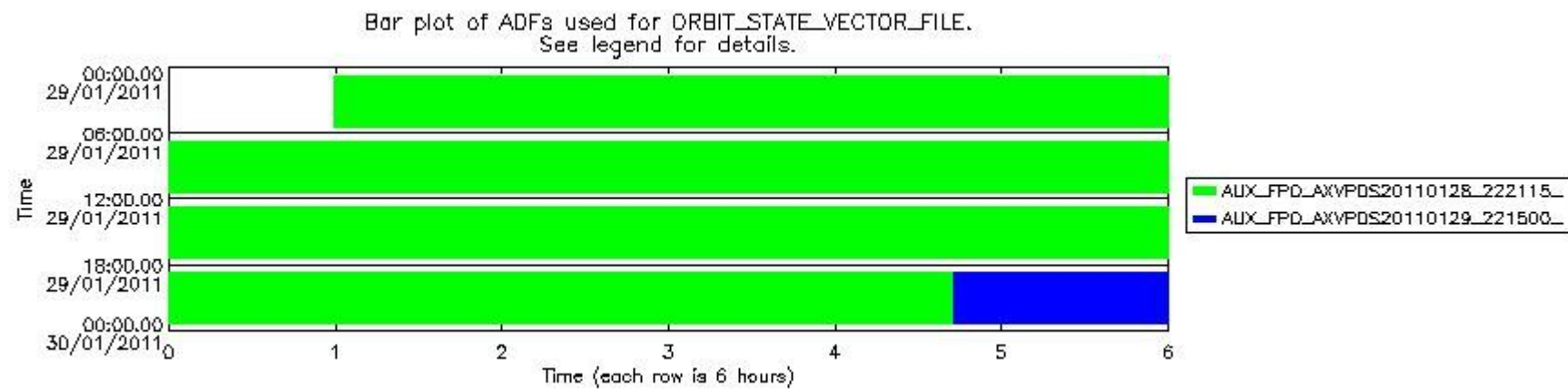
mipas_daily_report_level0_KSPT_L0_4504_N_20110129_13.PNG
