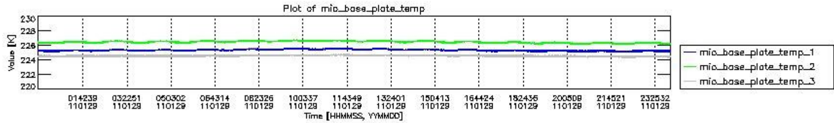
mipas_daily_report_level0_KSPT_L0_4504_N_20110129_1.PNG
