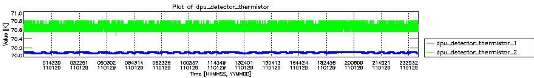
mipas_daily_report_level0_KSPT_L0_4504_N_20110129_3.PNG
