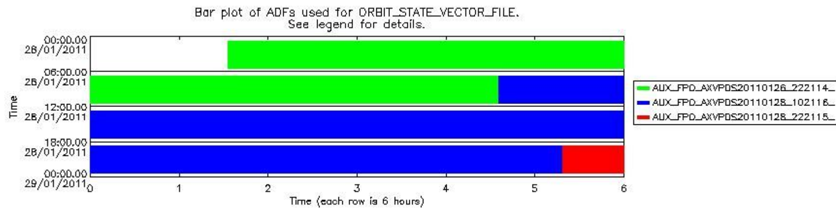
mipas_daily_report_level0_KSPT_L0_4504_N_20110128_13.PNG
