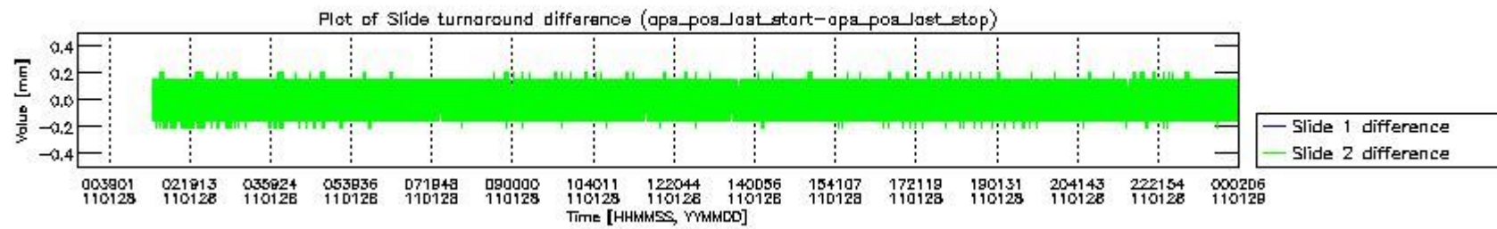
mipas_daily_report_level0_KSPT_L0_4504_N_20110128_5.PNG
