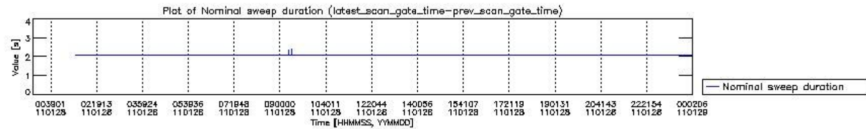
mipas_daily_report_level0_KSPT_L0_4504_N_20110128_4.PNG
