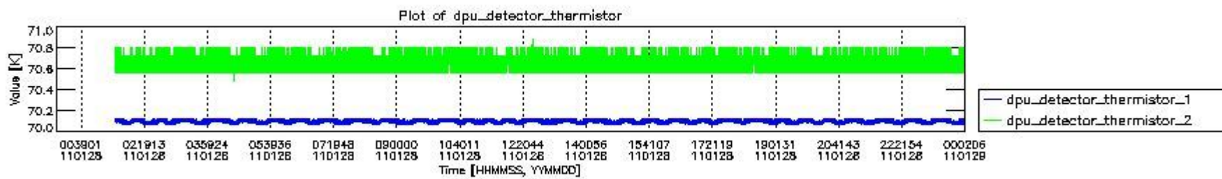
mipas_daily_report_level0_KSPT_L0_4504_N_20110128_3.PNG
