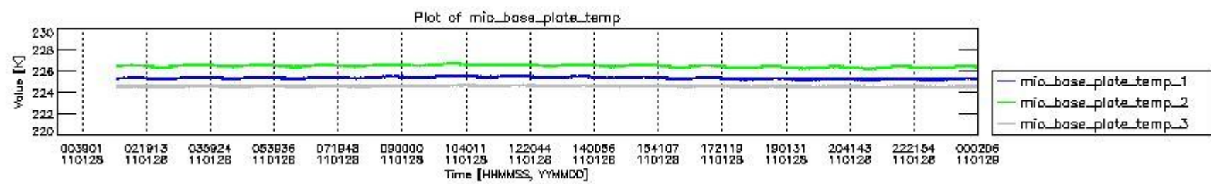
mipas_daily_report_level0_KSPT_L0_4504_N_20110128_1.PNG
