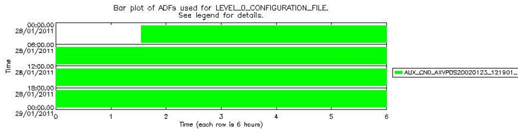
mipas_daily_report_level0_KSPT_L0_4504_N_20110128_12.PNG
