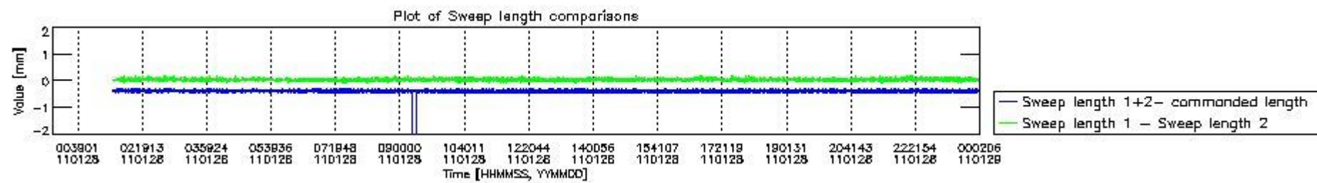
mipas_daily_report_level0_KSPT_L0_4504_N_20110128_8.PNG
