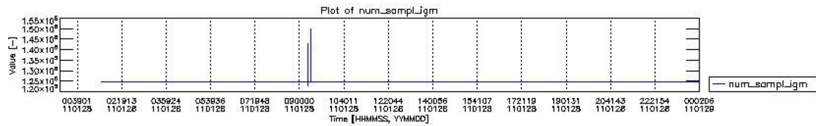
mipas_daily_report_level0_KSPT_L0_4504_N_20110128_0.PNG
