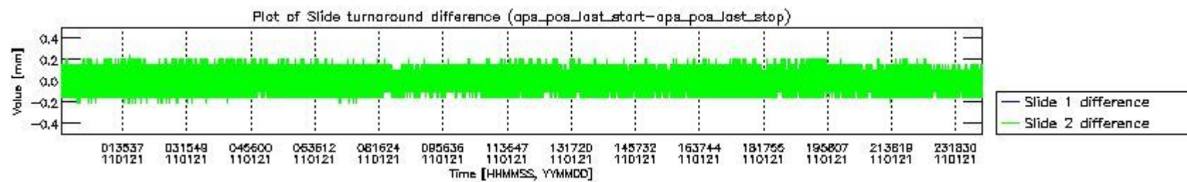
mipas_daily_report_level0_KSPT_L0_4504_N_20110121_5.PNG
