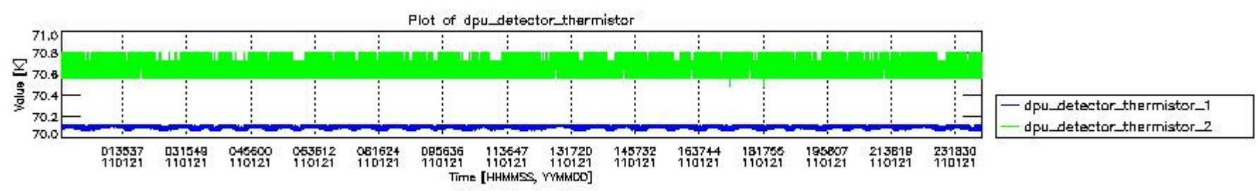
mipas_daily_report_level0_KSPT_L0_4504_N_20110121_3.PNG
