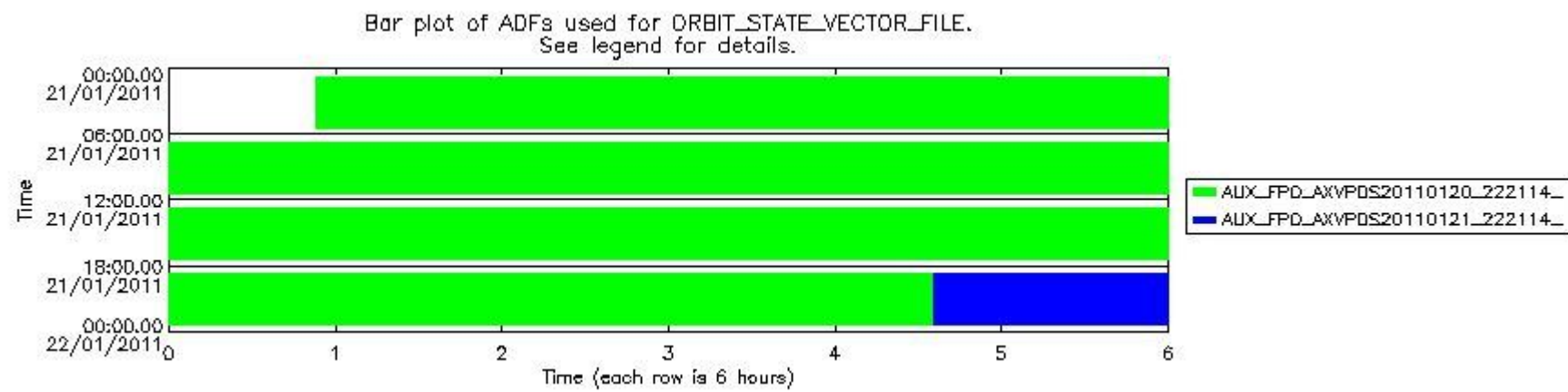
mipas_daily_report_level0_KSPT_L0_4504_N_20110121_13.PNG
