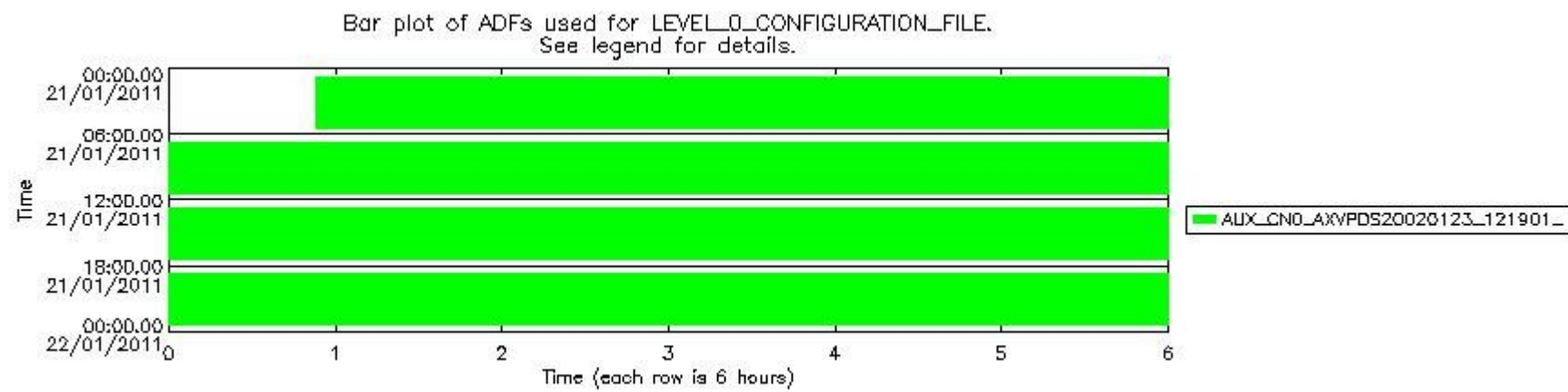
mipas_daily_report_level0_KSPT_L0_4504_N_20110121_12.PNG
