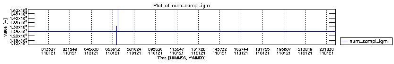
mipas_daily_report_level0_KSPT_L0_4504_N_20110121_0.PNG
