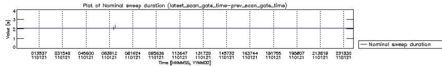
mipas_daily_report_level0_KSPT_L0_4504_N_20110121_4.PNG
