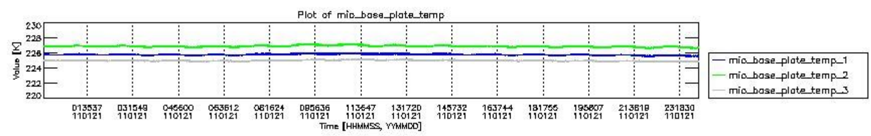
mipas_daily_report_level0_KSPT_L0_4504_N_20110121_1.PNG
