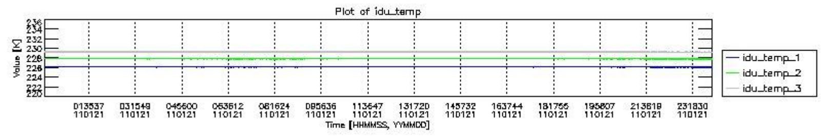
mipas_daily_report_level0_KSPT_L0_4504_N_20110121_2.PNG
