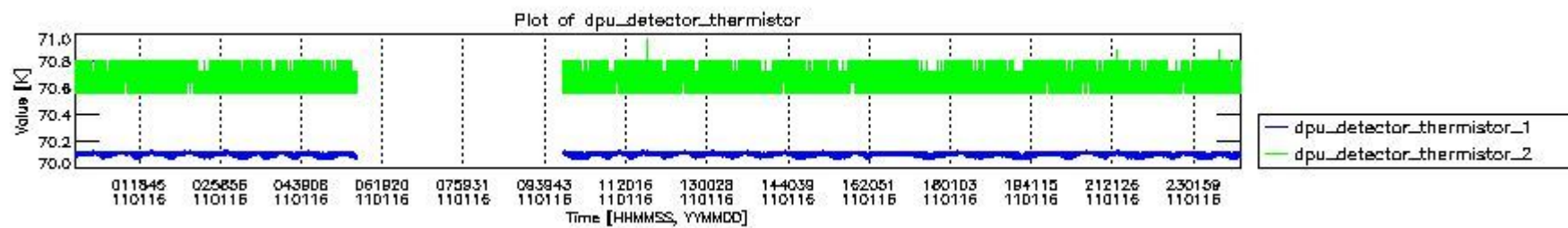
mipas_daily_report_level0_KSPT_L0_4504_N_20110116_3.PNG
