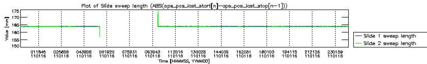
mipas_daily_report_level0_KSPT_L0_4504_N_20110116_7.PNG
