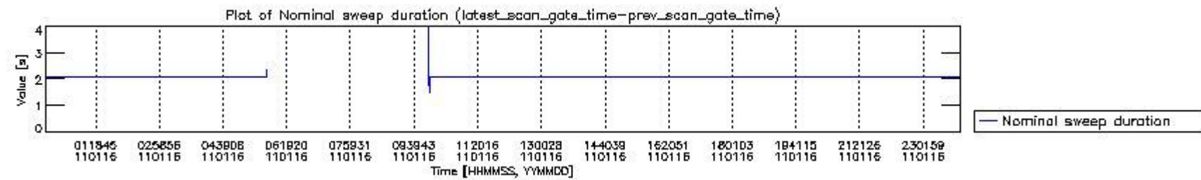
mipas_daily_report_level0_KSPT_L0_4504_N_20110116_4.PNG
