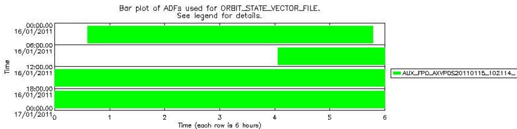
mipas_daily_report_level0_KSPT_L0_4504_N_20110116_13.PNG
