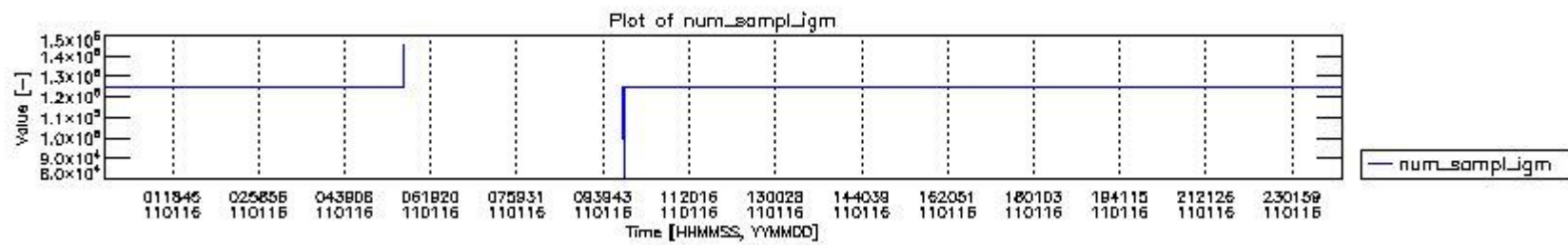
mipas_daily_report_level0_KSPT_L0_4504_N_20110116_0.PNG
