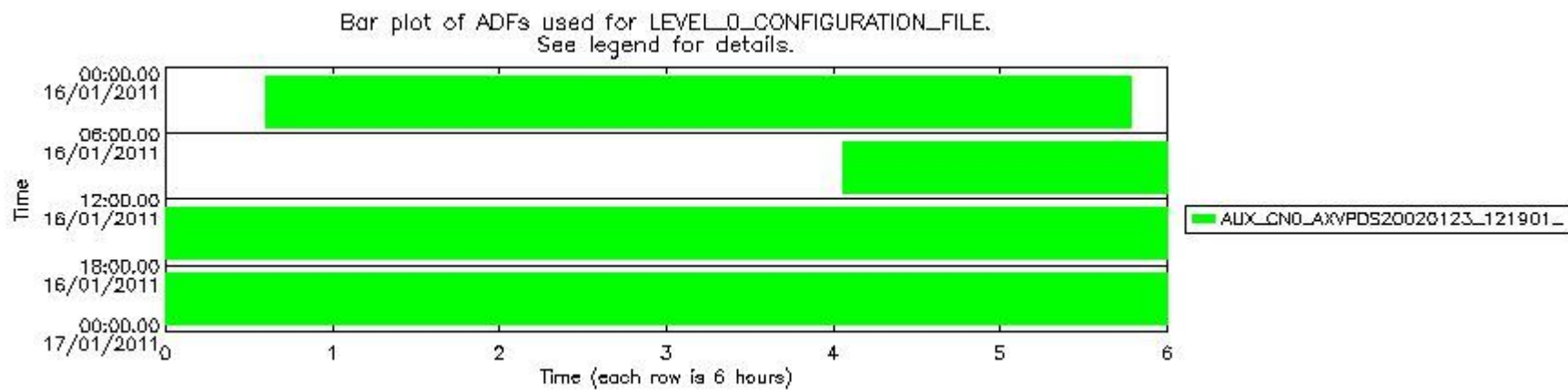
mipas_daily_report_level0_KSPT_L0_4504_N_20110116_12.PNG
