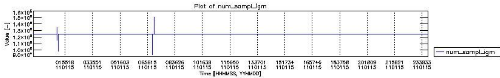
mipas_daily_report_level0_KSPT_L0_4504_N_20110115_0.PNG
