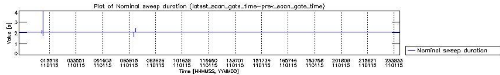
mipas_daily_report_level0_KSPT_L0_4504_N_20110115_4.PNG
