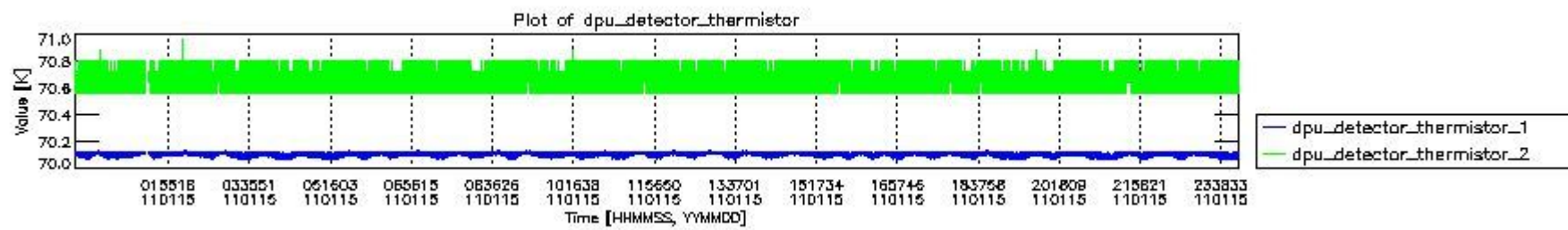
mipas_daily_report_level0_KSPT_L0_4504_N_20110115_3.PNG
