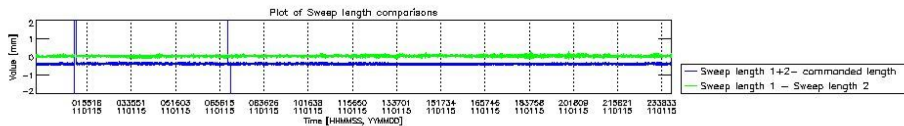
mipas_daily_report_level0_KSPT_L0_4504_N_20110115_8.PNG
