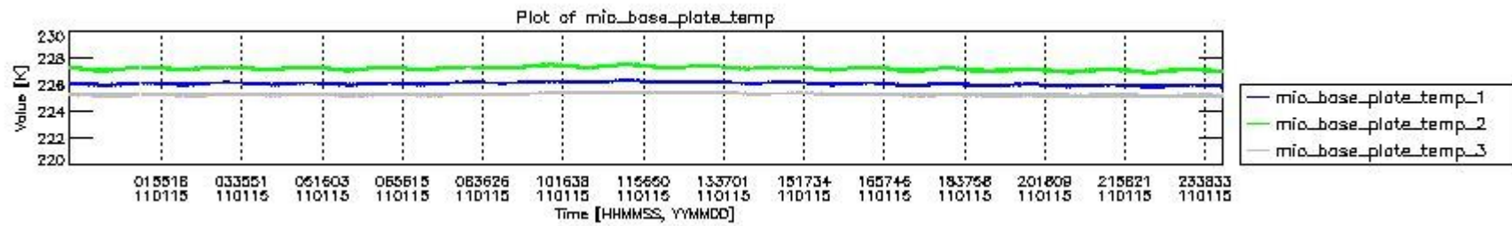
mipas_daily_report_level0_KSPT_L0_4504_N_20110115_1.PNG
