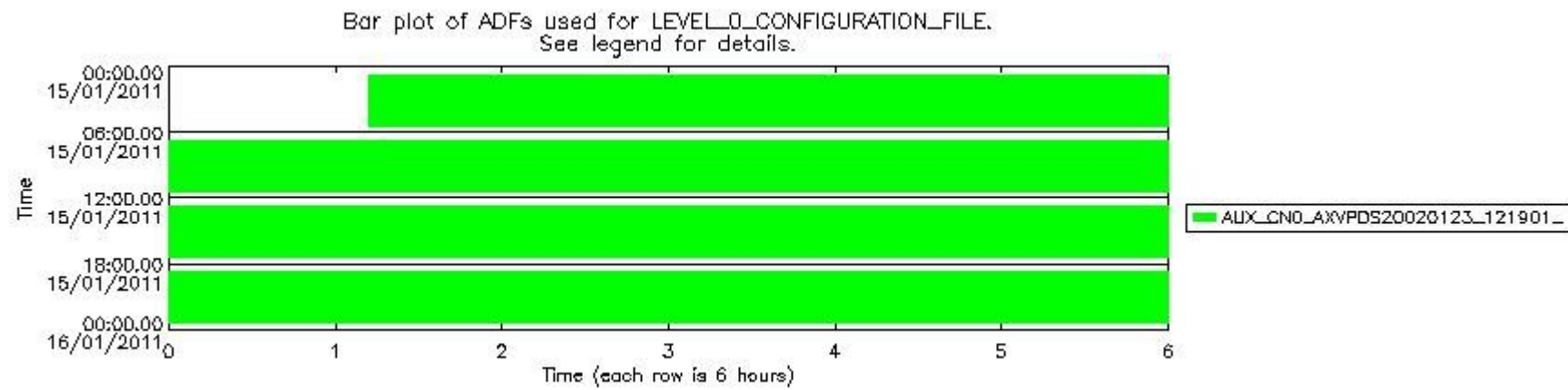
mipas_daily_report_level0_KSPT_L0_4504_N_20110115_12.PNG
