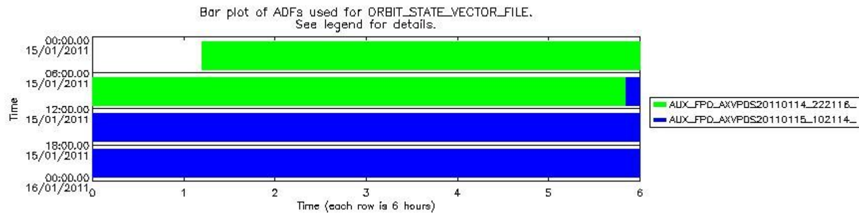
mipas_daily_report_level0_KSPT_L0_4504_N_20110115_13.PNG
