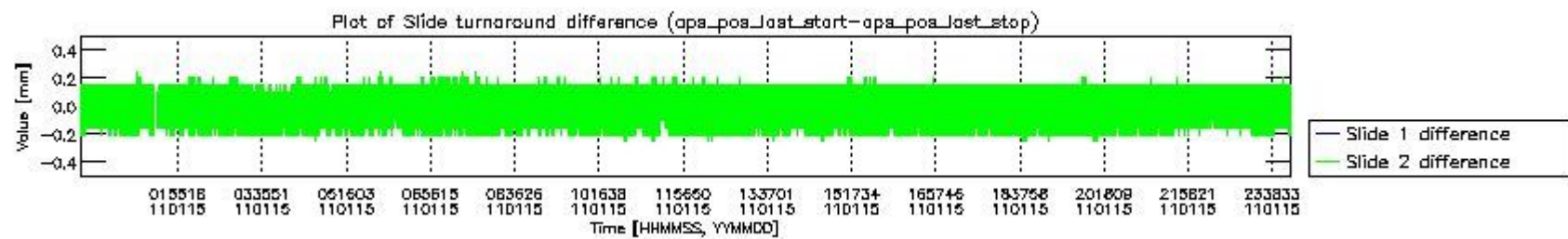
mipas_daily_report_level0_KSPT_L0_4504_N_20110115_5.PNG
