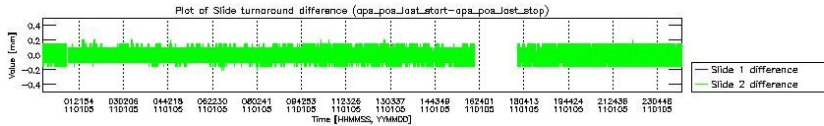
mipas_daily_report_level0_KSPT_L0_4504_N_20110105_5.PNG
