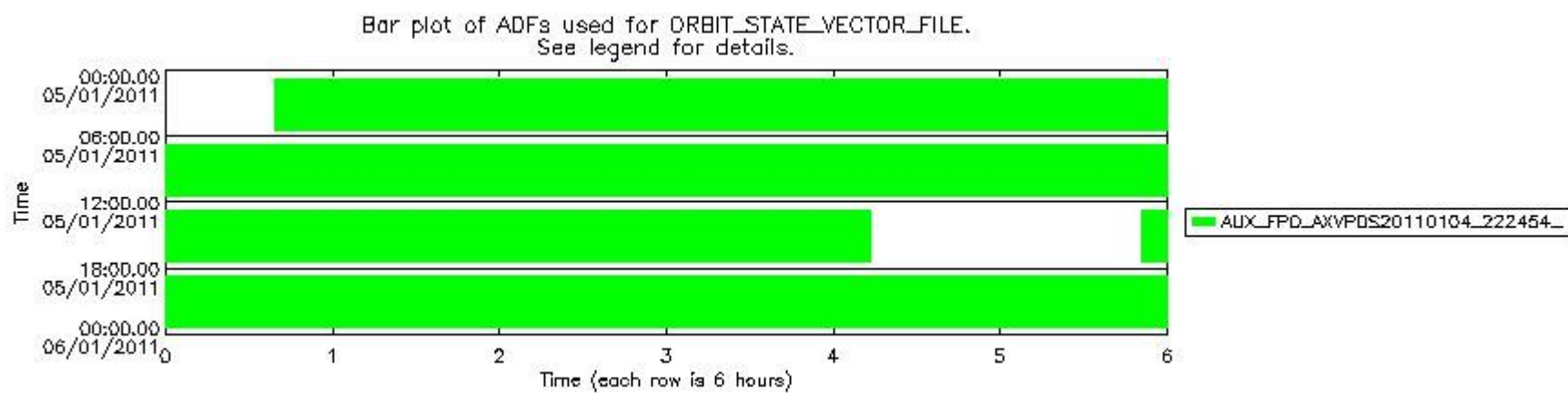
mipas_daily_report_level0_KSPT_L0_4504_N_20110105_13.PNG
