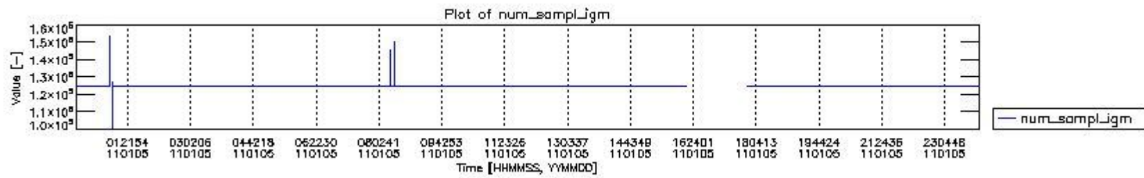
mipas_daily_report_level0_KSPT_L0_4504_N_20110105_0.PNG
