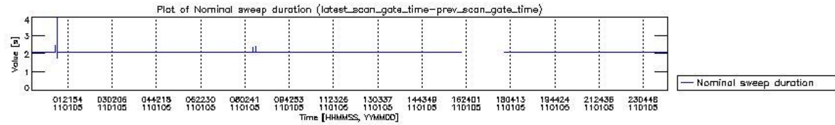
mipas_daily_report_level0_KSPT_L0_4504_N_20110105_4.PNG
