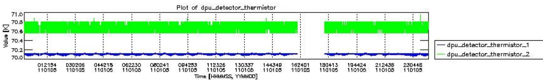
mipas_daily_report_level0_KSPT_L0_4504_N_20110105_3.PNG
