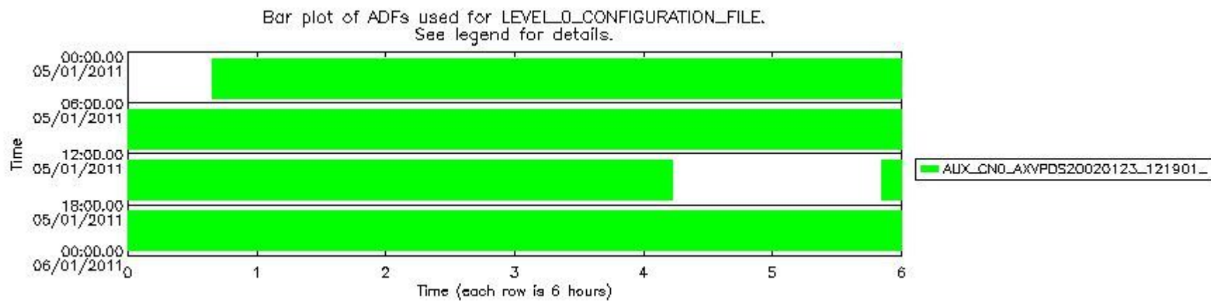
mipas_daily_report_level0_KSPT_L0_4504_N_20110105_12.PNG
