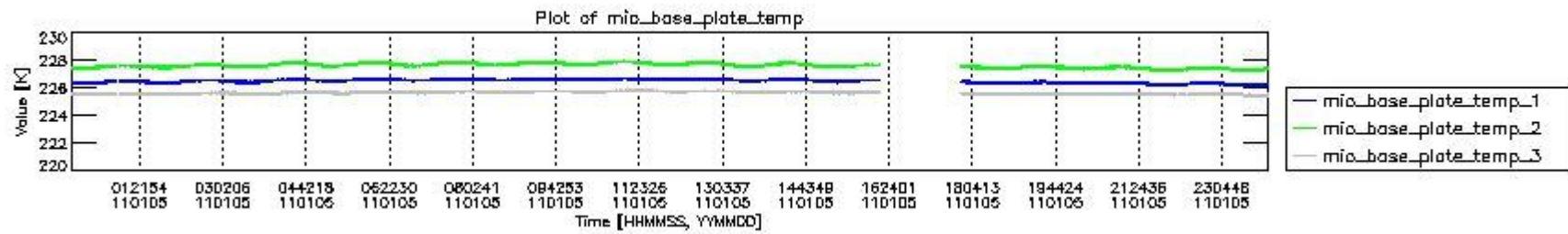
mipas_daily_report_level0_KSPT_L0_4504_N_20110105_1.PNG
