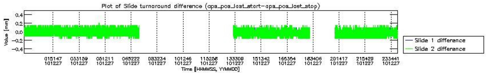
mipas_daily_report_level0_KSPT_L0_4504_N_20101227_5.PNG
