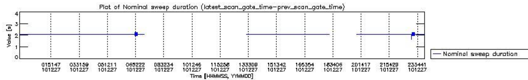
mipas_daily_report_level0_KSPT_L0_4504_N_20101227_4.PNG
