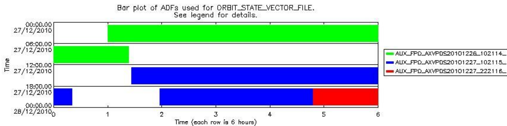
mipas_daily_report_level0_KSPT_L0_4504_N_20101227_12.PNG
