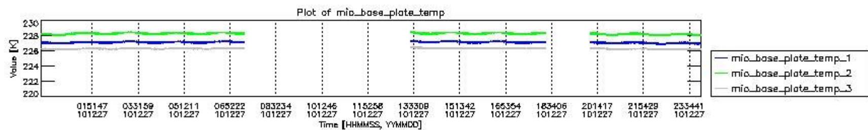
mipas_daily_report_level0_KSPT_L0_4504_N_20101227_1.PNG
