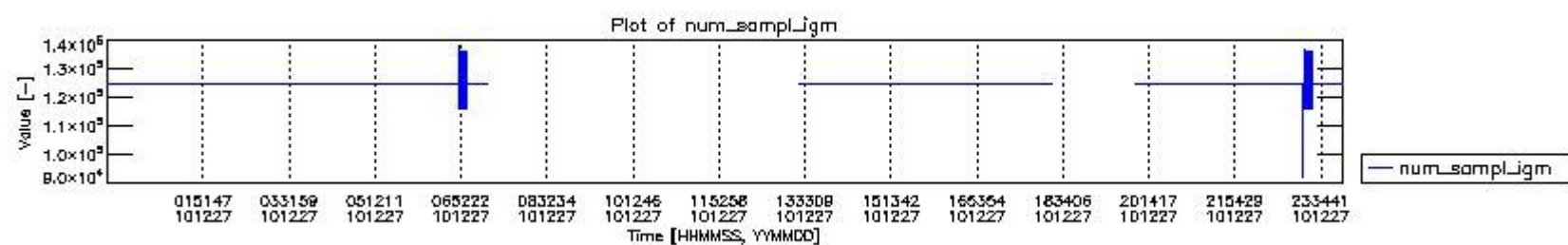
mipas_daily_report_level0_KSPT_L0_4504_N_20101227_0.PNG
