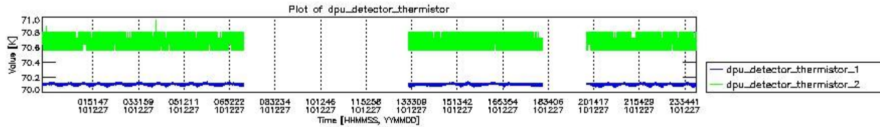
mipas_daily_report_level0_KSPT_L0_4504_N_20101227_3.PNG
