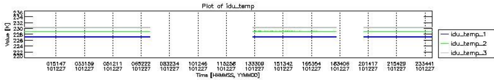
mipas_daily_report_level0_KSPT_L0_4504_N_20101227_2.PNG
