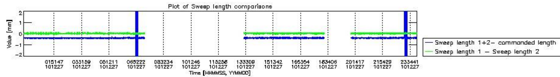
mipas_daily_report_level0_KSPT_L0_4504_N_20101227_8.PNG
