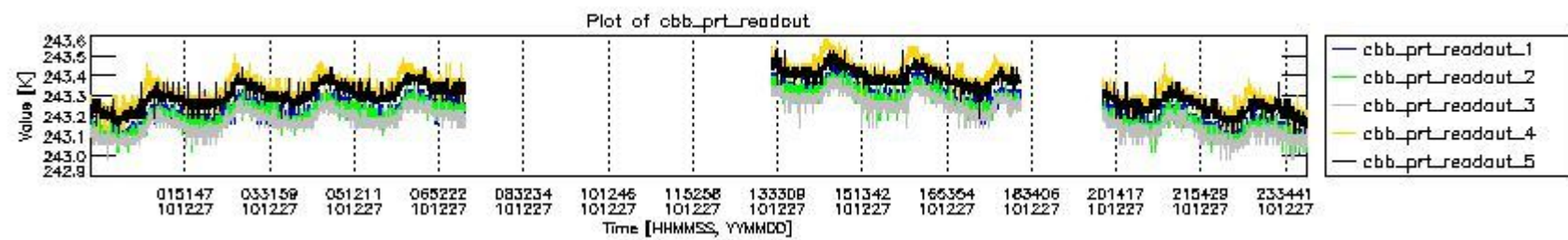
mipas_daily_report_level0_KSPT_L0_4504_N_20101227_9.PNG
