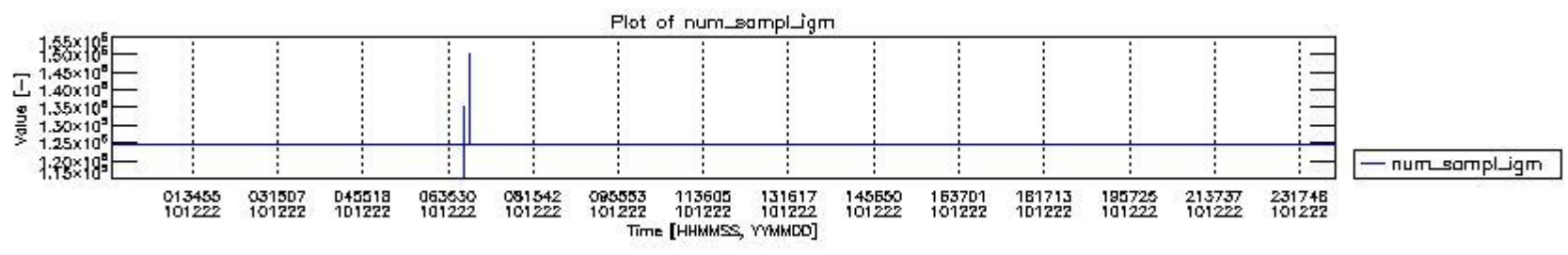
mipas_daily_report_level0_KSPT_L0_4504_N_20101222_0.PNG
