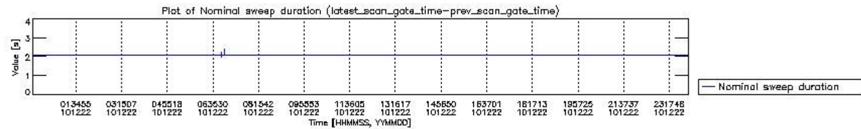
mipas_daily_report_level0_KSPT_L0_4504_N_20101222_4.PNG
