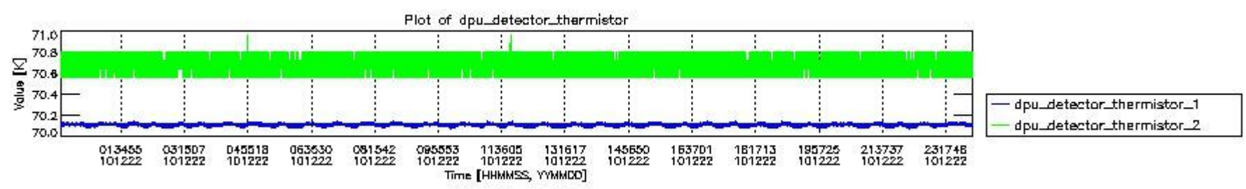
mipas_daily_report_level0_KSPT_L0_4504_N_20101222_3.PNG
