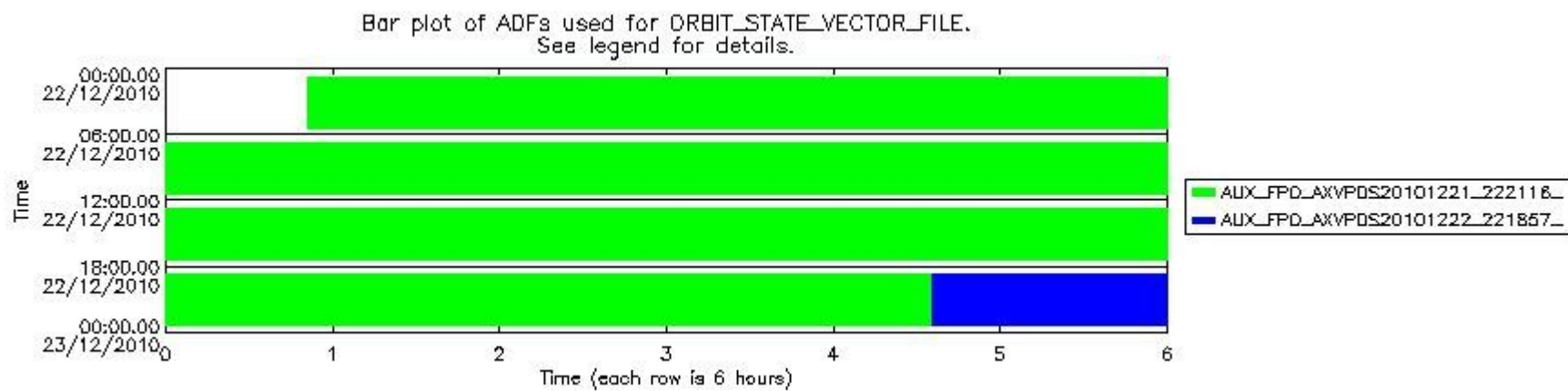
mipas_daily_report_level0_KSPT_L0_4504_N_20101222_13.PNG
