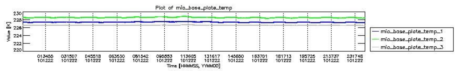
mipas_daily_report_level0_KSPT_L0_4504_N_20101222_1.PNG
