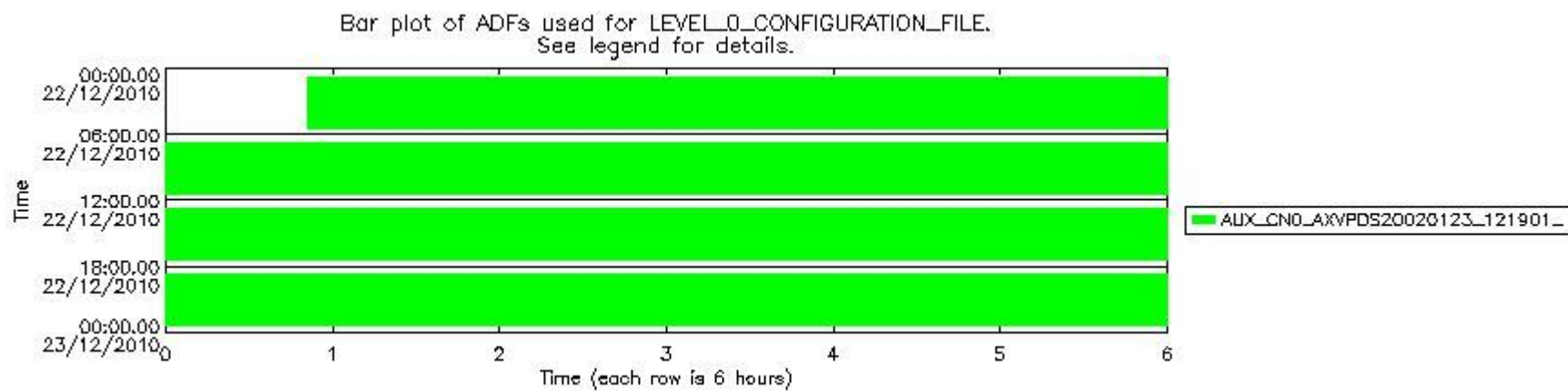
mipas_daily_report_level0_KSPT_L0_4504_N_20101222_12.PNG
