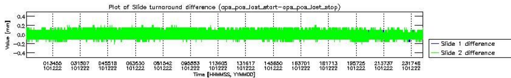
mipas_daily_report_level0_KSPT_L0_4504_N_20101222_5.PNG
