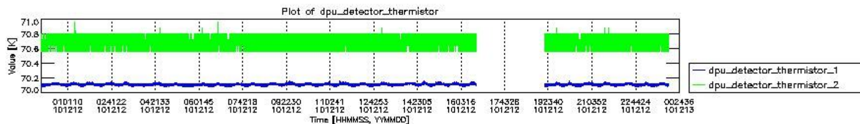
mipas_daily_report_level0_KSPT_L0_4504_N_20101212_3.PNG
