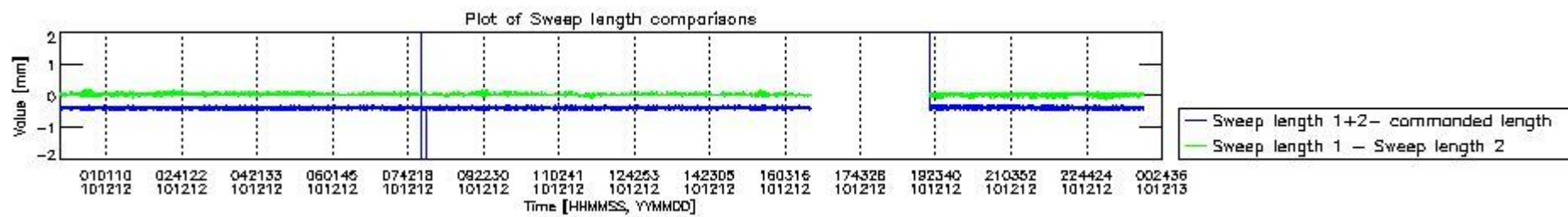
mipas_daily_report_level0_KSPT_L0_4504_N_20101212_8.PNG
