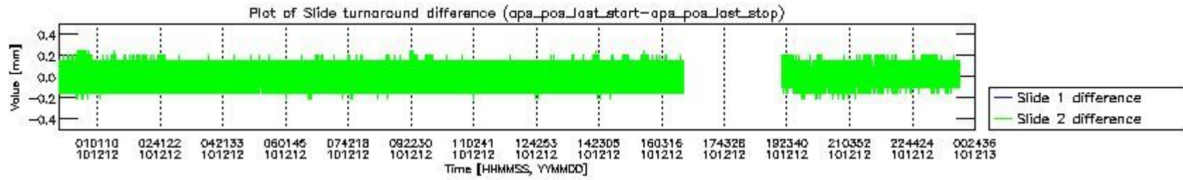
mipas_daily_report_level0_KSPT_L0_4504_N_20101212_5.PNG
