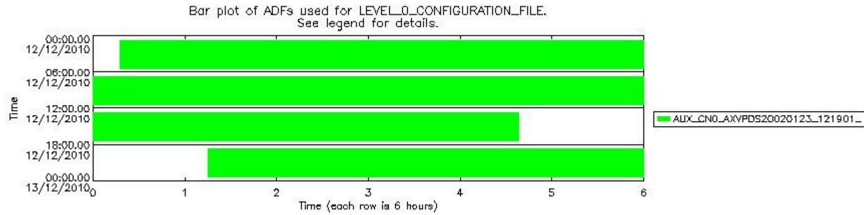
mipas_daily_report_level0_KSPT_L0_4504_N_20101212_12.PNG
