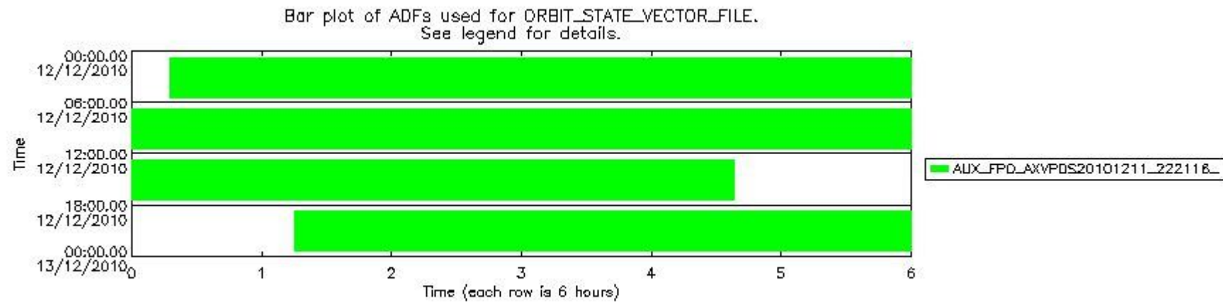
mipas_daily_report_level0_KSPT_L0_4504_N_20101212_13.PNG
