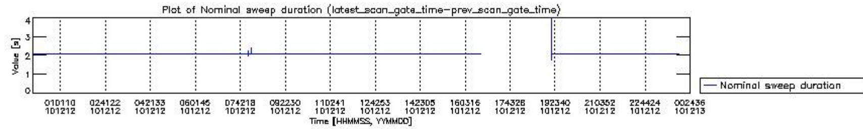
mipas_daily_report_level0_KSPT_L0_4504_N_20101212_4.PNG
