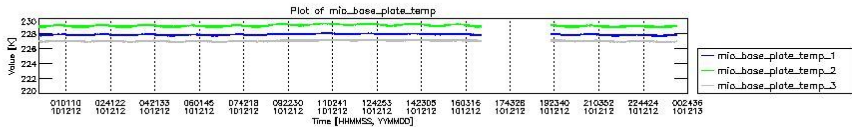
mipas_daily_report_level0_KSPT_L0_4504_N_20101212_1.PNG
