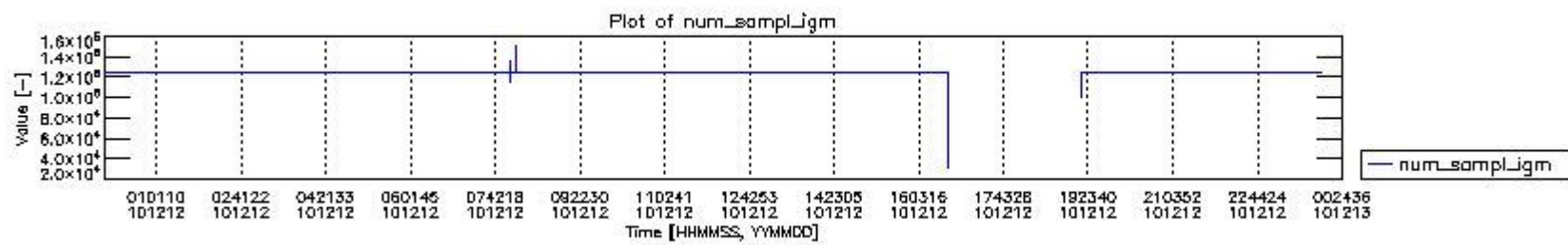
mipas_daily_report_level0_KSPT_L0_4504_N_20101212_0.PNG
