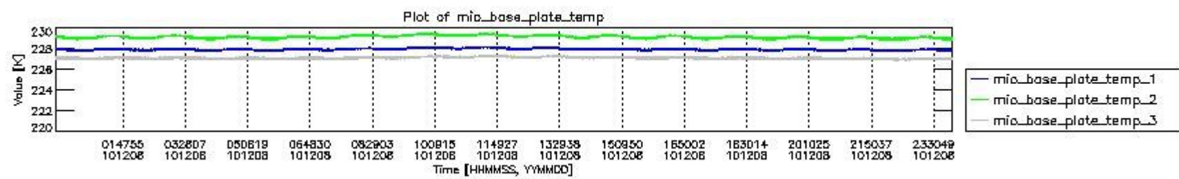
mipas_daily_report_level0_KSPT_L0_4504_N_20101208_1.PNG
