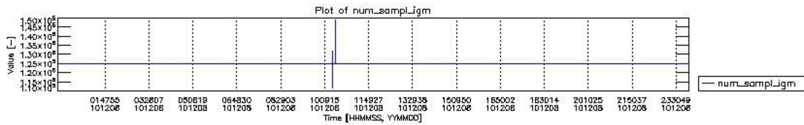
mipas_daily_report_level0_KSPT_L0_4504_N_20101208_0.PNG
