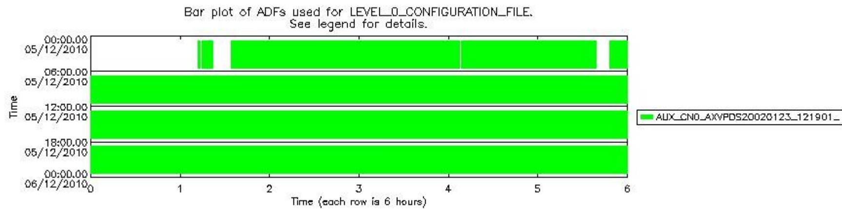
mipas_daily_report_level0_KSPT_L0_4504_N_20101205_12.PNG
