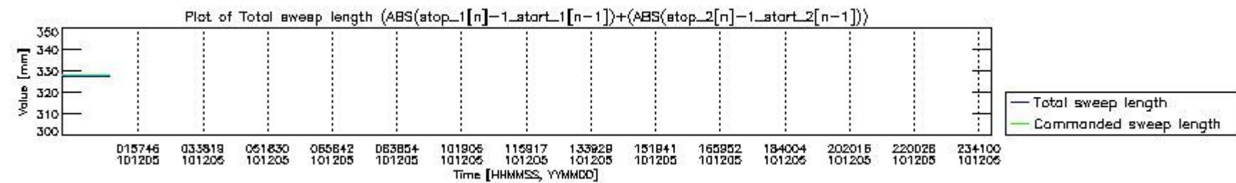
mipas_daily_report_level0_KSPT_L0_4504_N_20101205_6.PNG
