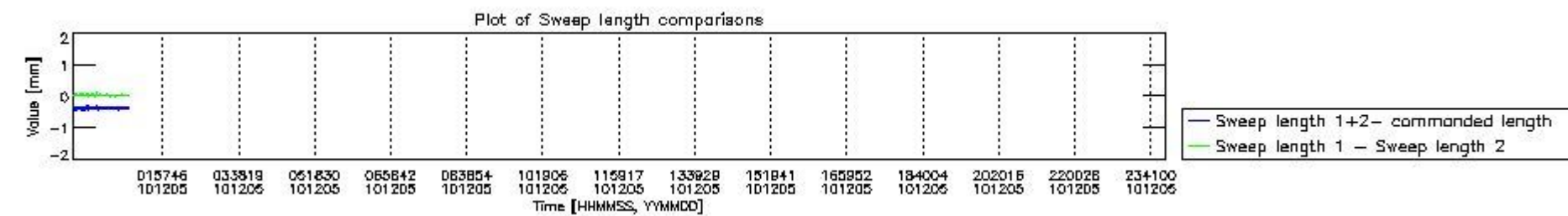
mipas_daily_report_level0_KSPT_L0_4504_N_20101205_8.PNG
