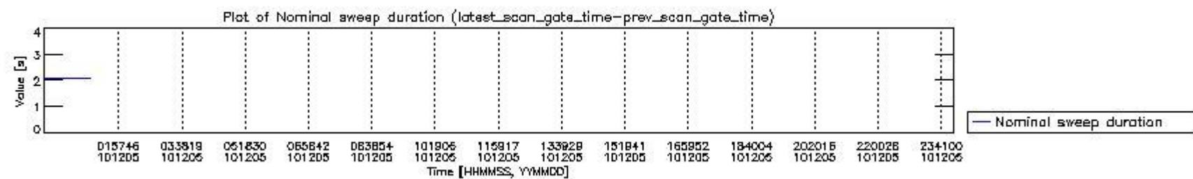
mipas_daily_report_level0_KSPT_L0_4504_N_20101205_4.PNG
