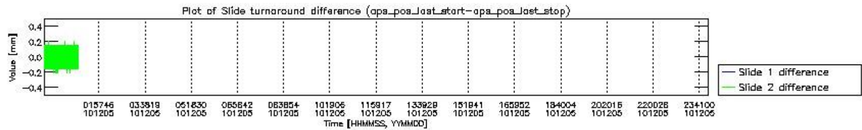
mipas_daily_report_level0_KSPT_L0_4504_N_20101205_5.PNG
