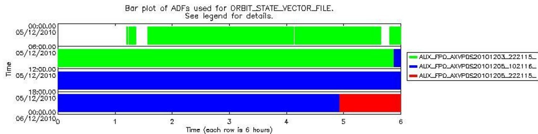
mipas_daily_report_level0_KSPT_L0_4504_N_20101205_13.PNG
