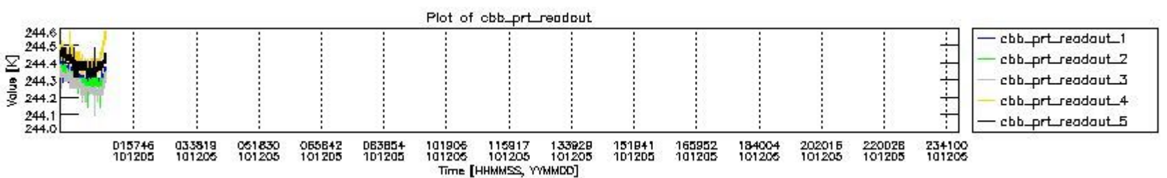
mipas_daily_report_level0_KSPT_L0_4504_N_20101205_9.PNG
