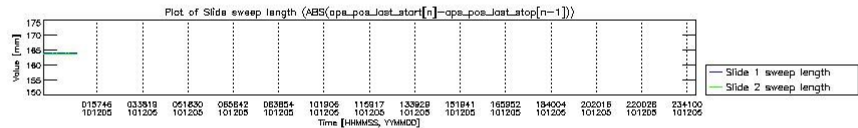
mipas_daily_report_level0_KSPT_L0_4504_N_20101205_7.PNG
