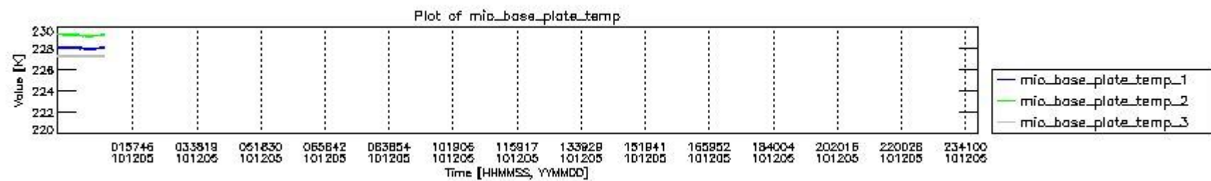
mipas_daily_report_level0_KSPT_L0_4504_N_20101205_1.PNG
