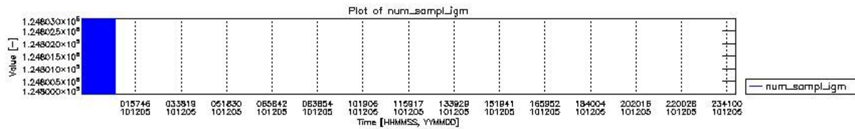
mipas_daily_report_level0_KSPT_L0_4504_N_20101205_0.PNG
