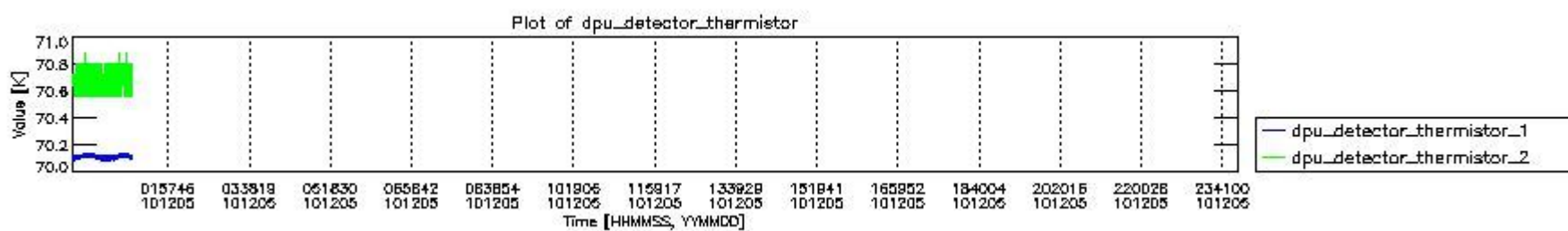
mipas_daily_report_level0_KSPT_L0_4504_N_20101205_3.PNG
