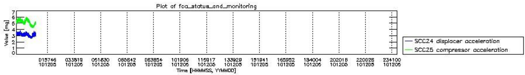
mipas_daily_report_level0_KSPT_L0_4504_N_20101205_10.PNG
