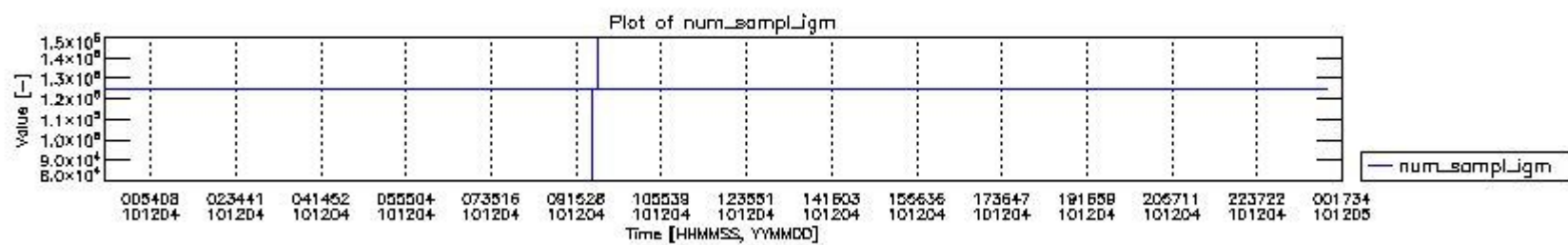
mipas_daily_report_level0_KSPT_L0_4504_N_20101204_0.PNG
