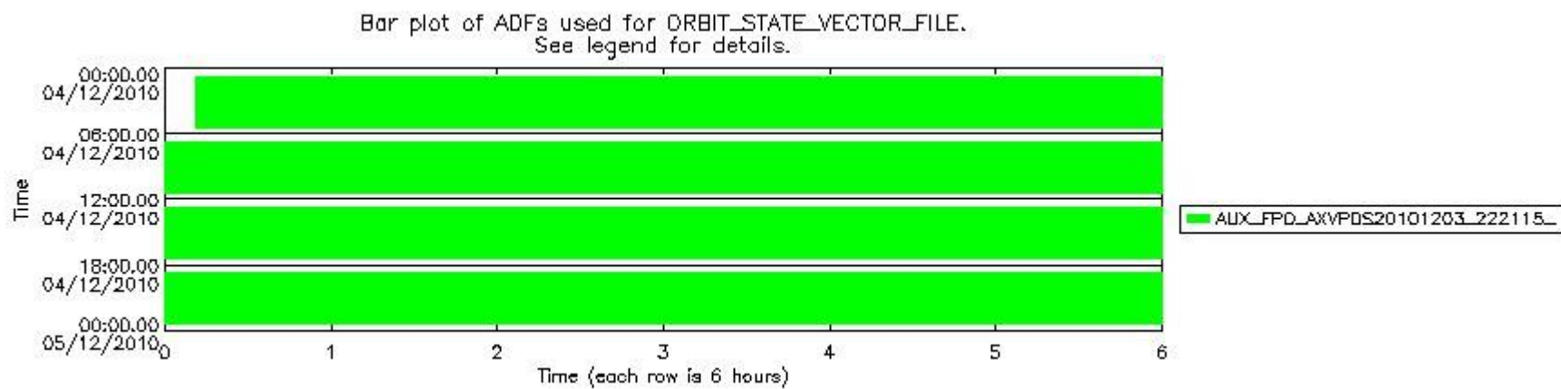
mipas_daily_report_level0_KSPT_L0_4504_N_20101204_13.PNG
