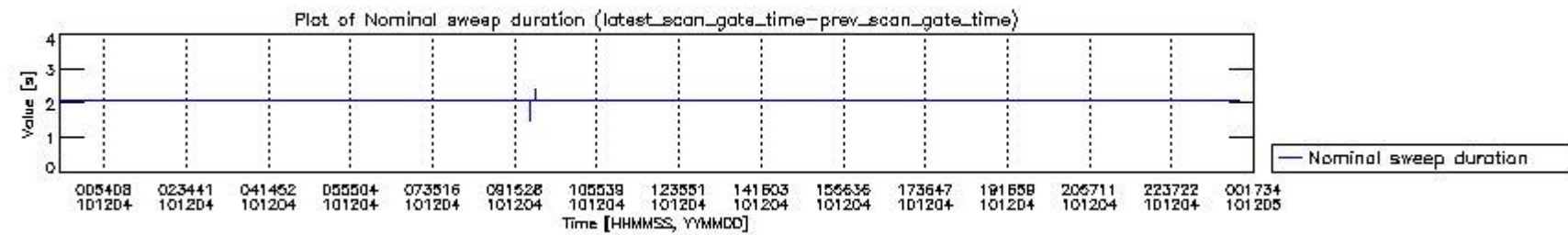
mipas_daily_report_level0_KSPT_L0_4504_N_20101204_4.PNG
