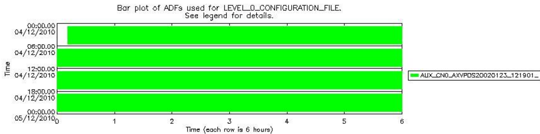
mipas_daily_report_level0_KSPT_L0_4504_N_20101204_12.PNG
