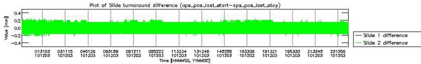
mipas_daily_report_level0_KSPT_L0_4504_N_20101203_5.PNG
