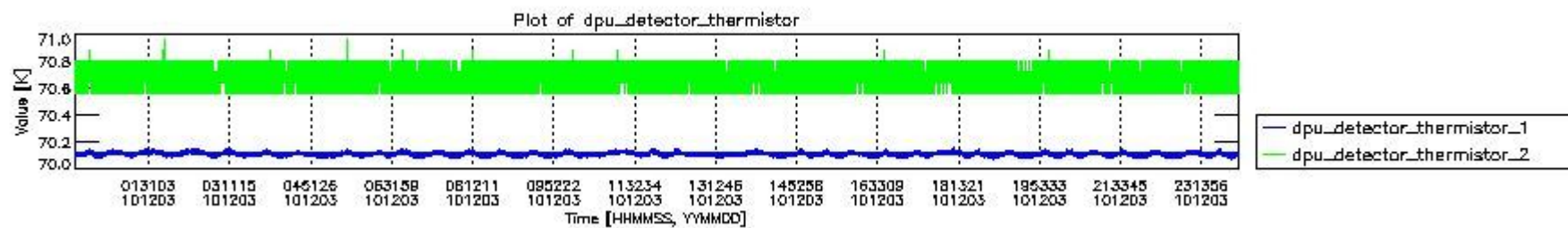
mipas_daily_report_level0_KSPT_L0_4504_N_20101203_3.PNG
