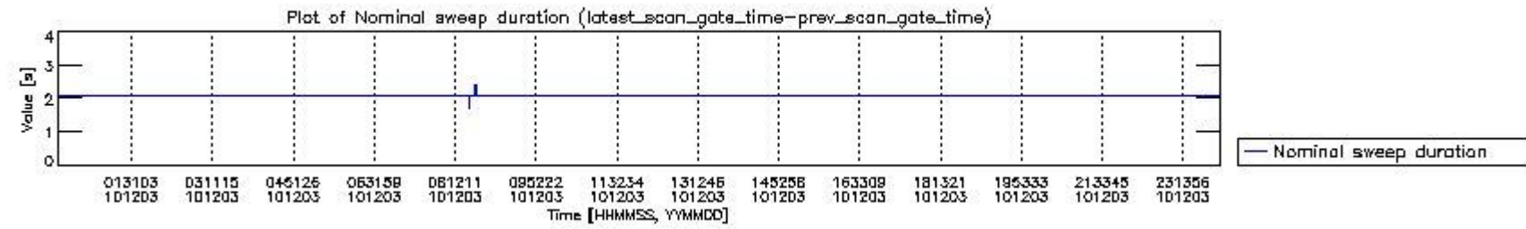
mipas_daily_report_level0_KSPT_L0_4504_N_20101203_4.PNG
