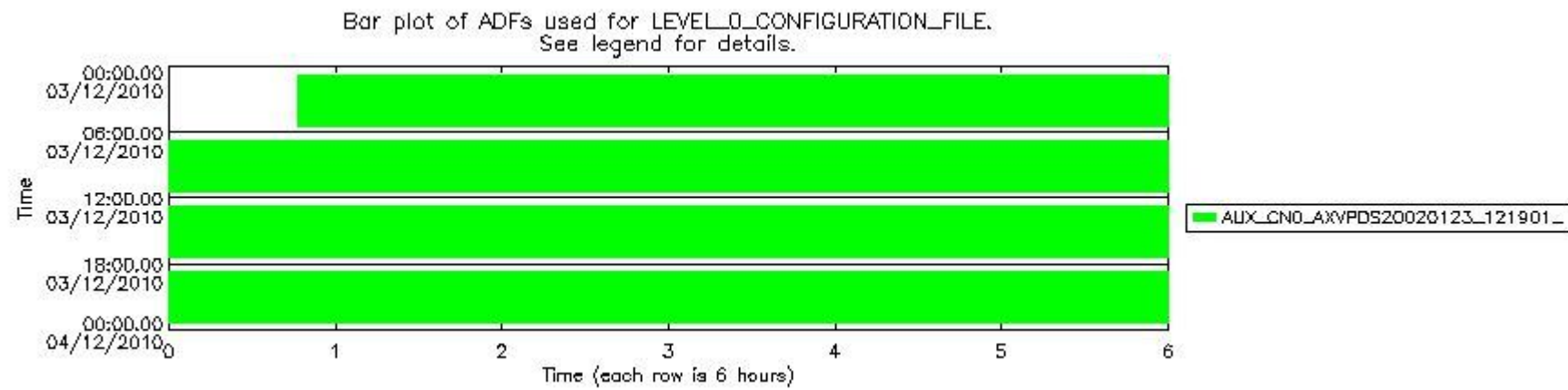
mipas_daily_report_level0_KSPT_L0_4504_N_20101203_12.PNG
