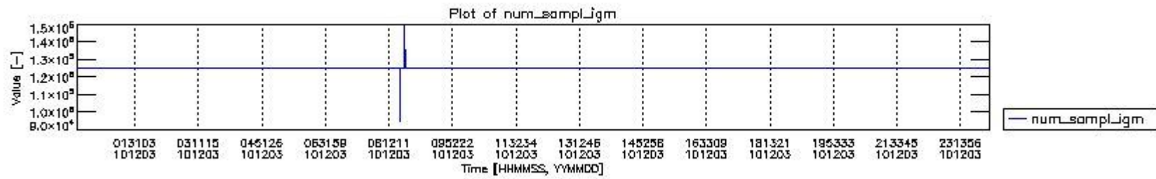
mipas_daily_report_level0_KSPT_L0_4504_N_20101203_0.PNG
