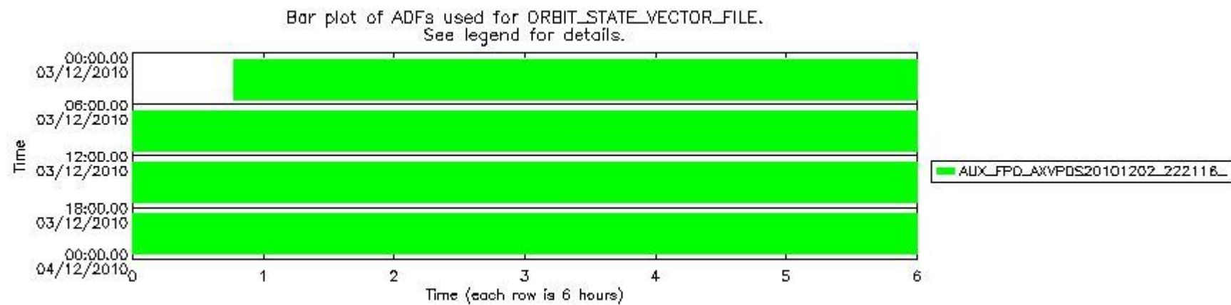
mipas_daily_report_level0_KSPT_L0_4504_N_20101203_13.PNG
