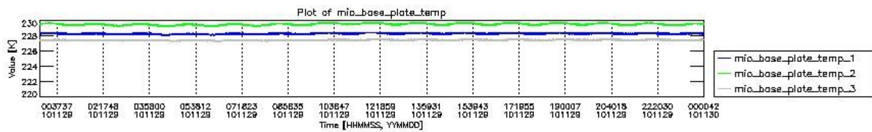
mipas_daily_report_level0_KSPT_L0_4504_N_20101129_1.PNG
