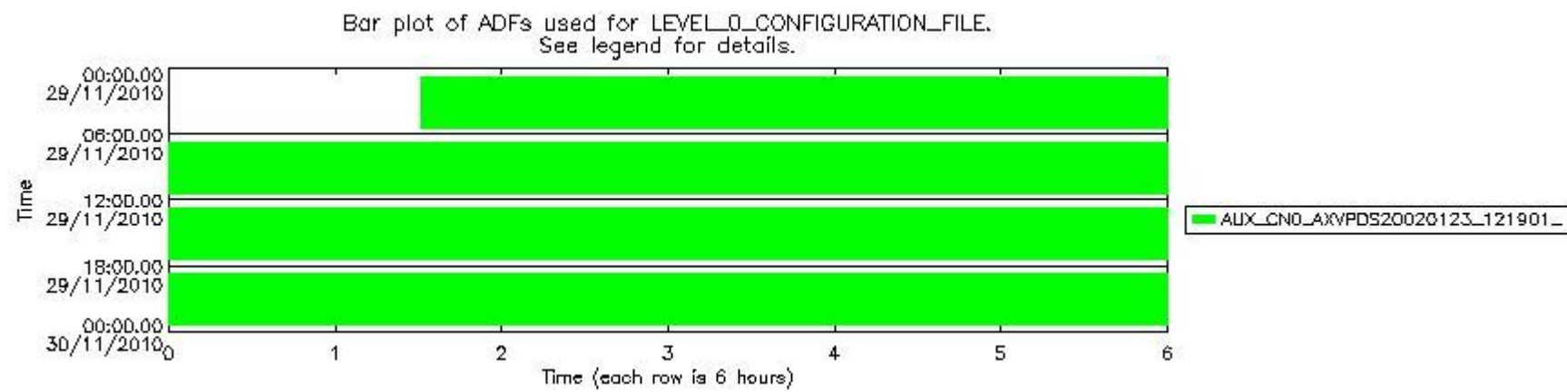
mipas_daily_report_level0_KSPT_L0_4504_N_20101129_12.PNG
