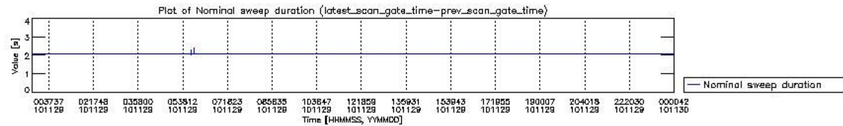
mipas_daily_report_level0_KSPT_L0_4504_N_20101129_4.PNG
