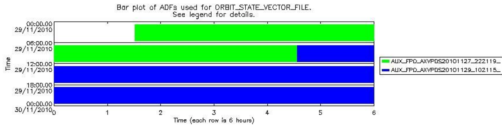
mipas_daily_report_level0_KSPT_L0_4504_N_20101129_13.PNG
