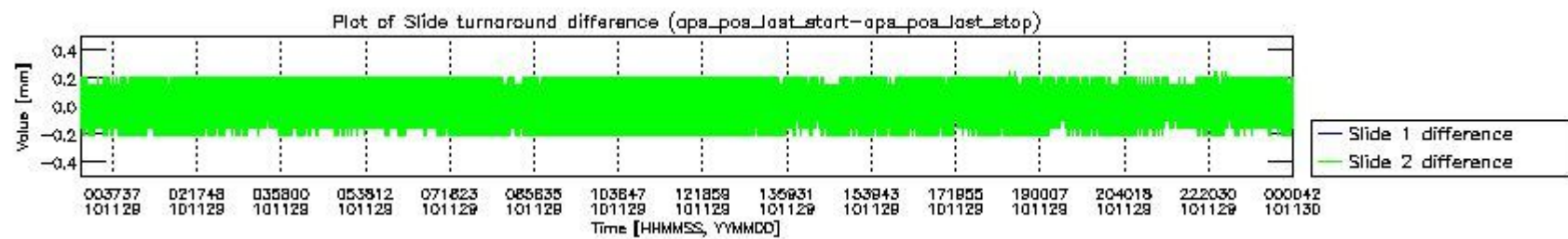
mipas_daily_report_level0_KSPT_L0_4504_N_20101129_5.PNG
