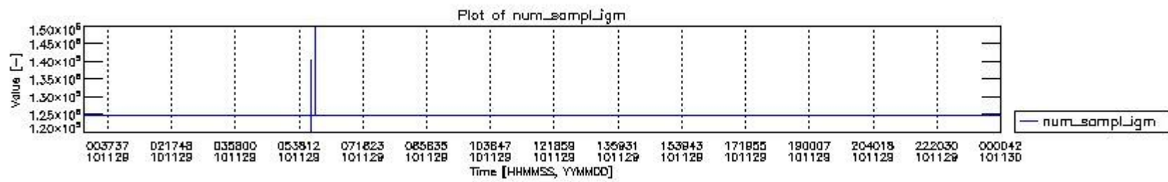
mipas_daily_report_level0_KSPT_L0_4504_N_20101129_0.PNG
