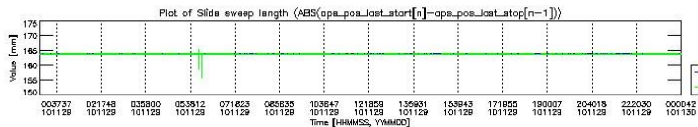
mipas_daily_report_level0_KSPT_L0_4504_N_20101129_7.PNG
