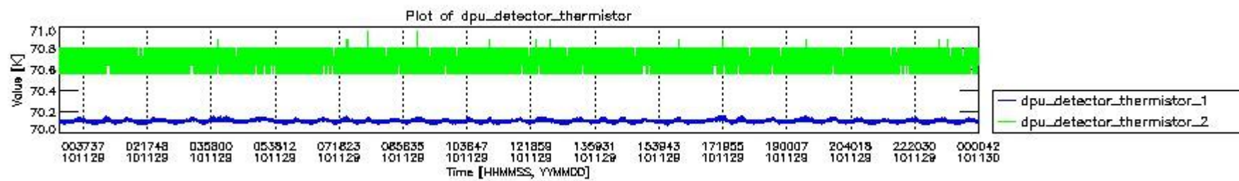
mipas_daily_report_level0_KSPT_L0_4504_N_20101129_3.PNG
