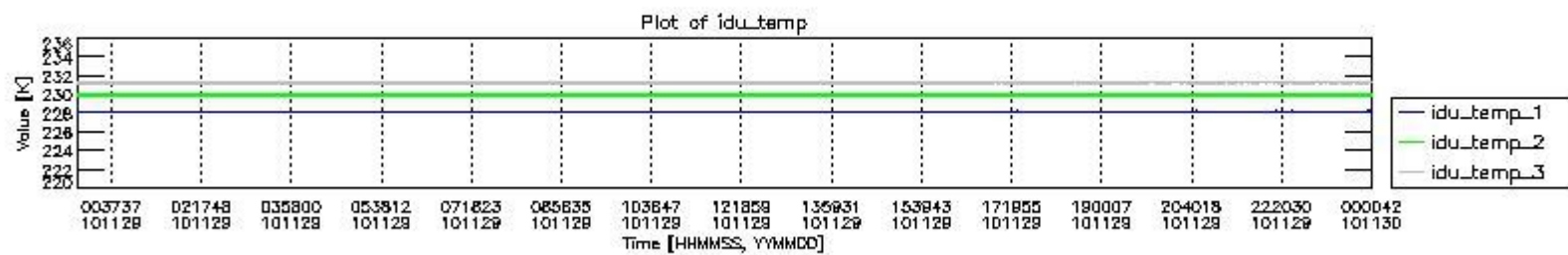
mipas_daily_report_level0_KSPT_L0_4504_N_20101129_2.PNG
