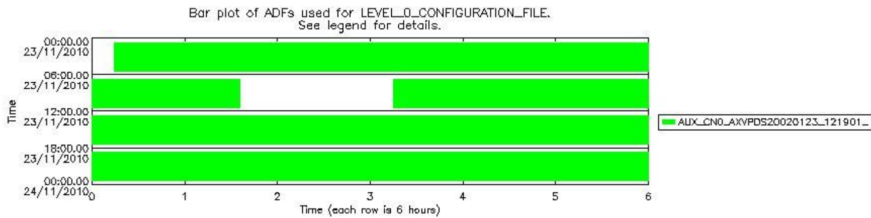
mipas_daily_report_level0_KSPT_L0_4504_N_20101123_12.PNG
