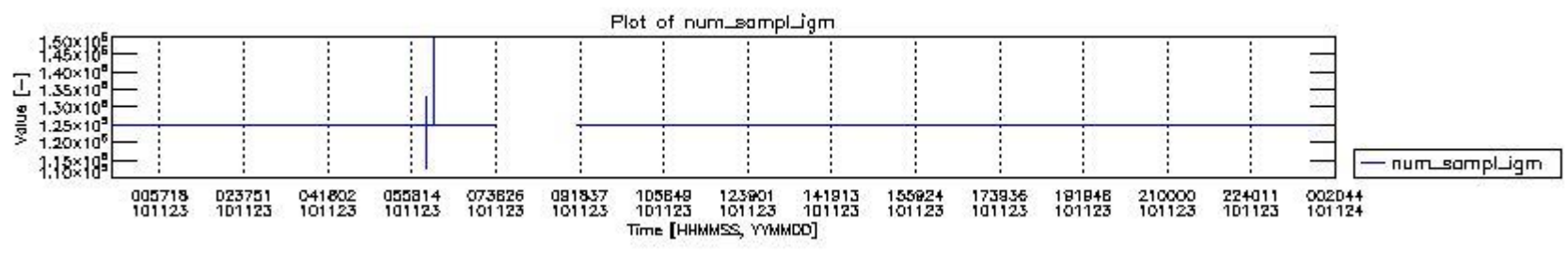
mipas_daily_report_level0_KSPT_L0_4504_N_20101123_0.PNG
