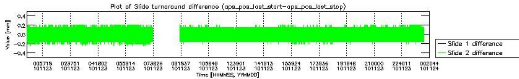
mipas_daily_report_level0_KSPT_L0_4504_N_20101123_5.PNG
