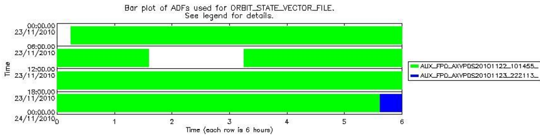
mipas_daily_report_level0_KSPT_L0_4504_N_20101123_13.PNG
