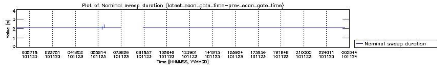
mipas_daily_report_level0_KSPT_L0_4504_N_20101123_4.PNG
