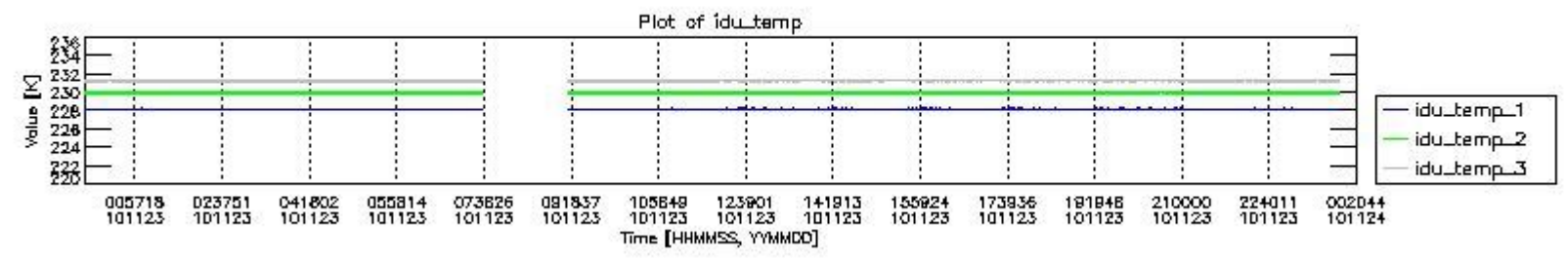
mipas_daily_report_level0_KSPT_L0_4504_N_20101123_2.PNG
