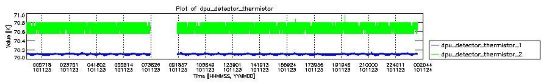
mipas_daily_report_level0_KSPT_L0_4504_N_20101123_3.PNG
