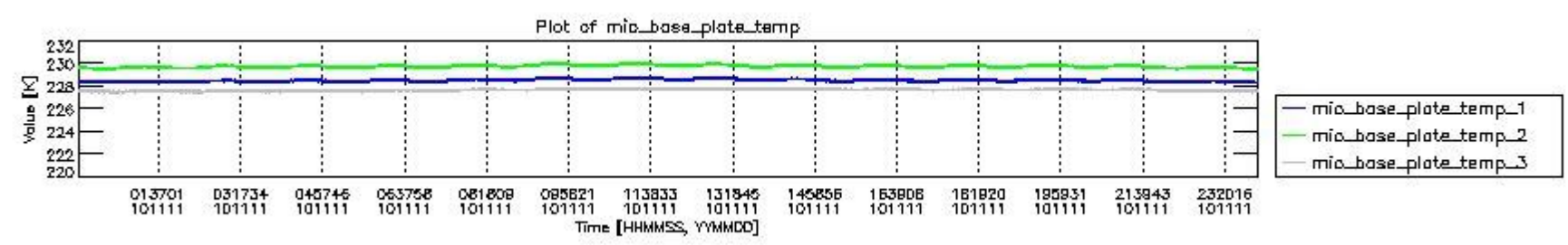
mipas_daily_report_level0_KSPT_L0_4504_N_20101111_1.PNG
