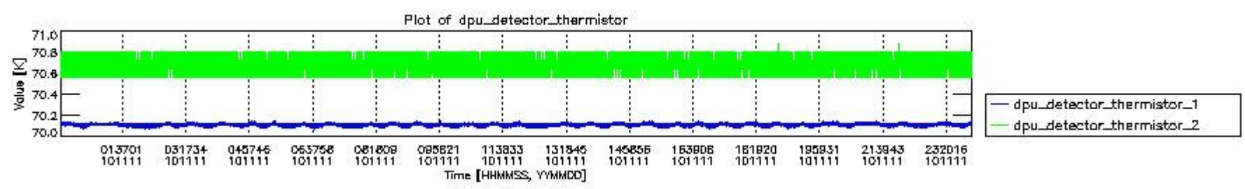
mipas_daily_report_level0_KSPT_L0_4504_N_20101111_3.PNG
