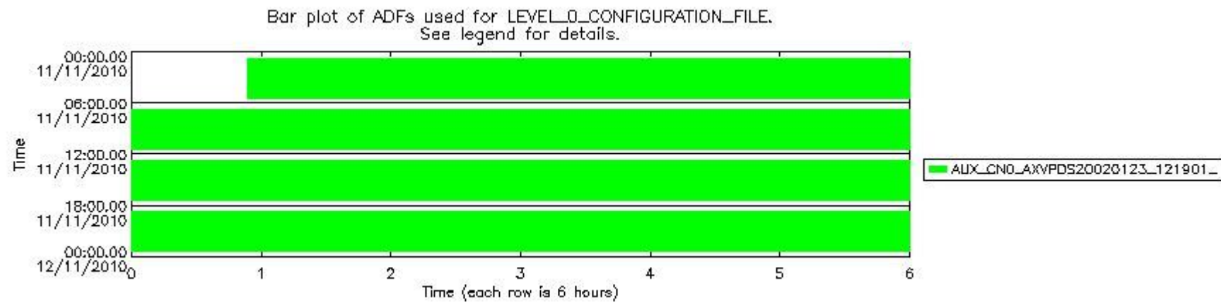
mipas_daily_report_level0_KSPT_L0_4504_N_20101111_12.PNG
