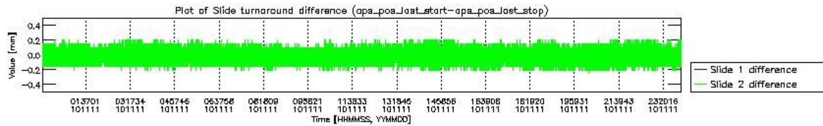
mipas_daily_report_level0_KSPT_L0_4504_N_20101111_5.PNG
