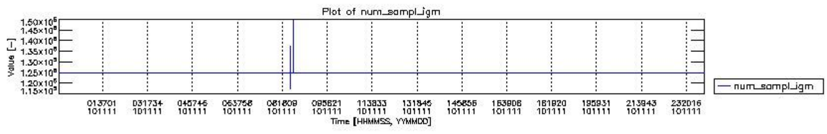
mipas_daily_report_level0_KSPT_L0_4504_N_20101111_0.PNG
