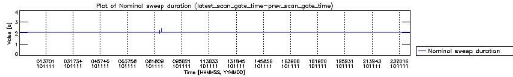
mipas_daily_report_level0_KSPT_L0_4504_N_20101111_4.PNG
