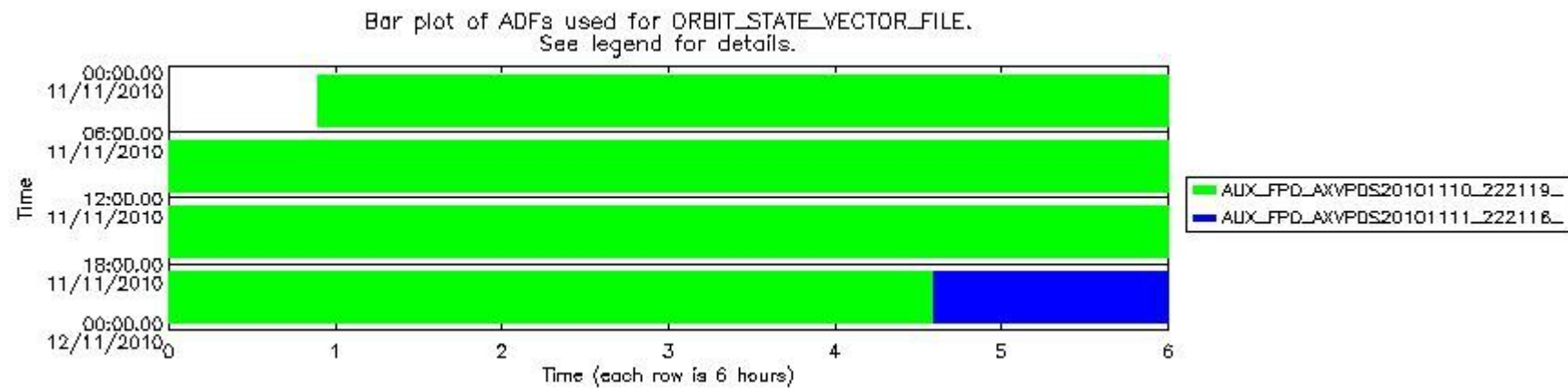
mipas_daily_report_level0_KSPT_L0_4504_N_20101111_13.PNG
